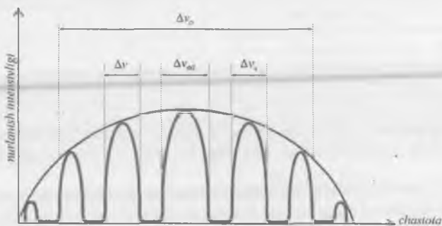
22.8-rasm. Optikaviy kvant generatorida nurlanish chizig'ini
