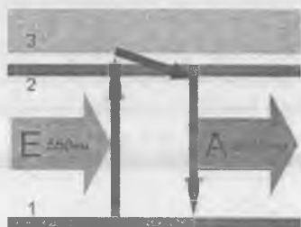
22.9-rasm. Yoqut lazerida xrom ionlari temlaridan ayrimlarining chizmasi.
