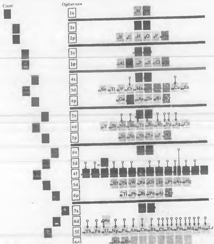
26.8-rasm. Kvant mexanik elementlarning davriy sistemasi.
