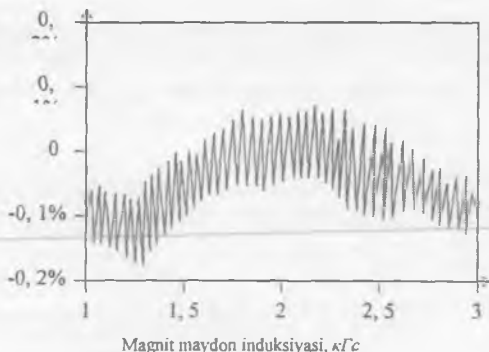
30.6-rasm Aaronov-Bom effektini oltin uzukcha bilan qilingan eksperiment grafiqi.
