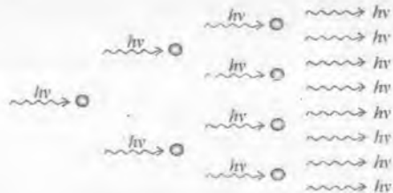
22.3-rasm. Foton lavinasining (uyumi) hosil bo'lishi
