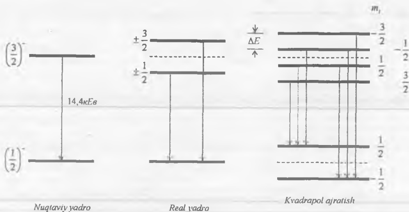
23.15-rasm. ^{57}\text{Fe} izotopida chiziqning o'ta nozik ajralishi.
