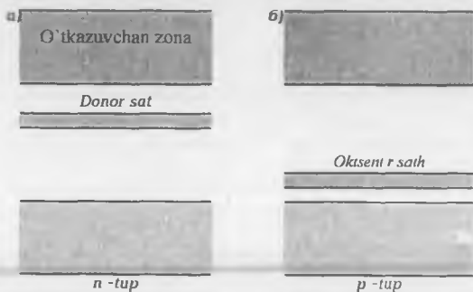
27.16-rasm. Aralashmaga yarimo'tkazgichlarda donor va akseptor energetik sathlar.
