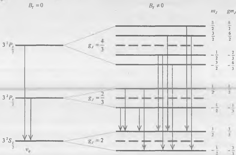
19.4-расм. Atom sathlarining kuchsiz magnit maydonda Zeyeman anomal ajralishi
