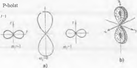
17.8-rasm. a) \theta - burchakka bog'liq bo'lgan p_\theta = |\theta_{1,0} \theta_{1,1}| va p_\theta = |\theta_{1,1} \theta_{1,-1}| holat uchun ehtimol zichligi; b) To'la ehtimol zichlik, burchak ehtimol zichligi p_\theta bilan radial ehtimol zichligi p_r ga ko'paytmasi.
