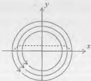
18.11-rasm Doiraviy elektromag-nit to'liqin paketida vaqt bo'yicha energiya oqimining sirkulatsiyasi.
