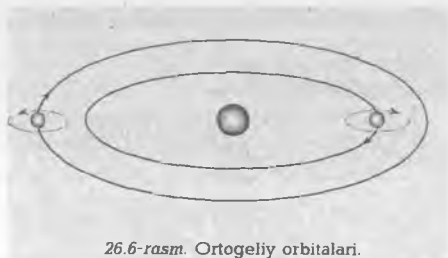
26.6-rasm. Ortogeliy orbitalari.
