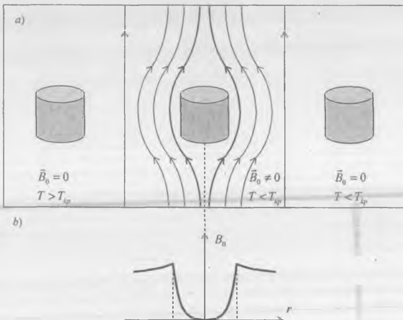
29.4- rasm a) Magnit maydonda o'ta o'tkazuvchan tsilindr b) \vec{B} magnit induksiyaning r ga bog'liqlik grafiqi.
