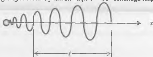
20.2-rasm. Yorug'lik impulsi yoki to'lqinlar sistemasini - sug.
