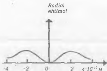
2p, uyg'ongan holatda elektronning radial ehtimol zichligi
