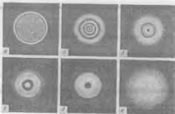
22.19-rasm. Doiraviy tirqishda Frenel difraksiyasi. \bar{z}_0 kattalik o'zgarmas, z esa a dan e gacha o'sib boradi.
