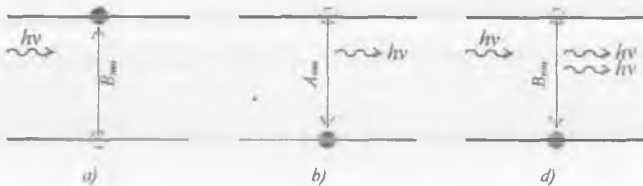
20.7-расм. Atomda pastdan yuqoriga ( n \rightarrow m )
