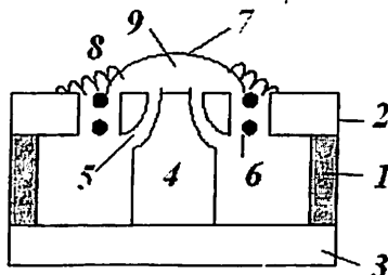
7.15–расм. Ғалтакли микрофон тузилиши.
