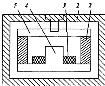
7.25–расм. Ларингофон тузилиши.
