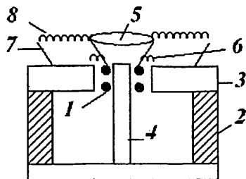
7.2–расм. Диффузорли динамик радиокарнай тузилмаси.
