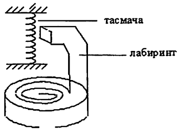
7.17–расм. Лабиринт.
