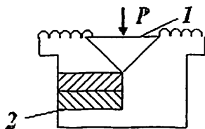
7.20–расм. Пьезоэлектрик микрофон тузилиши.
