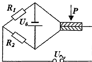
7.21–расм. Микрофоннинг электр уланиш схемаси.
