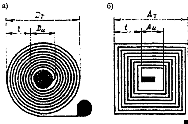
3.2-расм. Доиравий (а) ва квадрат (б) шаклдаги юпка пардали индуктивлик ғалтаги.
