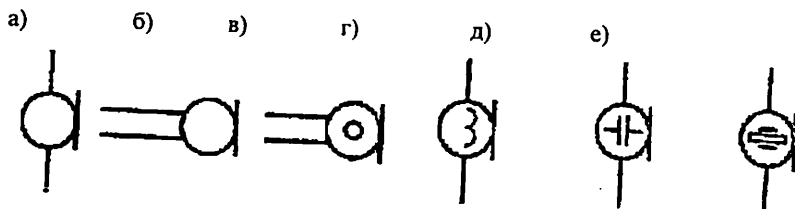
7.8–расм. Микрофонларнинг электр схемаларда шартли белгиланиши: умумий белгиланиши (а, б), углеродли (в), электродинамик (г), конденсаторли (д) ва пьезоэлектрик (е).
