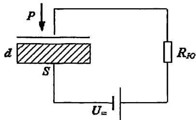
7.18–расм. Конденсаторли микрофон тузилиш схемаси.
