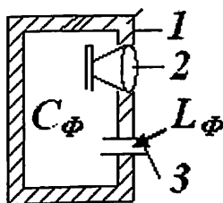
7.5–расм. Фазоинвертор.
