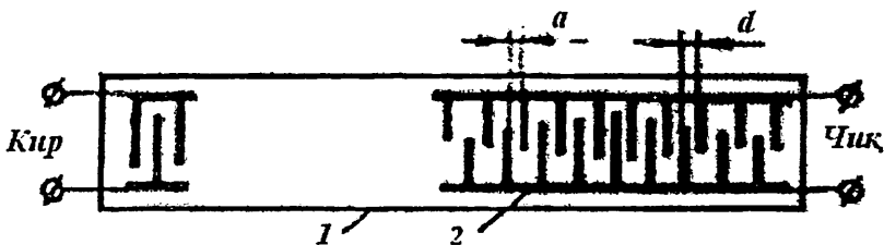
4.2–расм. САТдаги интеграл филтър: 1–пъезоэлектрик пластина; 2–тароксимон ўзгартиргич.
