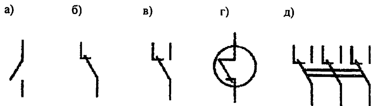
6.1–расм. Коммутация элементларининг схемаларда шартли белгиланиши: уловчи (а), узувчи (б), алмашлаб уловчи (в) контактлар, геркон (г) ва алмашлаб улагич (д).
