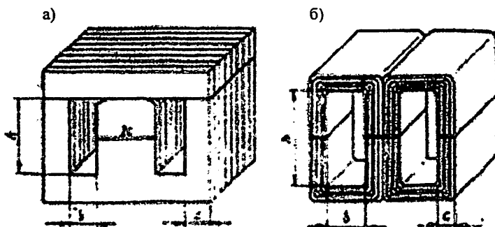
5.2–расм. Трансформаторларнинг зирхли ўзаклари: штампланган (а); лентали (б).
