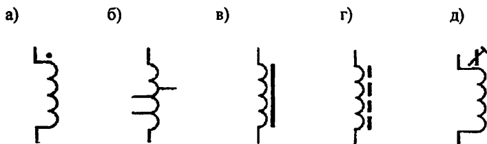
3.1–расм. Индуктивлик ғалтакларининг электр схемаларда шартли белгиланиши: дроссель (а), тармоқланган дроссель (б), магнит ўзакли (в), феррит ўзакли (г) ва созловчи ўзакли ғалтак (д) .
