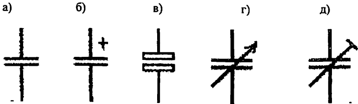
2.1–расм. Конденсаторларнинг электр схемаларда шартли белгиланиши: ўзгармас (а), кутли(б), кутбсиз (в), ўзгарувчан (г) ва созловчи (д).
