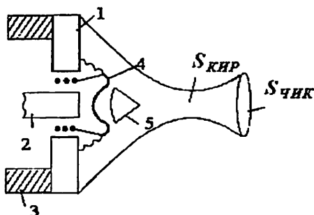
7.7 – Тор бўғизли рупорли радиокарнай.
