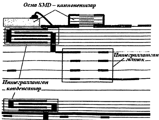
8.2–расм. LTCC асос қатламлари стейк намунаси.
