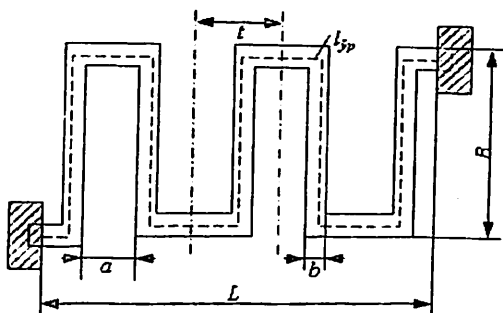
1.7–расм. “Меандр” туридаги юпқа парадали резистор геометрияси: l_{урт} ва b – резисторнинг ўртача узунлиги ва кенглиги; l , a , L ва B – меандрнинг қадами, звенолари орасидаги масофа, узунлиги ва кенглиги.
