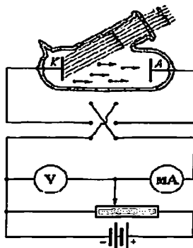
4.3– rasm. Fotoeffekt hodisasini o'rganuvchi qurilma
