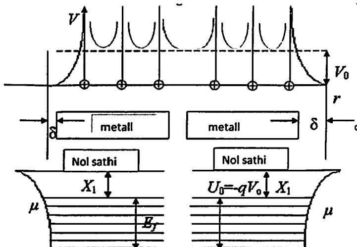
9.1 – rasm. Metall atomlarining energetik diagrammasi va ichki davriy potentsiali
