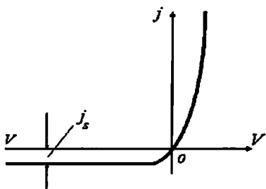
9.12 – rasm. Yarimo'tkazgich kontaktining volt – amper xarakteristikasi
