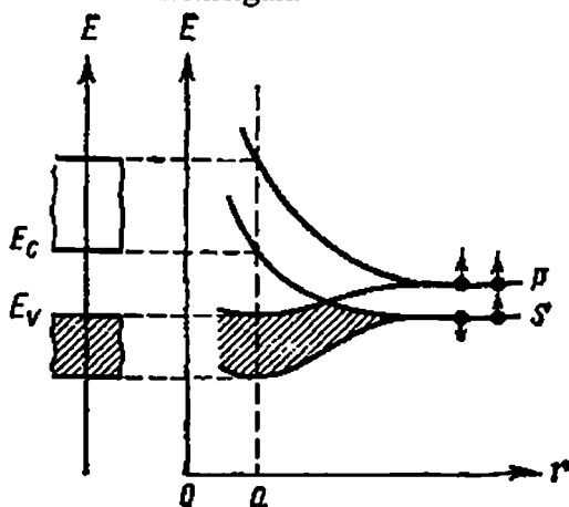
6.10 – rasm. Yarim o'tkazgichlarning energetik sohaları
