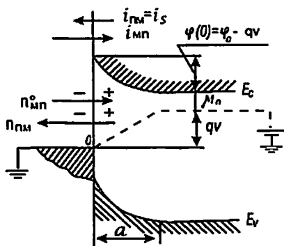
9.11 – rasm. M – yarimo'tkazgich kontaktiga to'g'ri yo'nalishda potentsiallar farqi qo'yilgan holat
