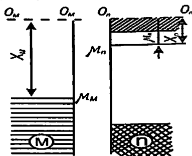
9.7 – rasm. Kontakt hosil bo'lguncha metall va yarimo'tkazgichning energetik diagrammalari
