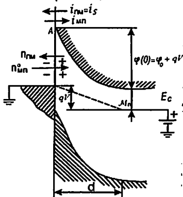
9.10 – rasm. Metall – yarimo'tkazgich kontaktiga teskari yo'nalishda tashqi potentsiallar farqi qo'yilishi
