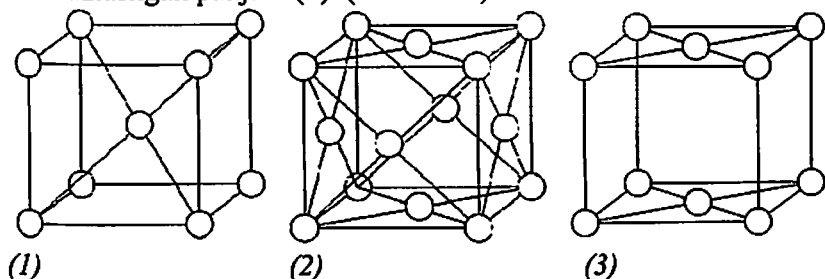
6.4 – rasm. Elementar yacheykalar turlari
