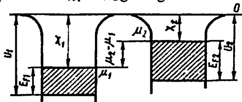
9.3– rasm. Ikkita ajratilgan metallning energetik diagrammalari
