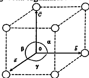
6.3 – rasm. Elementar yacheykaning asosiy parametrlari
