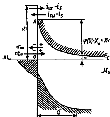
9.9 - rasm. Muvozanat holatdagi metall - yarimo'tkazgich kontakti
