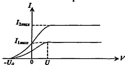
4.4 – rasm. Fotoeffektning volt – amper xarakteristikasi
