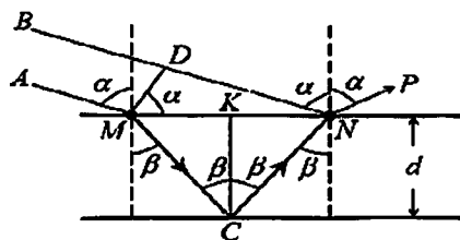
1.6-rasm. Yupqa tiniq plastinkadagi yorug'lik interferensiyasi
