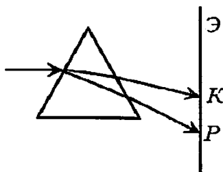
3.3 – rasm. Uchburchakli prizmadagi yorug'lik dispersiyasi
