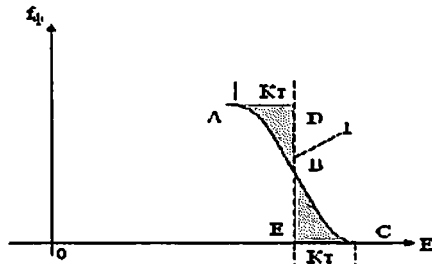
6.1.5 – rasm. Fermi –Dirak funksiyasini temperaturaga bog'liqligi
