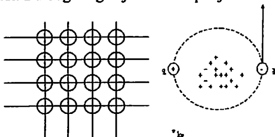
6.14 – rasm. O'taotkazish hodisasida Kuper juftlarini hosil bo'lishi
