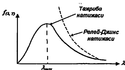
4.1-rasm. Nurlanish spektri.
