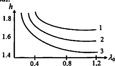
3.2 – rasm. Shisha(1), kvars(2) va flyuoritning(3) dispersiyasi
