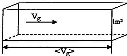
6.12 – rasm. \langle \vartheta_x \rangle harakat tezlikli elektronlar oqimi
