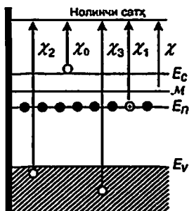
9.2– rasm. Elektron tipli yarim o'tkazgichda elektronlarni vakuumga chiqish yo'llari
