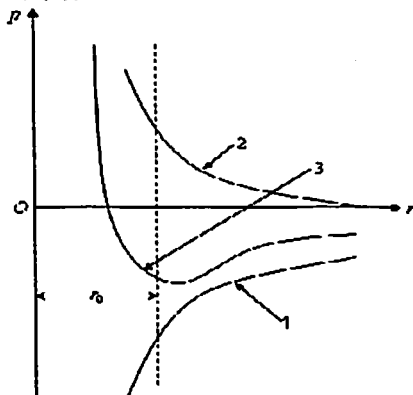
6.1 – rasm. Atomlar orasidagi bog'lanish kuchlari
