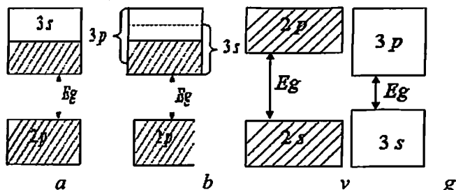
6.11 – rasm. Qattiq jismlar energetik sohasini elektronlar egallash turlari
