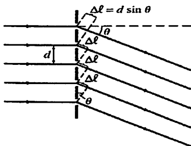
2.3-rasm. Difraksiyon panjara
