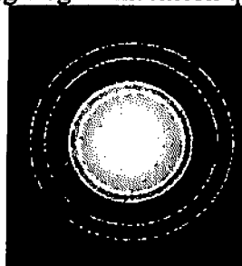
4.1.1-rasm. Elektronlar difraksiyasi
