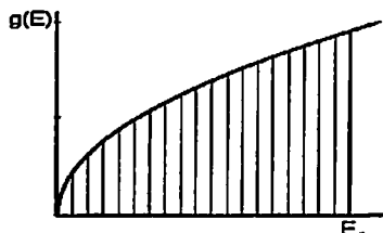
6.15 – rasm. Normal holatdagi metallarda holatlar zichligining energiyaga bog'liqligi
