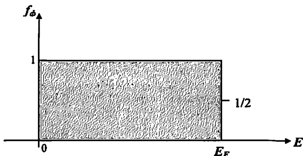
6.1.4 – rasm. Fermi – Dirak taqsimot funksiyasining energiyaga bog'liqlik grafigi
