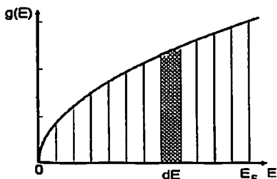
6.1.2 – rasm. Holatlar zichligini energiyaga bog'liqligi
