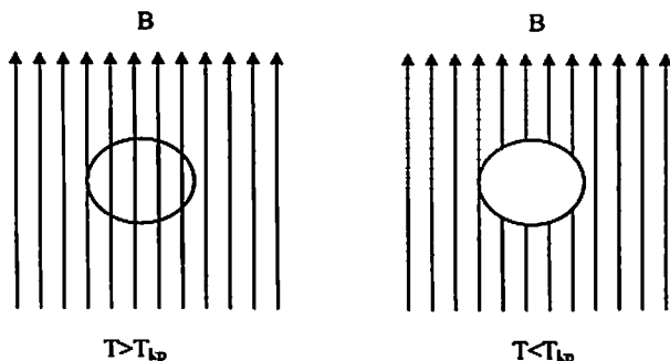
6.13 - rasm. O'tao'tkazish hodisasida qattiq jismlarda magnet maydonini siqib chiqarish
