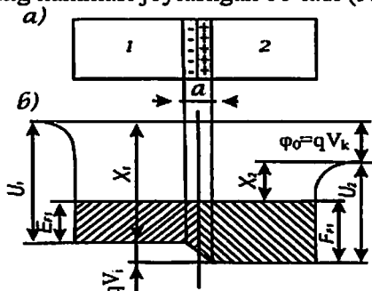
9.5 - rasm. Ikkita metall tutashganda ichki kontakt potentsiallar farqi hosil bo'lishi
