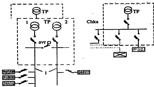
5.6-rasm. I toifali avariya yoritishni ta'minlash sxemasi.
