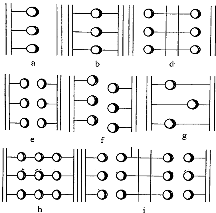
6.1- rasm. Yoritgichlarning joylashish sxemasi
