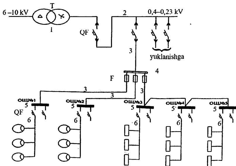
5.4-rasm. Elektr yoritish tarmog'i.
