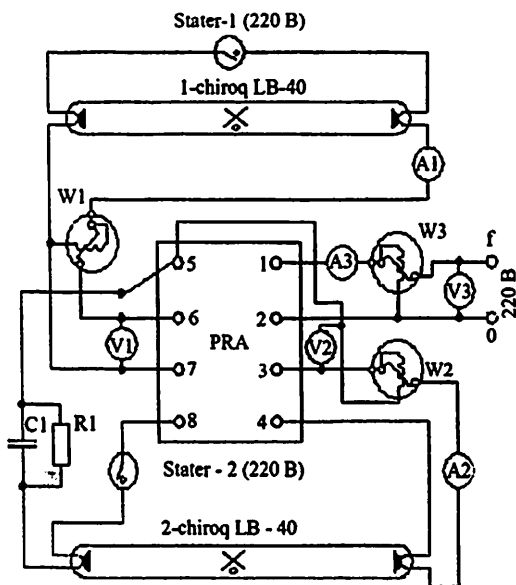
3.7-rasm. Ikki yoritgichli bir fazali ta'minotga ulangan lyuminessent chiroqlarning (2x20 W) antistroboskopik ulanish sxemasi.
