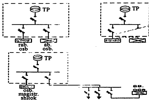
5.5-rasm. Avariya yoritishning bir transformatorli ta'minoti.
