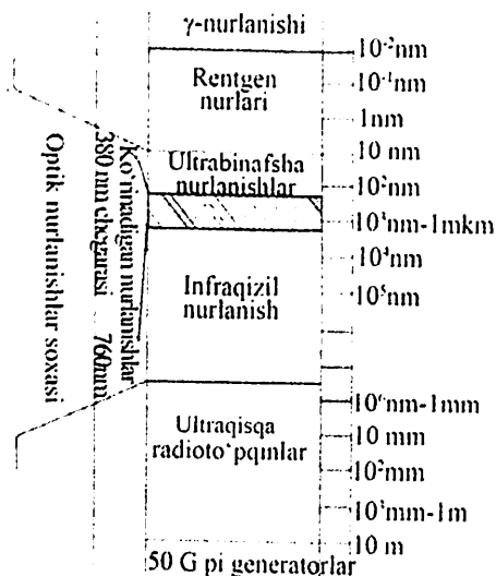
1.1-rasm. Elektromagnit nurlanishlar spektri
