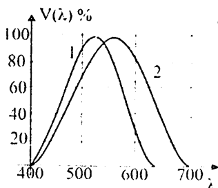
1.6-rasm. Nurlanishning nisbiy spektral yorug'lik samaradorligini egri chiziqdari. 1 – tungi ko'rish qobiliyati uchun 2 – kunduzgi ko'rish qobiliyati uchun .
