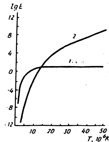
7.17-расм. Водород (1) ва углерод-азот (2) цикларида энергия чиқиш тезлиги.
