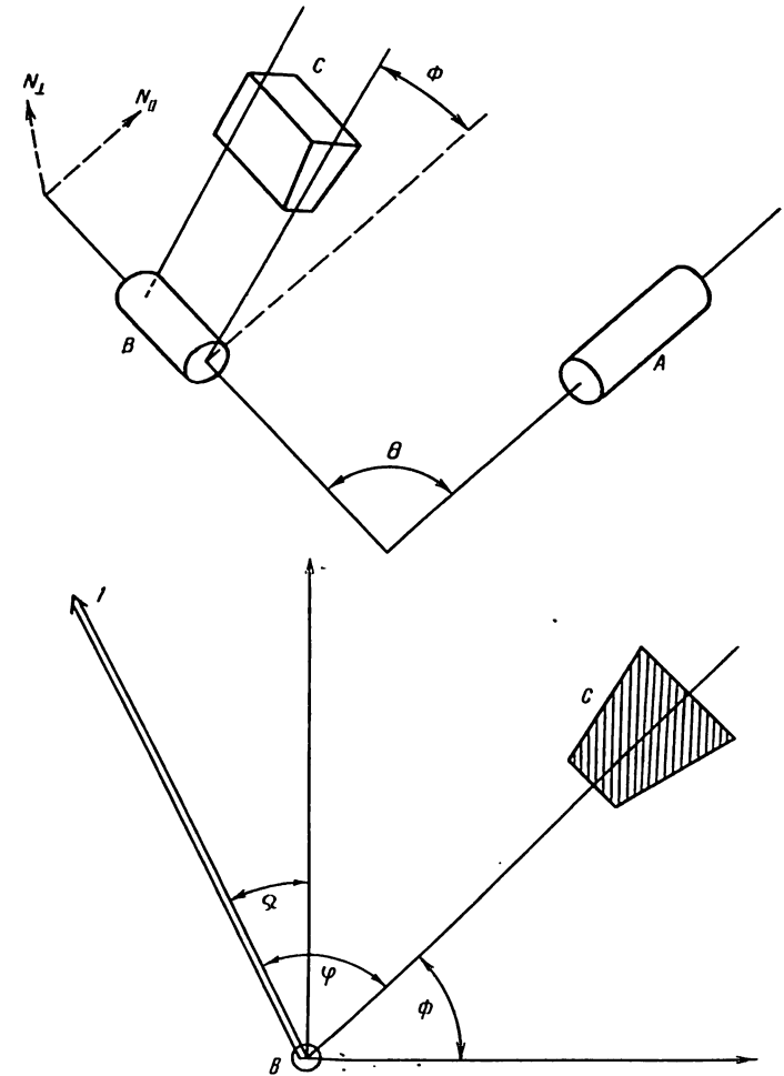
4. 8- расм. \gamma_1 — \gamma_2 — каскаднинг йўналиши (а) ва кутбланиш корреляцияларини (б) ўлчаш қурилмаларини: а) А, В, С — сцинтилляция счётчиклари; б) В—С поляри-метрли схема, 1 кутбланиш векторининг йўналиши, 2 \gamma_1 ва \gamma_2 нурланиш текислигига тик йўналиш.
