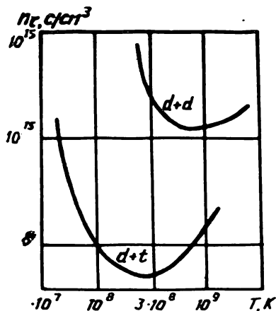
7. 10- расм. Дейтерий — три-тий ва дейтерий — дейтерий термоядро реакциялари учун ушлаб туриш параметрининг температурага боғлиқлиги.
