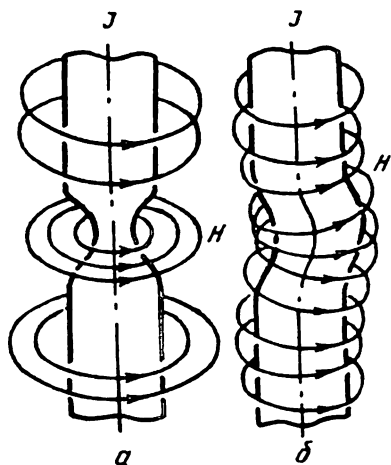
7. 13- расм. Плазма шнурдаги оддий «бўғиб кўйиш» (а) ва «эгилтиш» (б) типдаги бекарорликлар. Шнур ўқи бўйича стрелка ток йўналишини, айланалардаги стрелка эса, токнинг плазма ҳосил қилган магнит майдонининг йўналишини кўрсатади.
