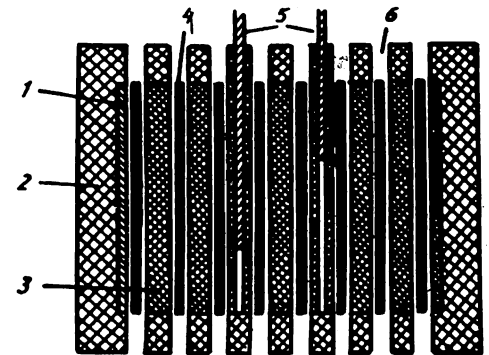
7.8-расм. Иссиқлик нейтронларда ишлайдиган ядро реактори схемаси:
