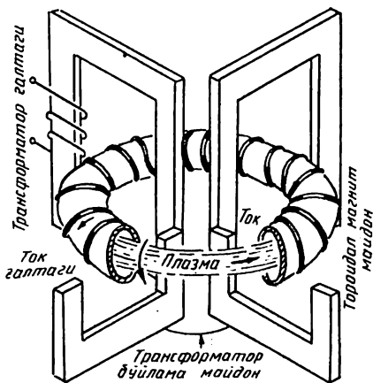
7. 14- расм. Плазмали тор ёки стелларатор типдаги қурилма.
