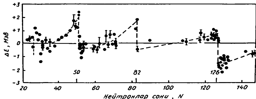
1. 14-расм. Нейтроннинг ажратиш энергиясининг тажрибада аниқланган ва боғланиш энергияси формуласи асосида ҳисобланган кийматлари орасидаги фарк \Delta E_n^{a,jp} нинг нейтронлар сонига қараб ўзгариши.
