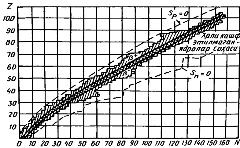
1. 3-расм. Сегренинг нейтрон-протон диаграммаси.
