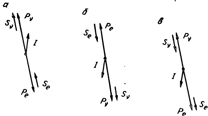
3. 16- расм. Ядро спини ва импульслари, электрон ва антинейтрино спинлари ўзаро йўналишларининг схемалари.
