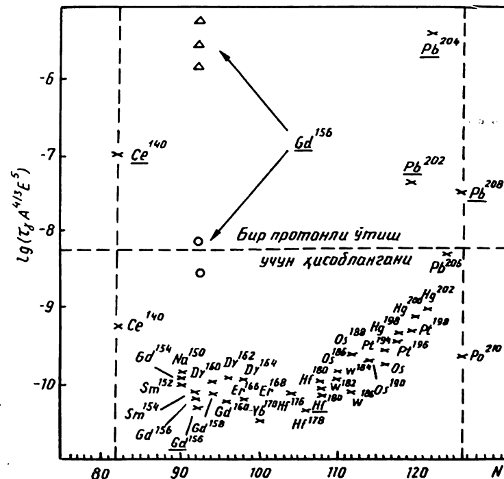
6. 22- расм. E2 - ўтишлар учун келтирилган яшаш вақтларининг N нейтронлар сонига боғлиқлиги. Назарий пункт чизиклар бир протонли ўтишлар учун ҳисобланган.
