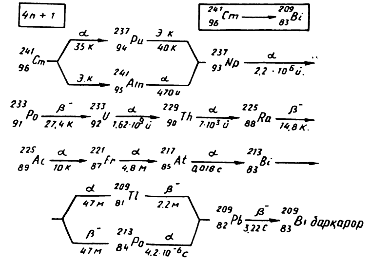
2. 1- б расм. Нептуний радиоактив онласи.
