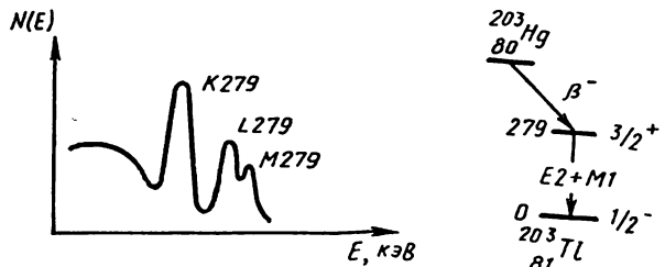
4. 14- расм. ^{203}\text{Hg} изотопининг узлуксиз \beta - спектри ва унинг устига тушган ички K , L , M конверсия электронларининг мос спектри чизиклари кўшилган \beta - спектрининг кўриниши (кэВ).
