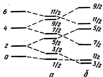
6. 17- расм. Баъзи тоқ ядроларнинг мумкин бўлган айланма ҳолатларининг ҳисобланган спектрлари: а) ташқи нуклон ўзак билан кучсиз боғланган; б) ташқи нуклон ўзак билан кучли боғланган.
