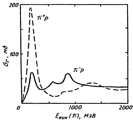
8. 9- расм. Пионларнинг протонларда сочилиш тўла кесимининг кинетик энергияга боғлиқлиги. Мусбат пионларнинг сочилиш кесими манфий зарядли пионларнинг сочилиш кесимига нисбатан деярли уч баробар катта.
