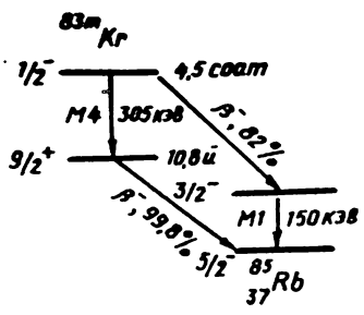
4. 15- расм. ^{85}\text{Kr} изомер 4,5 соатли ва 10,8 йиллик сатхларининг парчаланиши (кэВ).
