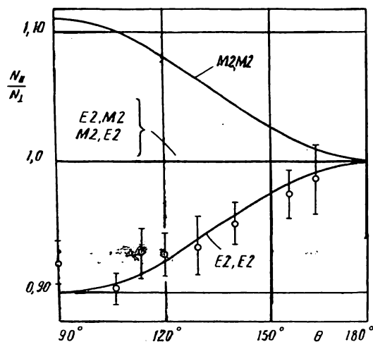
4. 9- расм. ^{46}\text{Ti} ядросида \gamma\gamma — йўналишлар ва қутбланиш корреляциялари. Экспериментал нукталар гамма ўтишлари мультиполликларини кўрсатади.
