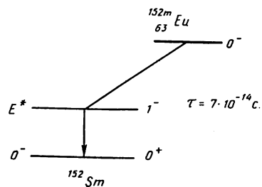
4. 13- расм. Европий-152 изомерининг парчаланиш схемасининг бир қисми.
