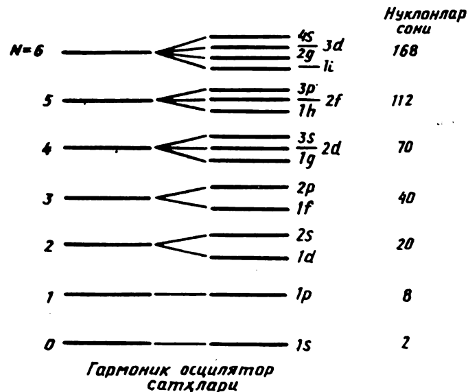
6.7- расм. Осциллятор қобиклари. Чапда гармоник осцилляторнинг энергия сатҳлари, ўнгда осциллятор потенциалнинг кўринишини ўзгартириш йўли билан турланиши бекор қилинган энергиялар сатҳлари. Чуқурни берилган қобиккача тўлдирадиган нуклонлар тўла сони кўрсатилган.
