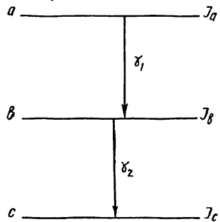
4. 4- расм. Каскадли \gamma - \gamma ўтишлар.
