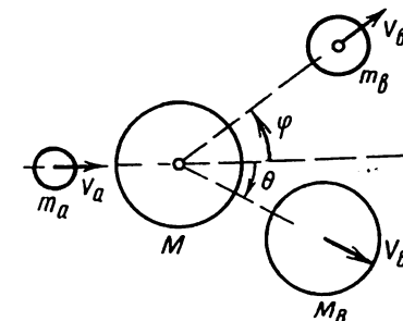
5. 1- расм. a + A \rightarrow B + b кўринишидаги ядро реакциясининг лаборатория системасидаги схематик тасвири.
