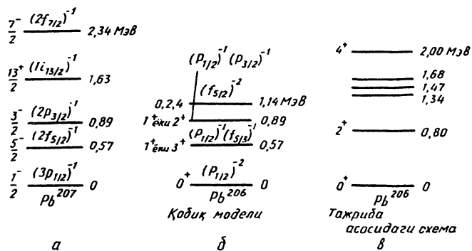
6. 10- расм. ^{206}\text{Pb} ва ^{207}\text{Pb} ядроларининг сатҳлари схемаси: а) ^{207}\text{Pb} қобик моделига асосан; б) ^{206}\text{Pb} ҳисобланган, яъни қутилган сатҳлар кетма-кетлиги; в) кузатилган экспериментал сатҳлар схемаси.
