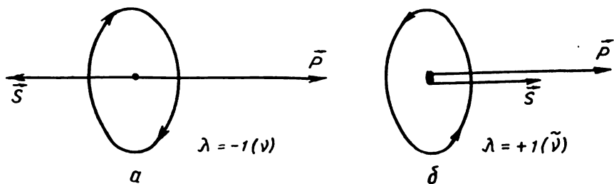
3. 11-расм. Нейтрино ва антинейтрино ҳамма вақт кутбланган: (а) нейтринонинг спини ҳаракат йўналиши (импульс)га тескари, (б) антинейтринонинг спини эса, импульс йўналиш бўйича бўлади.
