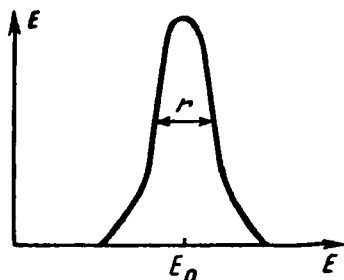
1. 17- расм. Сатх кенглигини кўрсатувчи эгри чизик.
