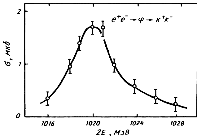
8.7-расм. Ўта катта энергия ( 2E ) ли электрон ва позитрон тўқнашиши натижасидаги e^+e^- \rightarrow K^+K^- жараённинг эффектив кесими.
