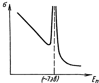
5. 7- расм. Нейтроннинг уран-238 ядросида ютилиш кесимининг нейтронлар энергиясига резонанс боғлиқлиги.
