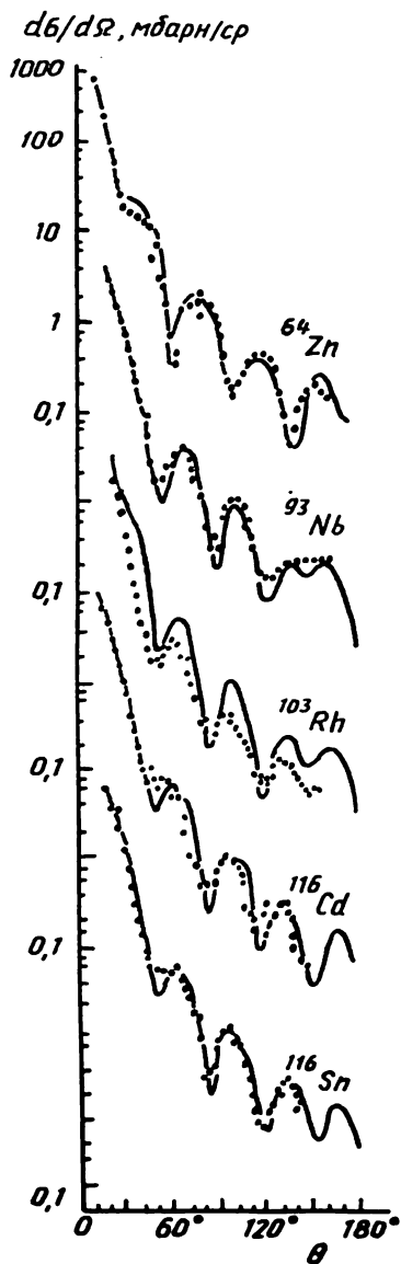
6. 20-расм. Протонларнинг ядроларда эластик сочилиш кесимининг бурчакка боғлиқлиги ( E_p = 22 МэВ).
