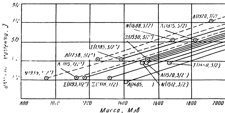
8. 20- расм. Барионларнинг Редже траекториялари.
