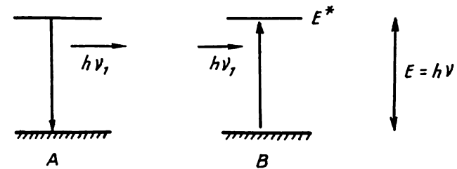
4. 10- расм. A^* ядронинг \gamma -квантлари билан худди ўзига ўхшаган B ядрони асосий ҳолатдан кўзғалган ҳолатига кўтариши. Аммо тепкига энергиянинг бир қисми йўқолганлиги туфайли B ядро E^* ҳолатга кўтарилмайди.
