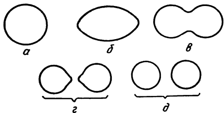
7. 1- расм. Нейтрон келиб ютилгандан сўнг ядро-томчининг бўлиниш кетма-кетлиги.
