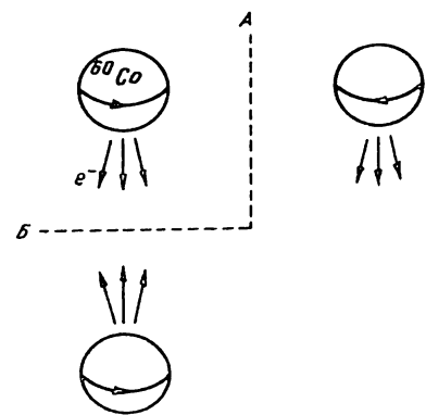
3. 14- расм. ^{60}\text{Co} -нинг парчаланишида жуфтликнинг сақланмаслиги.
