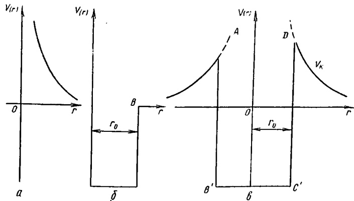
1.19-расм. Ядро билан мусбат зарядли зарра ўзаро таъсир энергиясининг масофага кўра ўзгариши: а) зарра ва ядронинг кулон итаришиши; б) ядро кучларини ифодаловчи тўғри бурчакли потенциал ўра; в) ядро ва кулон ўзаро таъсирларининг қўшилишидан ҳосил бўлган потенциал ўра.
