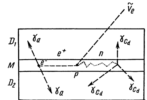
3. 10- расм. Анти-нейтринони қайд қилиш қурилмаси.
