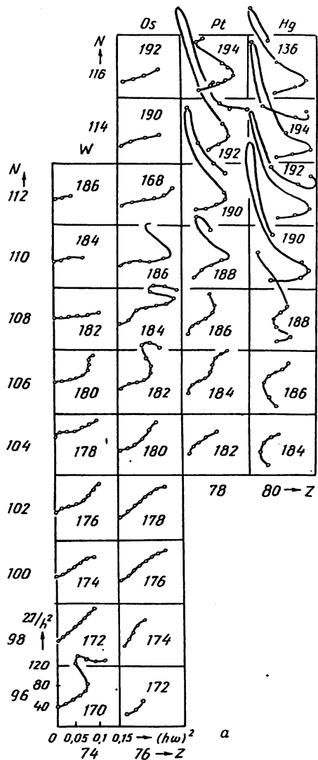
6. 24- а, б расм. Нейтрон сонлари 96 \div 116 ва 88 \div 96 протонлар сони 74 \div 80 ва 62 \div 72 гача бўлган ядроларнинг инерция моментларини ядро айланишининг бурчак тезлиги квадратига боғлиқлиги. Қийшиқ чизиқлар устидаги нукталар ираст ҳолатларнинг спин қийматлари (системалаштирган Р. Б. Бекжонов).
