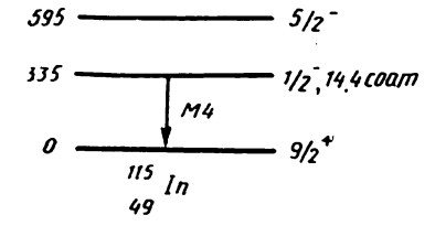
4.17- расм. ^{115}\text{In} изотопининг изомер сатҳининг парчаланиши (кэВ).
