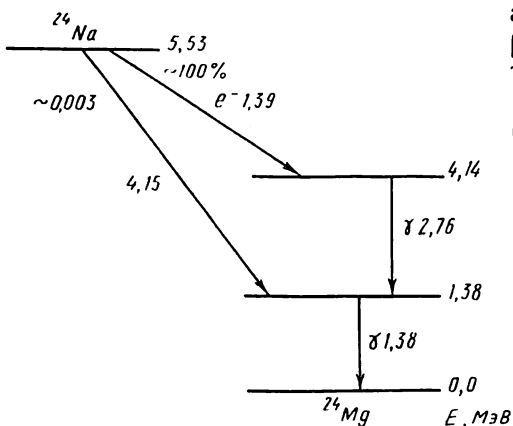
3.6-расм. {}^{24}\text{Na} — нинг \beta -парчаланиш схемаси.
