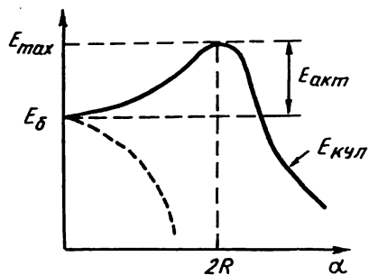
7. 2- расм. Ядро бўлиниш энергиясининг деформацияланишга боғликлги. Туташ чизик Z^2/A < 46,6 ва узлуклиги Z^2/A > 46,6 бўлган ядролар учун.
