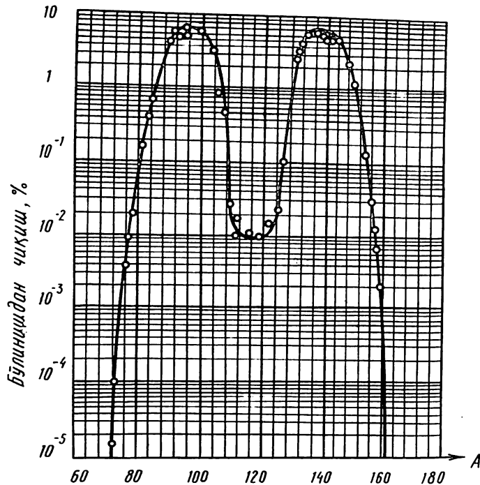
7. 6- расм. Уран-235 ядролари бўлиниш парчаларининг масса A бўйича тақсимоли. Вертикал ўқида парчаларнинг чиқиш эҳтимоллиги кўйилган.
