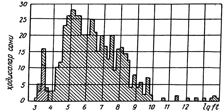
3. 5-расм. ft — микдор қийматларини гистограммаси, штрихланган соҳалар кўзгу ўтишларига тегишли.
