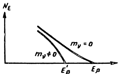
3. 12- расм. Юқори чегарада \beta -спектрнинг шакли.
