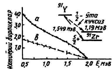
3.8-расм. Такикланган ўтишлар учун Ферми графиги: а) эксперимент натижалари; б) ўша графигнинг a_n кўпайтма ёрдамида тўғриланиши.
