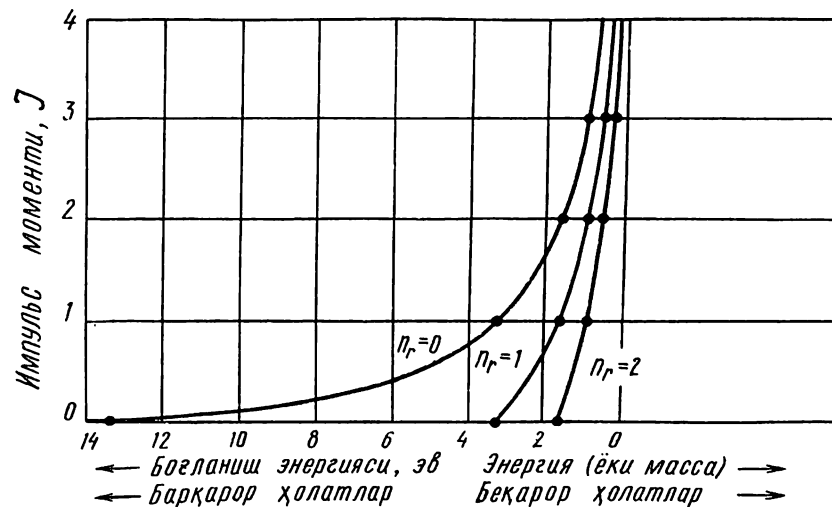
8. 19- расм. Водород атоми учун Редже траекториялари.
