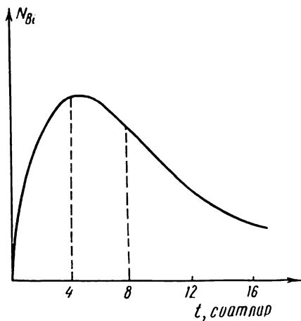
2. 2- расм. Кўрғошин- 212 нинг бета-парчаланишида висмут- 212 ядроларининг йиғилиши.
