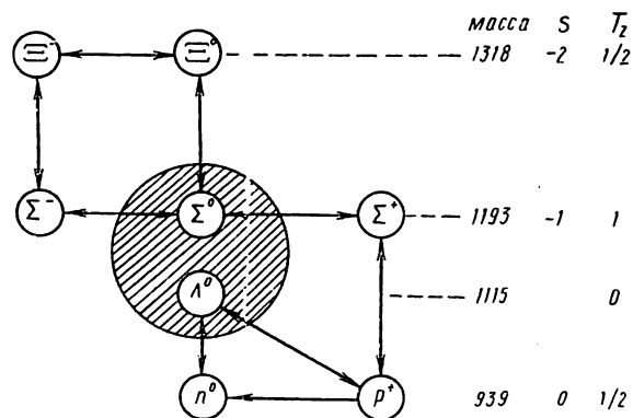
8. 17- расм. Нуклон ва гиперонлардан иборат супермультитиплетбарион октети (саккизлиги). Бу октетга N -дуплети, \Lambda^0 -синглети, \Xi -дуплети ва \Sigma -триплетги киради.
