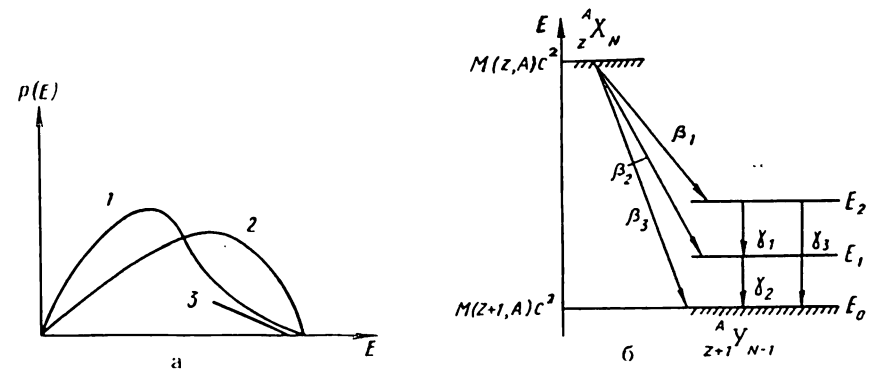
3. 4- расм. \beta^- -спектр шаклининг нейтрино массасига боғлиқлигини мос равишда ўзгарishi: 1) — m_\nu = 0 , 2) — m_\nu = m_e 3) — m_\nu \neq 0 ҳоллар учун.
