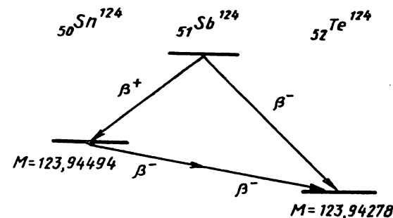
3. 13- расм. {}^{124}\text{Sn} ядросининг кўш \beta - парчаланиши ( 2\beta^- ) мумкин эканлигини кўрсатувчи диаграмма. Атом массалари фарқидан \beta - парчаланишнинг кинетик энергияси \sim 2 МэВ эканлиги кўриниб турибди. {}^{124}\text{Sb} нинг массаси {}^{124}\text{Te} нинг массасидан 2,9 МэВ га катта.
