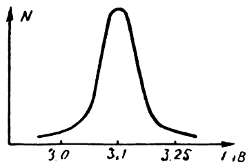
8. 11-расм. Нишондан e^+e^- жуфтининг чиқиш эҳтимоллигининг бомбардимон қилувчи протонларнинг энергиясига боғлиқлиги.
