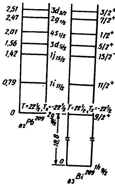
1.18- расм. ^{209}\text{Bi} ва ^{209}\text{Pb} ядроларининг T = 22\frac{1}{2} ли изотопик мультиплетга кирувчи энергия сатҳлари (МэВ).
