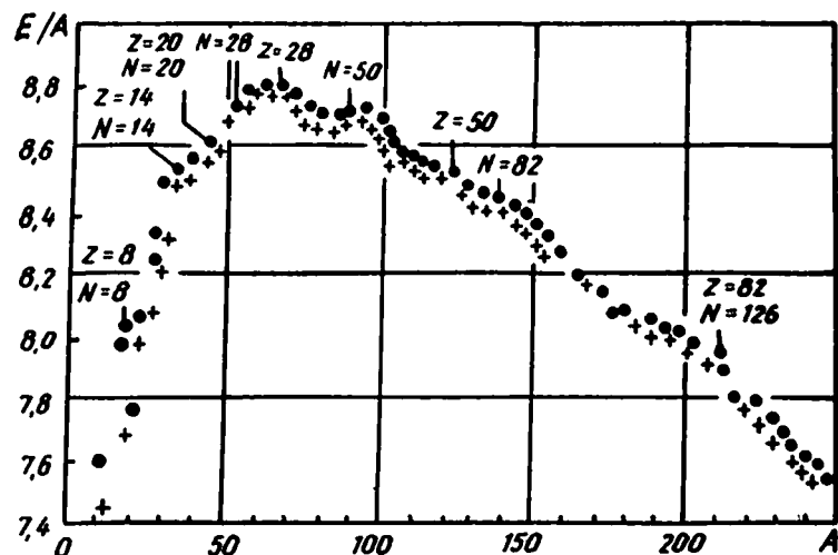
1. 10- расм. Ядродеги ҳар бир нуклонга тўғри келадиган боғланиш энергияси \frac{E}{A} нинг масса сони A га боғлиқлиги (нукталар ж-ж ядролар, «+» белгилар тоқ ядролар учун)
