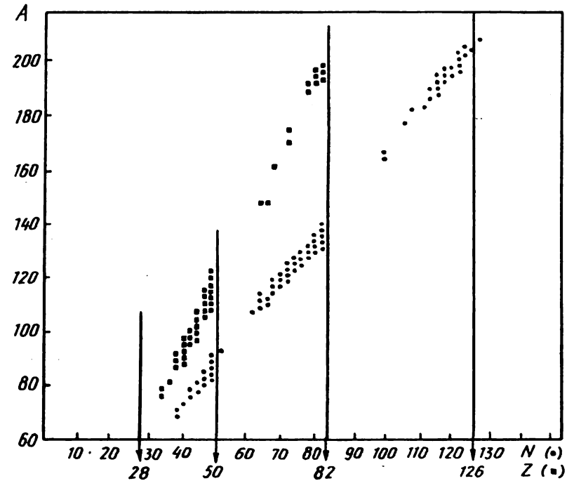
4.18- расм. Узок вақт яшовчи масса сони (A) ток бўлган изомерларнинг ток сонли нуклонлар (Z ёки N — ток) сонига мос тақсимоти.
