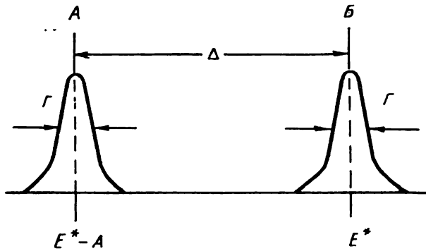
4. 11- расм. Резонанс кўзғатиш учун B частоталар тутами (дастаси) лозим, лекин тепки туфайли \Delta га силжиган A кичик частоталар тутами келади. A ва B частоталар тутамлари оз бўлса-да бир-бирини қоплайди. Агар ҳар хил усуллар билан бу етишмовчи ( \Delta ) энергия қопланса, A^* биринчи сатҳидан чиққан \gamma -квант асосий ҳолатда бўлган A=B ядрони E^* ҳолатга резонанс кўтаради.
