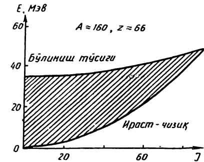
6. 23- расм. Энергиянинг сатҳларнинг спин қийматига боғлиқлигини кўрсатувчи диаграмма.
