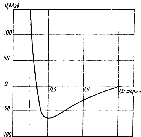
1. 21- расм. Таърибадан олинган протон билан нейтроннинг ўзаро таъсирининг потенциал энергияси.
