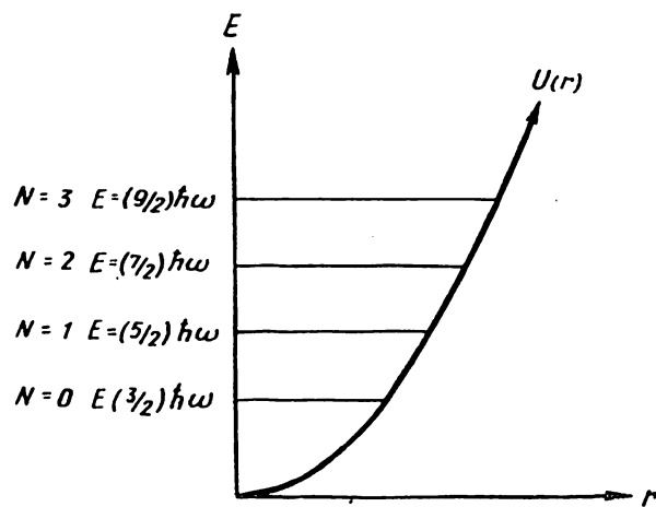
6. 5- расм. Уч ўлчовли гармоник осциллятор ва унинг энергия сатҳлари.
