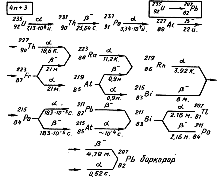
2. 1- в расм. Уран радиоактив онласи.
