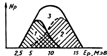
5. 12-расм. Индий ядросидан учиб чиққан фотопротонлар спектри. 1- ва 2-буғланиш ва бевоСИТА фотоэффектив механизмларга тааллуқли назарий эгри чизиклар. N_p — нисбий интенсивлик.
