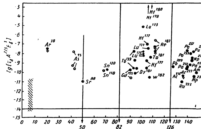
6. 21- расм. Кичик энергияли E1 -ўтишлар учун келтирилган яшаш вақтларнинг N нейтронлар сонига боғлиқлиги. Назарий чизик — бир протонли ўтишларга тегишли сатҳ. Энергиялари МэВ, ярим яшаш вақтлари секундларда берилган.
