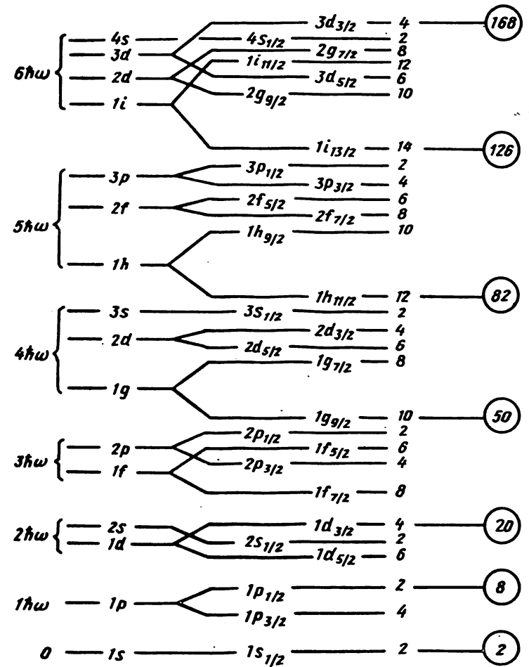
6. 9-расм. Протон ва нейтронлар учун спин-орбитал ўзаро таъсир ҳисобга олинган ҳолдаги ядро сатхларининг диаграммаси. Ҳар бир сатхдаги протон ва нейтронларнинг сони ҳамда «сеҳрли» сонлар кўрсатилган. Осциллятор сатхлар гуруҳи чапда. Нейтрон ва протонлар А-50 гача тахминан бир хил диаграммага эга. Катта А лар учун фарк пайдо бўла бошлайди. Кичик ҳаракат микдори моментларига эга бўлган нейтронлар сатхи кичик моментли протон энергия сатхларидан пастроқ ётади.
