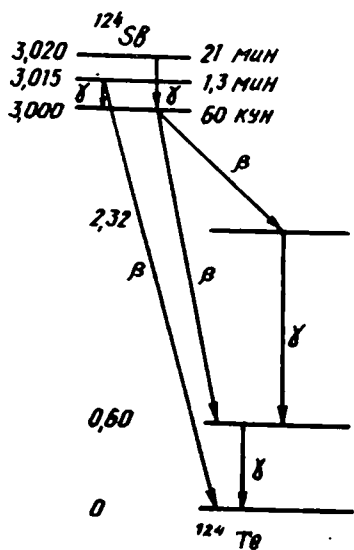
1. 2-расм. Сурьманинг изомер сатҳлари (энергия МэВларда берилган).
