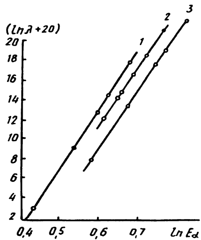
2. 8- расм. «Гейгер--Неттол» коидасининг график ифодаси. 1 — уран, 2 — торий ва 3 эса, актиноуран радио-актив оилаларига мансуб.
