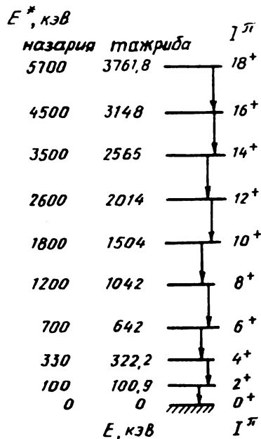
6.13- расм. Деформацияланган ж-ж гафний-170 ядросининг айланма энергия сатхлари схемаси.
