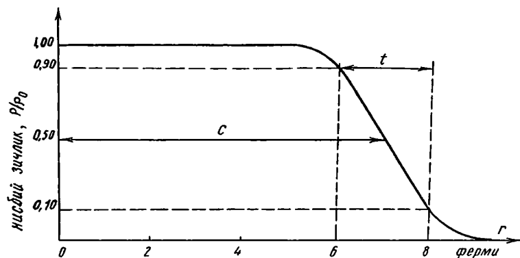
б) Ядродаги зарядлар таксимотининг Ферми функцияси: c — ярим зичлик радиуси, t — сирт қалинлиги.
