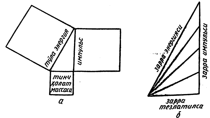
8. 1-расм. Масса, тезлик, импульс ва тўла энергиянинг ўзаро боғлиқлик учбурчаклари: а) тинч ҳолатдаги масса, импульс ва тўла энергия; б) тезлик ортганда, тўла энергия гипотенуза, импульс эса катети каби ортиб боради.
