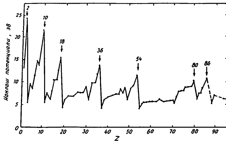
1.13- расм. Нейтрал атомдан электронни ажратиш энергияси — ионизация потенциали.
