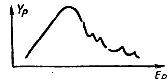
5. 8- расм. (d, p) реакция чиқишининг протонлар энергиясига боғлиқлиги.
