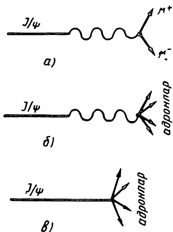
8.12- расм. J/\psi — зарранинг виртуал фотон чиқиш йўли билан лептонлар ( e^+e^- ёки \mu^+\mu^- ) жуфтига (а), ёки адронлар (асосан пионлар) га парчаланиши (б), (в) — расмда эса, J/\psi — зарра оркали фотонсиз, тўғридан-тўғри адронларга парчаланади.
