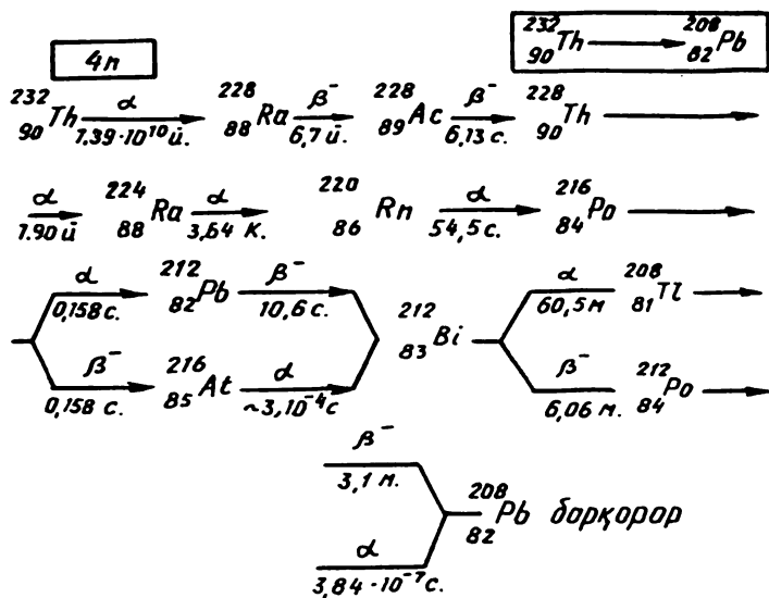
2. 1-г расм. Актиноуран радиоактив оиласи.
