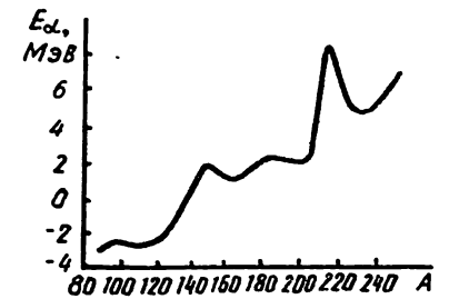
2. 5- расм. Альфа-парчаланиш энергияси.
