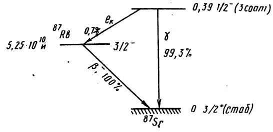
4.16- расм. ^{87}\text{Sr} ядронинг изомер сатҳининг парчаланиши (кэВ).
