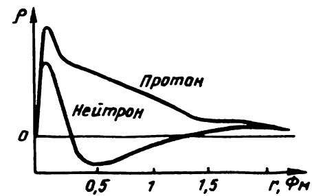
1. 22- расм. Нуклонлар заряднинг тақсимо­ти (водород (протон) ва дейтерий (нейтрон) нишонларида электронлар сочилиши бўйича ўтказилган тажрибалардан олинган би­ринчи натижалар).
