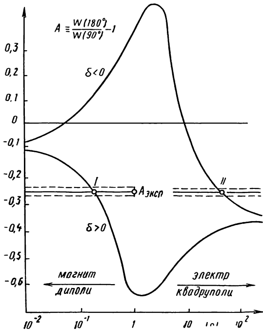
4. 7- расм. ^{111}\text{Cd} нинг сатҳлари \gamma_1 - \gamma_2 каскаднинг \gamma_1 -ўтиши E_2 ва M_1 — ўтишларнинг аралашмасидан иборат, деб тахмин қилинган, \delta^2 = \frac{I(E_2)}{I(M_1)} E_2 ва M_1 — ўтишлар интенсивликлари нисбати. Бунда A_{\gamma_1 - \gamma_2} — каскаднинг анизотропияси. Ҳар икки чизик маълум \delta га тегишли, аралашмиш нисбати \delta ни экспериментга тўғриси расмда I қилиб белгиланган.
