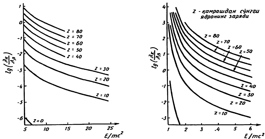
3. 9-расм. K — камраш эҳтимолликларининг \beta^+ -парчаланиш эҳтимолликларига нисбати.
