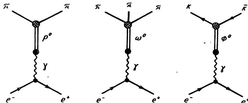
8.8-расм. Виртуал фотоннинг ( e^+e^- ) вектор мезонларга айланиши парчланиши қарама-қарши йўналтирилган электрон ва позитрон дасталаридаги тажрибаларда кузатиловчи резонанслар ҳосил бўлишига олиб келади. Бу диаграммалар \rho^0 , \omega^0 , \phi^0 вектор мезонларнинг ( e^+e^- ) дасталарида тугилишини кўрсатади.
