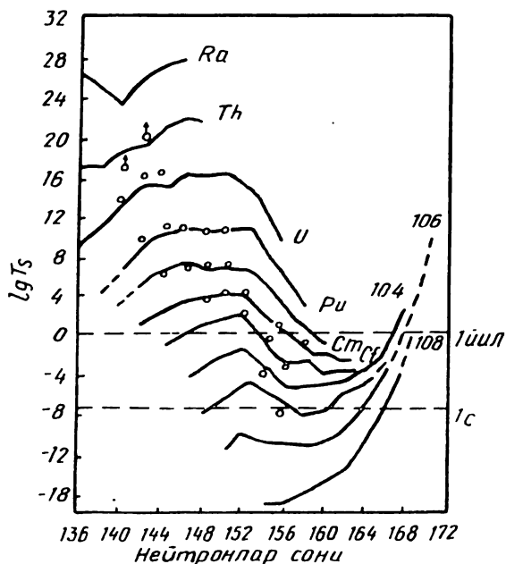
7. 5- расм. Трансурани элементлар изотопларининг спонтан бўлиниш давларининг янги назарияга асосланиб ҳисобланган кийматлари.
