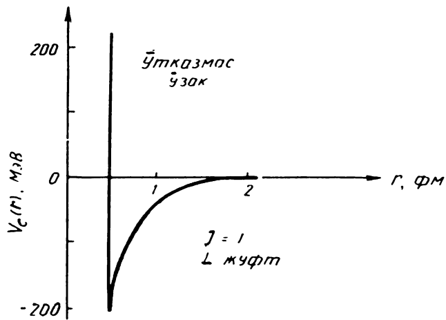
8. 4- расм. Мусбат жуфтликли спин-триплет ҳолатларида таъсир қилувчи нуклон-нуклон кучларининг марказий симметрик ташкил этувчилари учун Ямада — Жонсон потенциалининг кўриниши.
