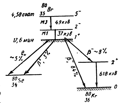
3.3-расм. {}^{80}\text{Br} — изомерларининг парчаланиш схемаси.
