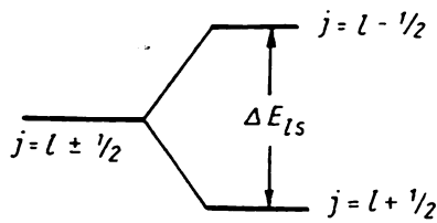
6. 8-расм. l моментга эга бўлган сатхнинг иккита сатхга ажралиши. Спин-орбитал ўзаро таъсир тўла ҳаракат микдори momenti j = l + 1/2 бўлган сатхни камайтириб, j = l - 1/2 бўлган сатхни кўтареди.
