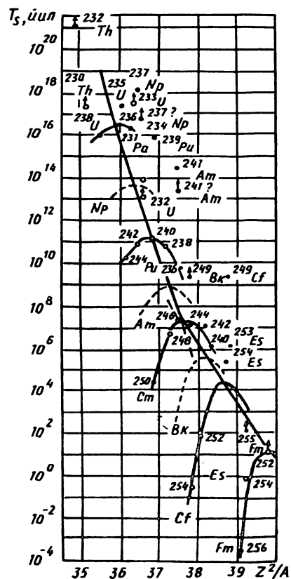
7. 3-расм. Спонтан бўлиниш эҳтимоллигининг бўлиниш параметрига боғлиқлиги.
