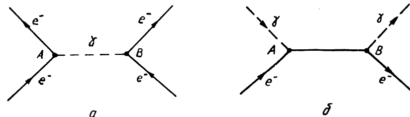
8.5- расм. Фотоннинг электронда сочилишининг Фейнман диаграммаси.
