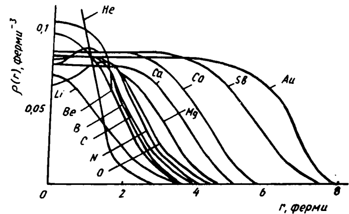
1. 4-расм. а) Ядроларда электрон сочилиши бўйича ўтказилган тажрибалардан олинган зарядлар тақсимоти.
