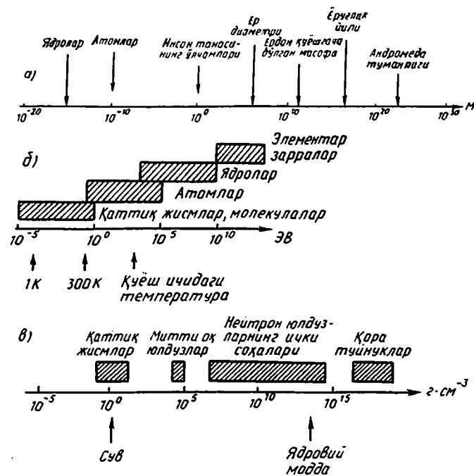
1. 1-расм. а) Характерли масофалар. Тахминан 10^{-17} м дан кичик соҳалар яхши ўрганилмаган. Ҳозирги пайтда бу соҳаларда янги турдаги кучлар ва янги ҳодисаларнинг кашф қилиниши кутилмоқда; б) Қўзғатиш энергияларининг характерли катталиклари. Шунингдек, кўрсатилган энергияларга мос келувчи температуралар кийматлари ҳам берилган; в) Зичликларнинг характерли кийматлари.
