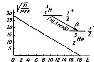
3.7-расм. Ўта рухсат этилган \beta -спектр учун Ферми графиги.
