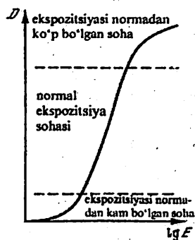
69-rasm. Fotomaterialning xarakteristik egriligi
