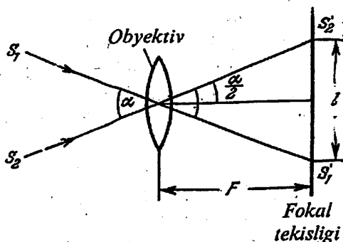
61-rasm. Fotografik tasvirning chiziqli o'lchami
