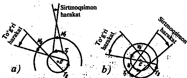
24-rasm. Sayyoralarning sirtmoqsimon harakatlari va ularni tushuntirish
