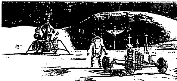
99-rasm. Oy sirtini «Apollon» ekipaji yordamida tekshirish
