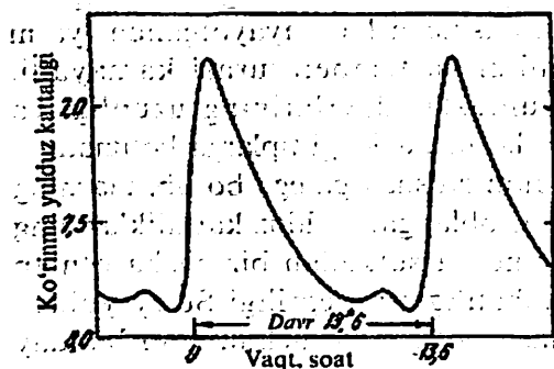
140-rasm. Liraning RR yulduzi ravshanligi o'zgarish grafigi
