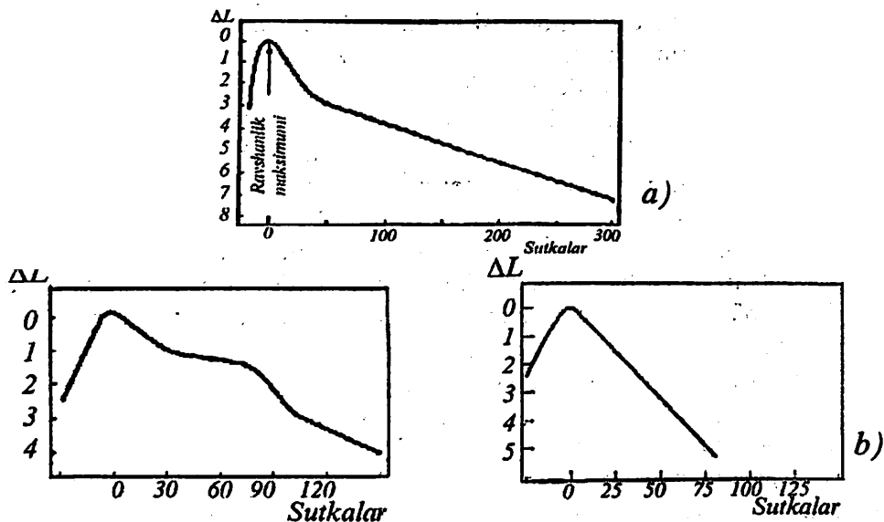
144-rasm. O'ta yangi yulduzning chaqnash egriligi
