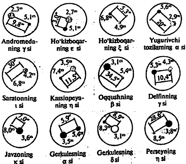
131-rasm. Bir guruh taniqli qo'shaloq yulduzlar
