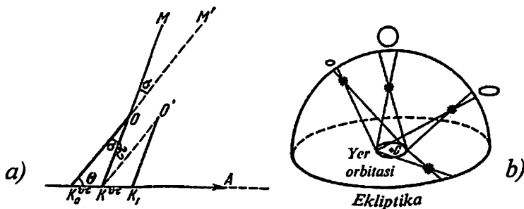
39-rasm. Yoritgichlarning yillik parallaksini aniqlash
