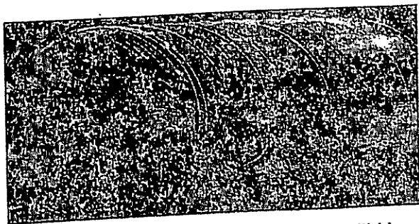
85-rasm. Xromosferaning emission spektri (Quyosh to'la tutilishi paytida olingan)
