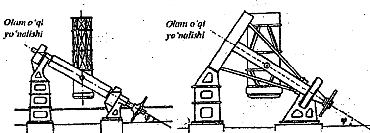
68-rasm. Massiv teleskoplarni rama yordamida parallaktik qurilma ko'rinishiga o'rnatish
