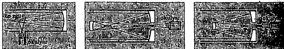
58-rasm. Teleskopik sistemalar:
