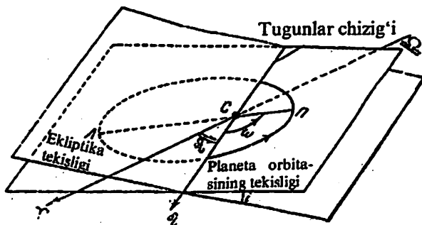
26-rasm. Sayyoralarning orbita elementlari
