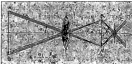
57-rasm. Refraktor teleskopida nurning yo‘li
