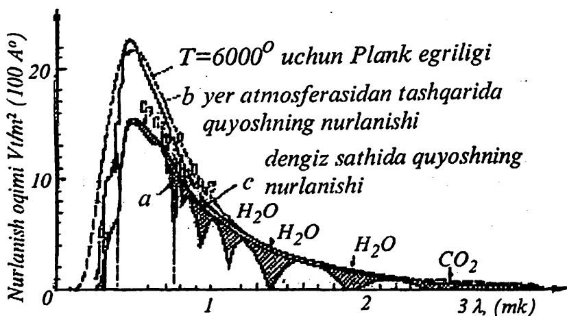
53-rasm. Absolyut qora jism nurlanish spektrida energiyaning to'liq uzunligi bo'yicha taqsimlanish grafigi
