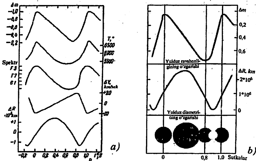
138-rasm. a) sefeidlar ravshanligi, temperaturasi, spektral sinfi, nuriy tezligi va radiuslarining o'zgarishi, b) sefeyning \delta yulduzi ravshanligi o'zgarishining radiusiga bog'liqlik grafigi
