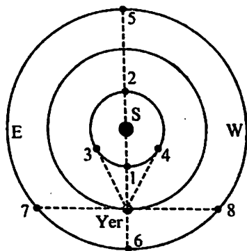
25-rasm. Ichki va tashqi sayyoralarning konfiguratsiya holatlari
