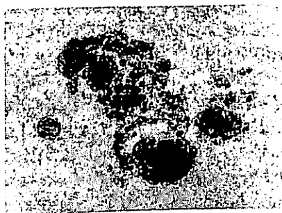
81-rasm. Quyosh sirtidagi dog' guruhlari
