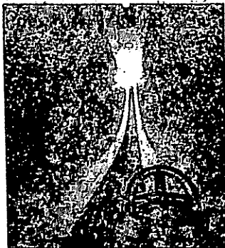
72-rasm. Ulug'bek rasadxonasi bosh «teleskopi» – sekstantining qoldiqlari
