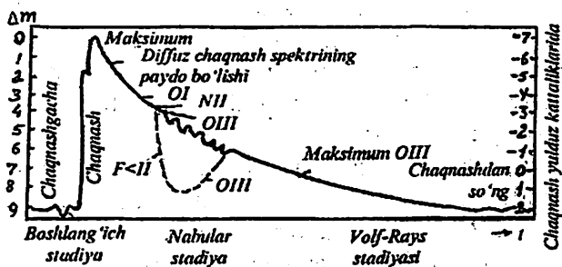
143-rasm. Yangi yulduzning chaqnash egriligi
