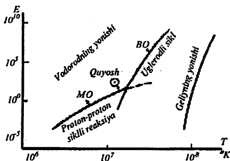
128-rasm. Yadroviy reaksiyalardan ajraladigan energiyaning temperaturaga bog'liqligi
