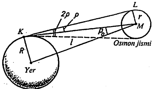
37-rasm. Quyosh sistemasi jismlarining chiziqli o'lchamlarini hisoblash.
