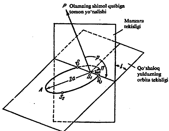
134-rasm. Qo'shaloq yulduzning orbita elementlari
