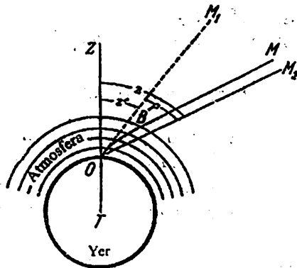
18-rasm. Astronomik refraksiya hodisasi
