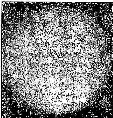
86-rasm. Quyoshning vodorodning H \alpha chizig'iga tegishli spektrogeliogrammasi
