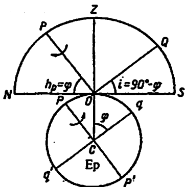
7-rasm. Olam qutbining balandligi va joyning kenglamasi orasidagi bog'lanish
