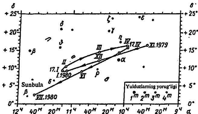
21-rasm. Sayyoraning yulduzlar fonidagi sirtmoqsimon harakati
