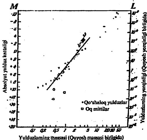
126-rasm. Yulduzlarning yorqinliklari va massalari orasidagi bog'lanish
