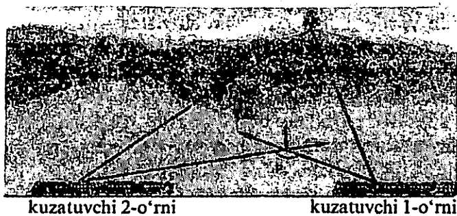
33-rasm. Ikki nuqtadan qaralganda jismning parallaktik siljishi
