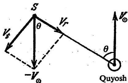
152-rasm. Yulduzlarning fazoviy tezligini topish
