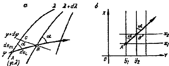
36-rasm. Loksodromiya va uning tasviri: a) ellipsoidda; b) yuzada
