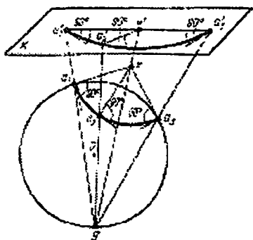
30-rasm. Stereografik proyeksiyaning asosiy xossasini isbotlash sxemasi
