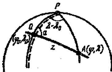
19-rasm. Qiyshiq tizimning z va a sferik koordinatalari
