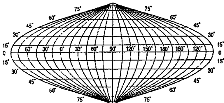
43-rasm. Teng maydonli sinusoidal psevdosilindrik Sanson proyeksiyasi
