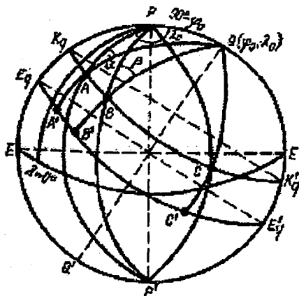
21-rasm. Berilgan uchta nuqta bo'yicha (A, B, C) qutb koordinatalarini hisoblash chizmasi
