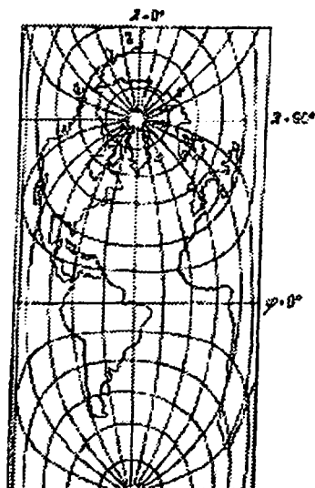
39-rasm. Vertikallar bo'yicha teng oraliqli ko'ndalang silindrik proyeksiya
