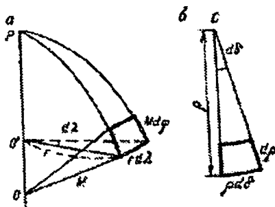
23-rasm. Cheksiz kichik trapetsiya: a – ellipsoidda; b – konusli proyeksiyada
