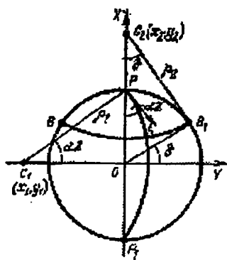
55-rasm. Lagranj proyeksiyasi koordinatalari tizimi.
