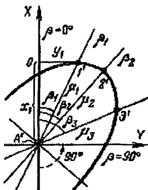
8-rasm. Xatoliklar ellipsi elementlari
