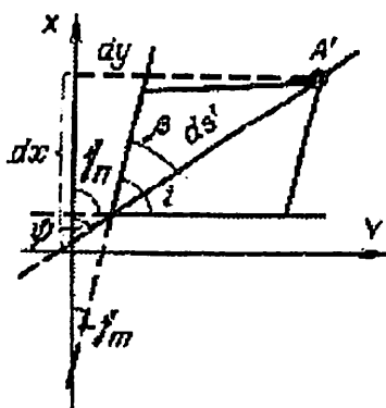
6-rasm. Proyeksiyada azimutni tasvirlash
