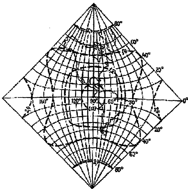
68-rasm. Adams proyeksiyasida r izokolalari
