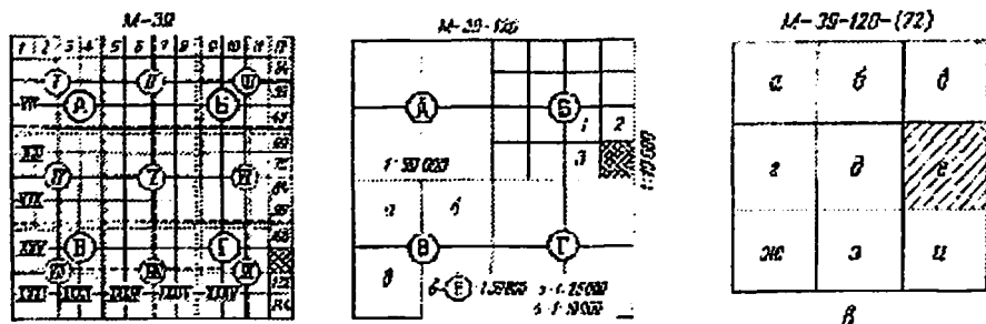
63-rasm. Sobiq Ittifoq topografik kartalarining razgrafkalarini ishlab chiqish va ularning nomenklaturasi
