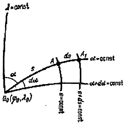
2-rasm. Qutbiy geodezik koordinatalar tizimi
