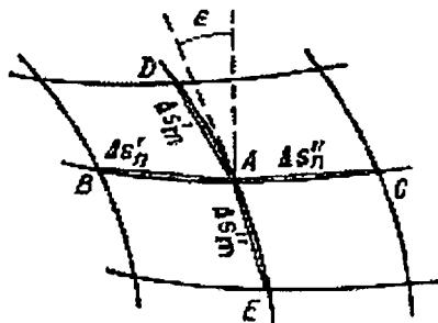
51-rasm. m va n qiymatlarini aniqlash chizmasi
