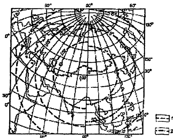
34-rasm. «Sinus tarmoq»li azimutal proyeksiyalarda t (1) va \omega (2) izokollari
