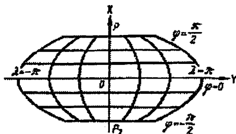
42-rasm. Psevdosilindrik proyeksiyalar koordinatalari tizimi
