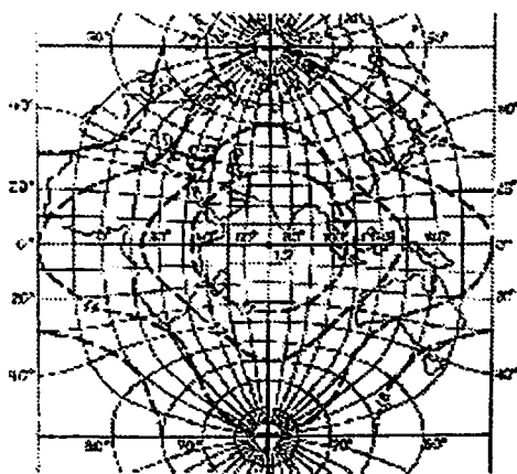
66-rasm. Gyuy proyeksiyasida p izokollari
