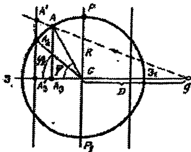
40-rasm. Normal perspektiv-silindrik proyeksiyani hosil qilish
