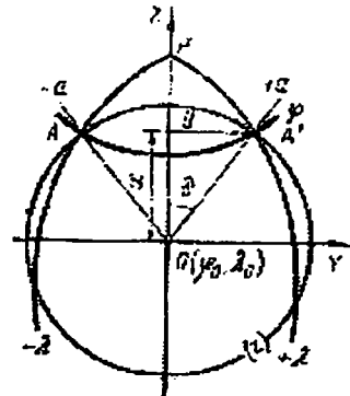
27-rasm. Qiyshiq va ko'ndalang azimutal proyeksiyalarda koordinatalar tizimi
