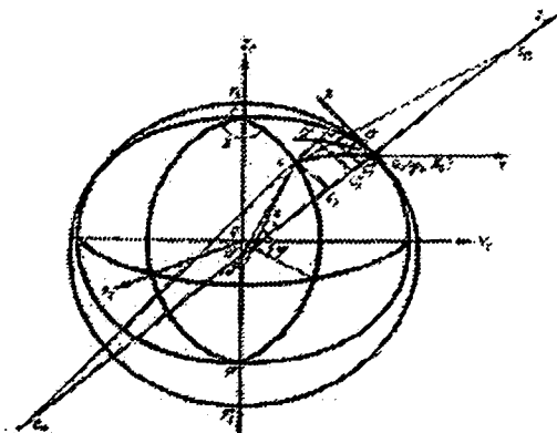
11-rasm. Sferada ellipsoidni perspektiv tasvirlash
