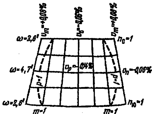
58-rasm. 1:1 000 000 mashtabli karta varag'ida xatoliklarning taqsimlanishi.
