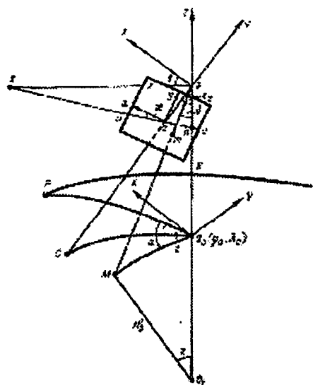
33-rasm. Qiyshiq tasvir tekisligida perspektiv-azimutal proyeksiyani pozitivli tasvirlash
