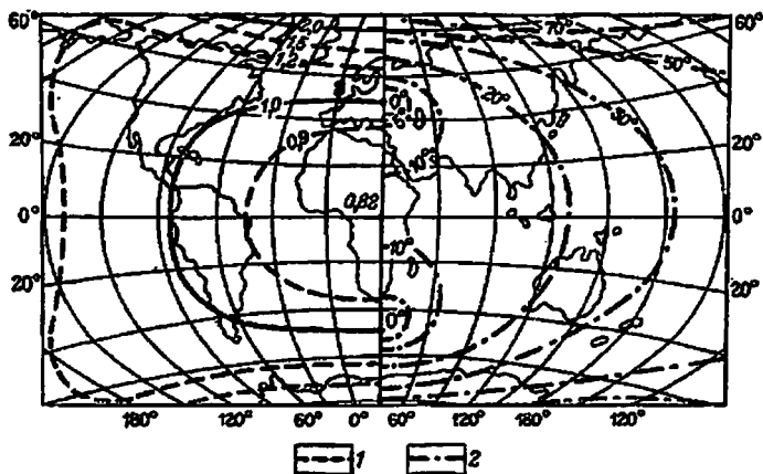
54-rasm. Dunyo kartasida yarim konusli proyeksiya izokolalari – r (1) va \omega (2).
