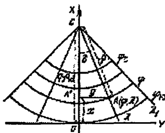
22-rasm. Normal konusli proyeksiyada koordinatalar tizimi
