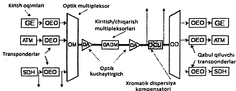
5.7-rasm. DWDM texnologiyasining ishlash tamoilini tushuntiruvchi sxemasi
