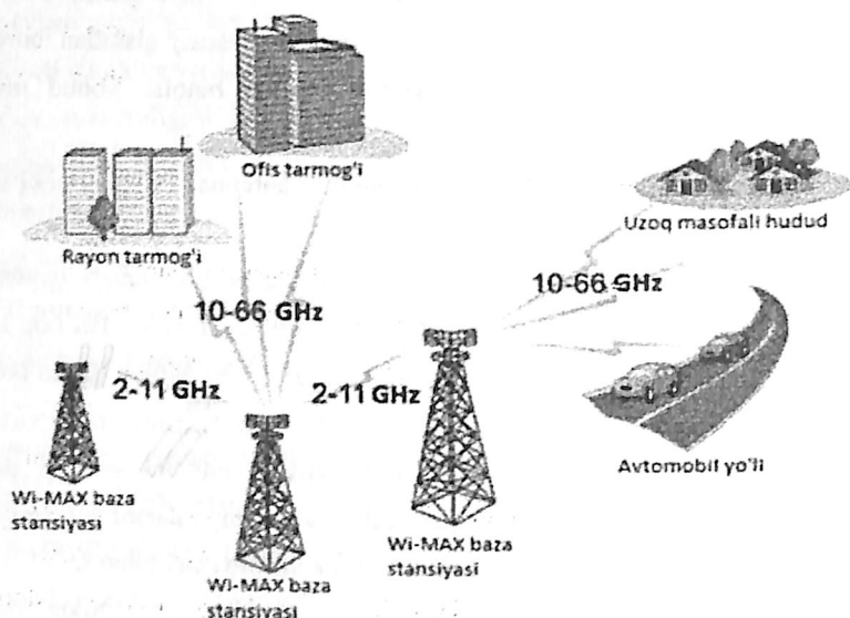
9.1-rasm. Wi-MAX stansiyalararo aloqa tarmog'i
