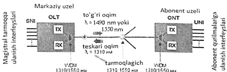
4.19-rasm. PON tarmog'idagi asosiy elementlar va ishlash prinsipi
