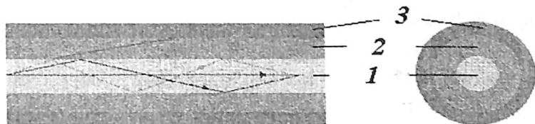
2.8-rasm. Optik tola va uning asosiy elementlari
