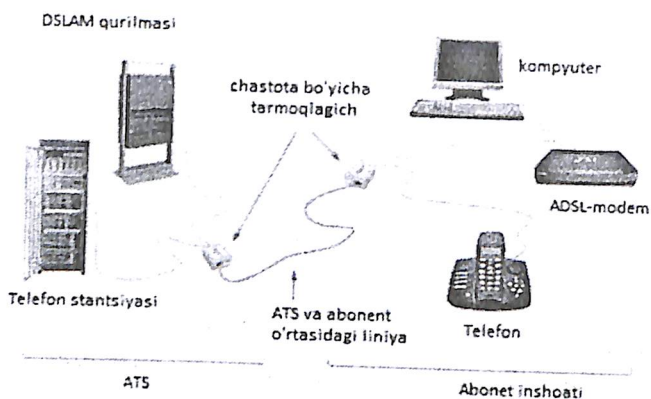
4.4-rasm. ADSL asosida raqamli abonent kirish tarmoqlarini qurishda qo'llaniluvchi qurilmalarning ulanish ketma-ketligi ifodalangan
