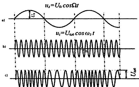
3.4-rasm. Chastota bo'yicha modulyatsiya jarayoni a – past chastotali foydali signal; b – yuqori chastotali tashuvchi signal; c – chastota bo'yicha modulyatsiyalanga signal.
