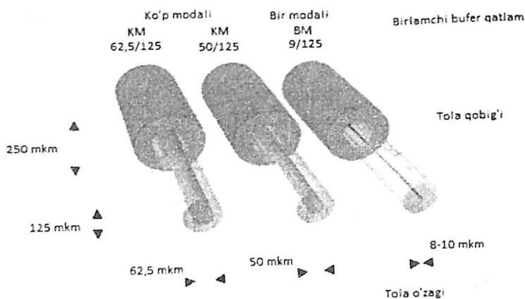
2.10-rasm. Bir va ko'p modali optik tolalar va ularning geometrik parametrlari
