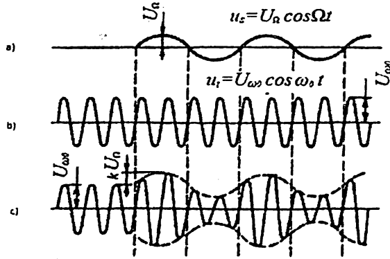
3.2. Amplituda bo'yicha modulyatsiya jarayoni. a – past chastotali foydali signal; b – yuqori chastotali tashuvchi signal; c – amplituda bo'yicha modulyatsiyalangan signal
