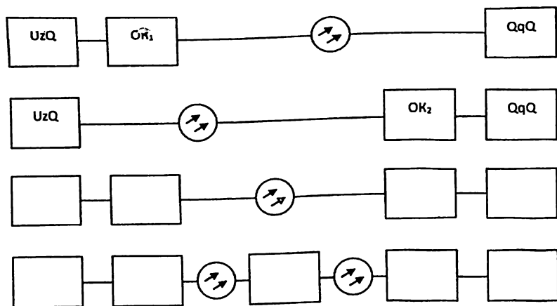
10.1-rasm. Turli optik kuchaytirgichlarni qo'llash sxemalari
