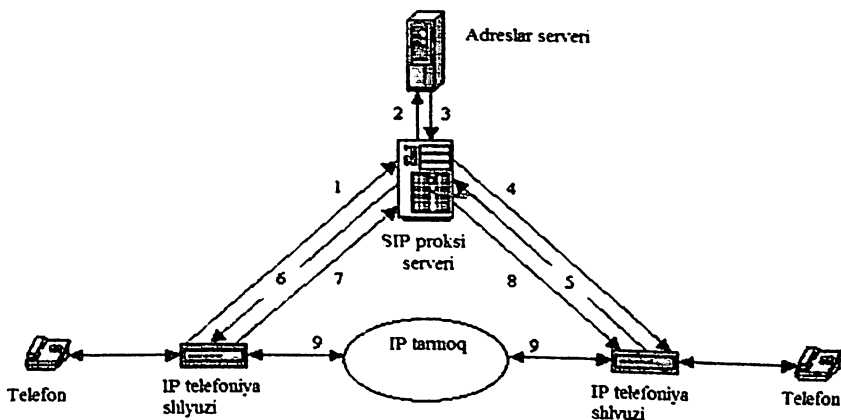
8.3-rasm. SIP protokoli IP tarmoq orqaqli telefoniya'ni ta'minlashda qo'llanilishi
