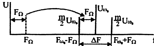
3.3-rasm. Amplituda bo'yicha modulyatsiyalangan signalning spektri
