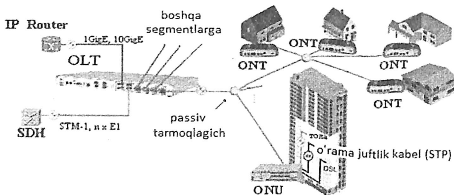
4.15-rasm. PON texnologiyasi asosida qurilgan passiv optik tarmoqning prinsipl sxemasi
