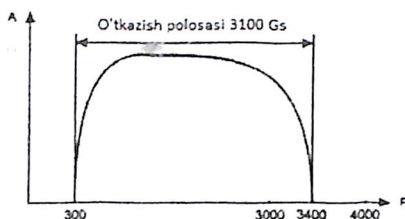
3.7-rasm. Standart telefon kanalining amplituda-chastotaviy harakteristikasi
