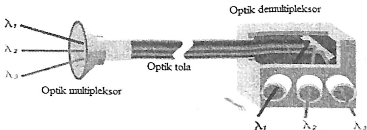
5.3-rasm. DWDMning optik multipleksor va demultipleksorlarini ishlash prinsipi
