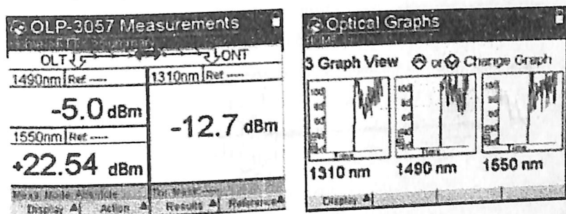
11.3-rasm. PON tarmoqlarida satxlarni o'lchash
