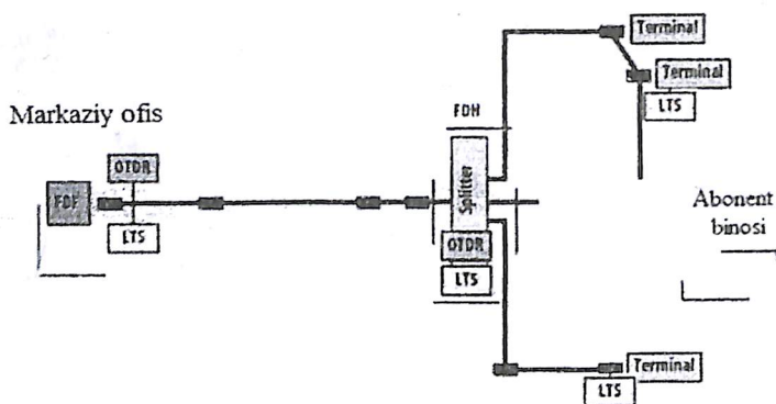
11.4-rasm. PON tarmog'i qurilishida testlash o'lchoq qurilmasining ulanish sxemasi
