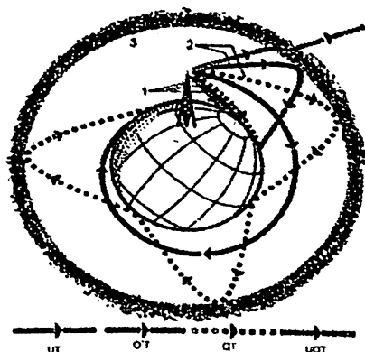
2.1-rasm. Turli to‘lqinlarning tarqalish xususiyatlari
