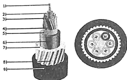
2.12-rasm. Tuproq va suv ostiga yotqiziluvchi o‘rama zirxli optik tolali kabelning ichki tuzilishi.
