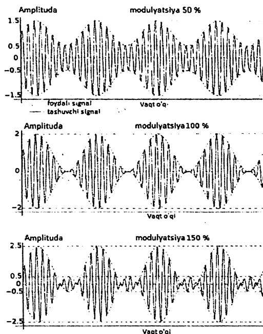
3.3-rasm. Turli modulyatsiyalash koeffitsiyentlarida modulyatsiyalash jarayoni. Eng quyi ossilogrammada ortiqcha modulyatsiyalanish yuzaga kelgan
