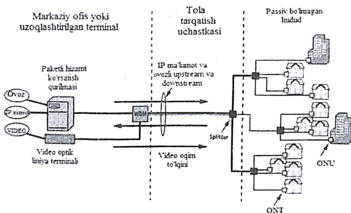
11.1-rasm. FTTx tarmog'i strukturasi
