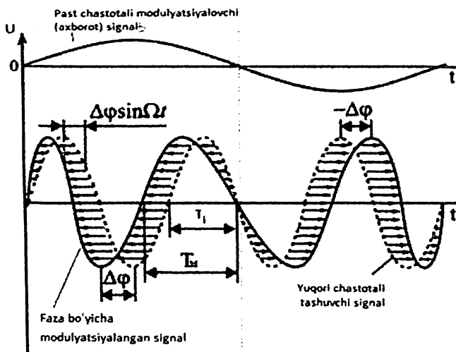
3.6 – rasm. Tashuvchini faza bo'yicha modulyatsiyalash jarayoni
