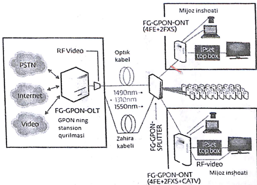
7.3-rasm. GPON tarmoqlarini qurish sxemasi
