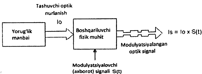
3.16-rasm. Tashqi modulyatsiya jarayonining ishlash tamoili
