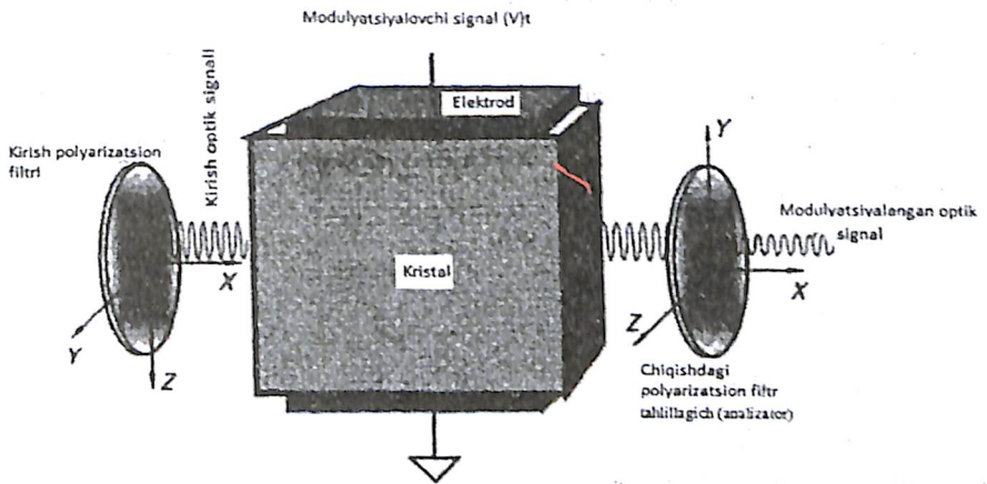
3.10-rasm. Chiziqli elektrooptik hodisa asosida ishlaydigan elektrooptik modulyatorning tuzilishi
