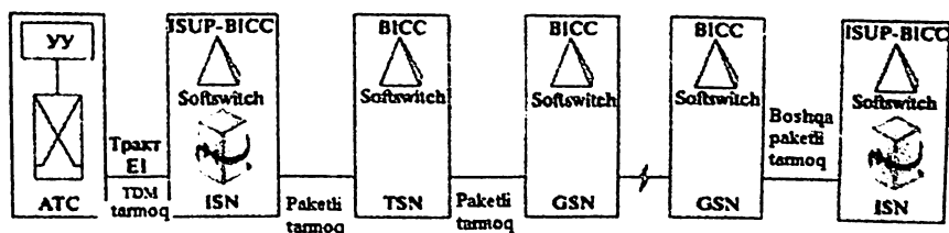
8.4-rasm. BICC protokolinig ishlash tamoyili
