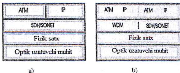
5.5-rasm. Asosiy transport texnologiyalarining modelini o'zaro bog'lanishi A) WDM texnologiyasi yaratilgunga qadar;
