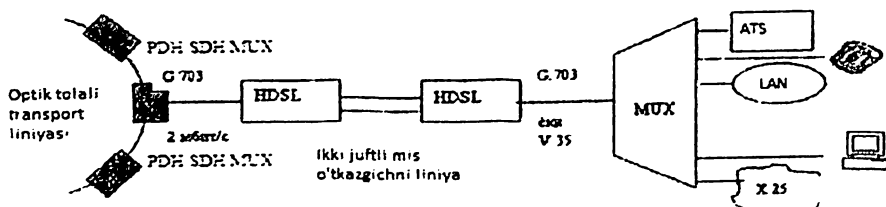
4.7-rasm. HDSL texnologiyasi asosidagi abonent ulanish liniyasi
