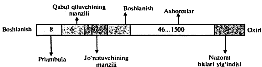
6.2 – rasm. Ethernet tarmog'ida uzatiluvchi paketining tuzulishi va uning xajmiy miqdori (bayt)
