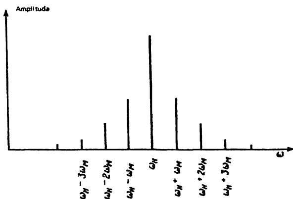
3.6-rasm. Chastota bo'yicha modulyatsiyalangan signal spektri \omega_H -tashuvchi chastota ; \omega_M - modulyatsiyalash chastotasi.
