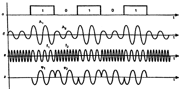
3.8-rasm. Diskret ma'lumotlarni uzatishda qo'llaniluvchi turli hil monipulyatsiya usullari
