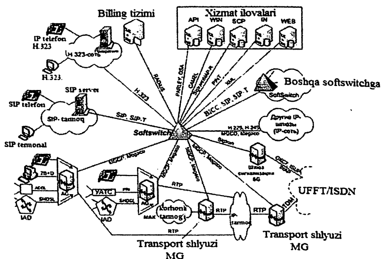
8.1-Rasm. Keng polosali xizmatlarni taqdim etuvchi multiservis tarmog'ida protokollar qo'llanilishi
