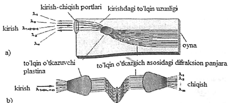
5.6-rasm. WDM da multipleksorlash jarayoni
