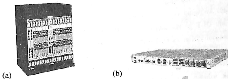
4.17- rasm. GPON/ EPON ga xos bo'lgan katta xajmdagi OLT qurilmasi (a) va GPON ning kam xajmdagi ixcham markaziy uzeli OLT qurilmasi (b).
