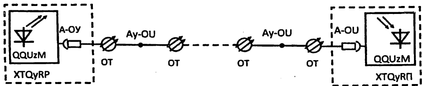
10.2-rasm. RTOU regeneratsiyalash uchastkasining hisobiy sxemasi
