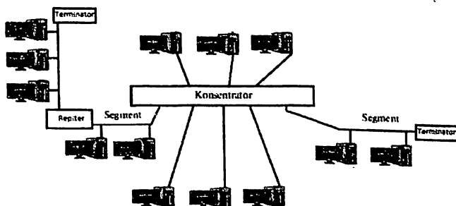
6.1 – rasm. Ethernet tarmog'i va unda tarmoq elementlarining ulanish topologiyasi
