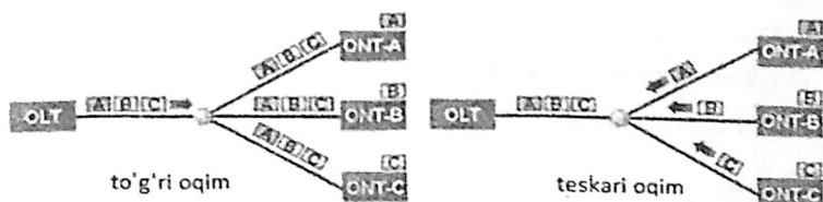
4.20-rasm. PON tarmog'ida to'g'ri va teskari oqimning yuzaga kelishi
