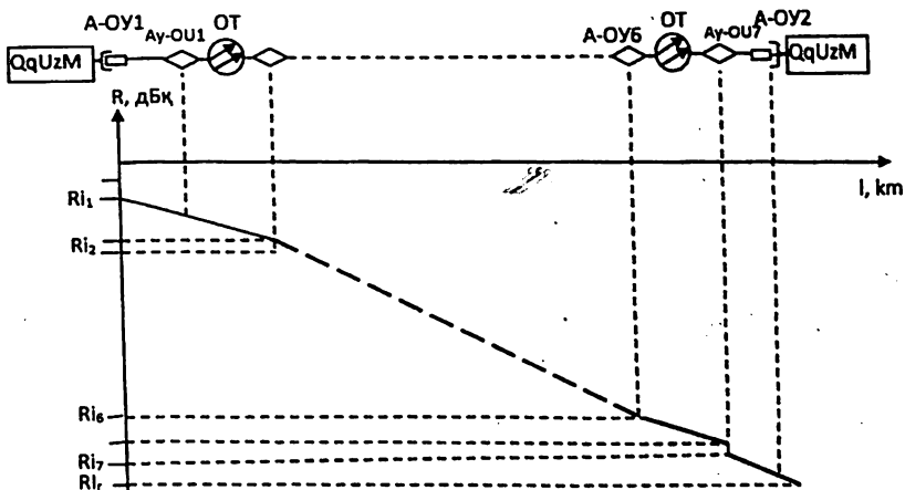
10.3-rasm. Energetik potensialning taqsimlanish diagrammasi
