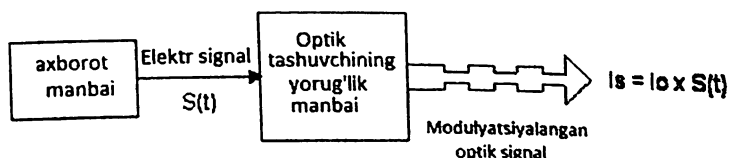
3.17-rasm. To'g'ridan-to'g'ri modulyatsiyalash usulining ishlash tamoili
