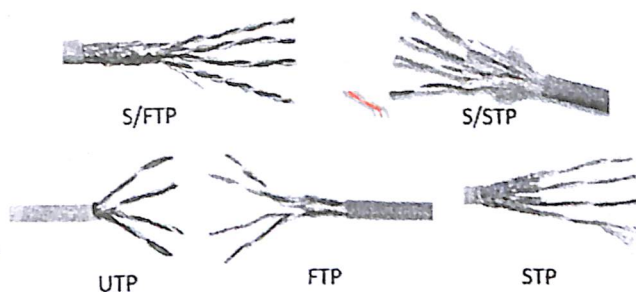
2.4-rasm. Simmetrik o'rama juftli kabellarning turlari
