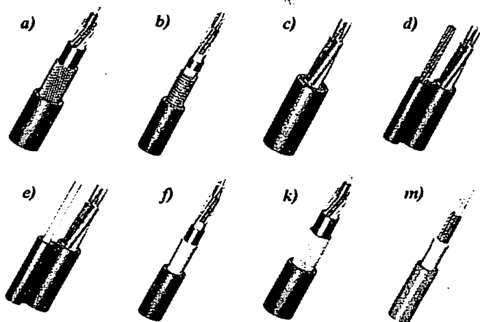
2.11-rasm. Optik tolali aloqa kabellari konstruksiyalari.
