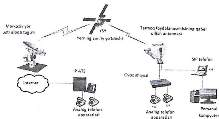
2.3-rasm. Sun'iy yo'ldoshi aloqa tizimining tashkil etilishi
