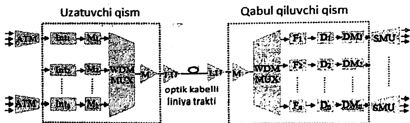
5.4-rasm. WDM asosidagi tizimlarning asosiy sxemasi
