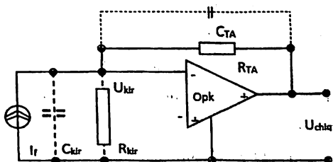
10.4-rasm. Fotodetektor kuchaytirgichining tipli sxemasi
