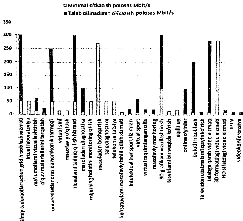
7.1-rasm. Xizmatlarni taqdim etish uchun zarur bo'lgan tarmoqning polosa kengligi
