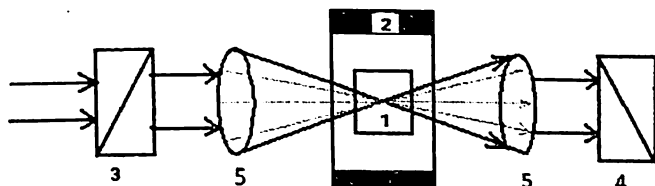
3.15- rasm. Magnitooptik modulyatorning tuzilish sxemasi.
