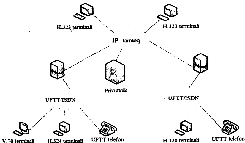
8.2-rasm. H.323 tarmog'i strukturasi
