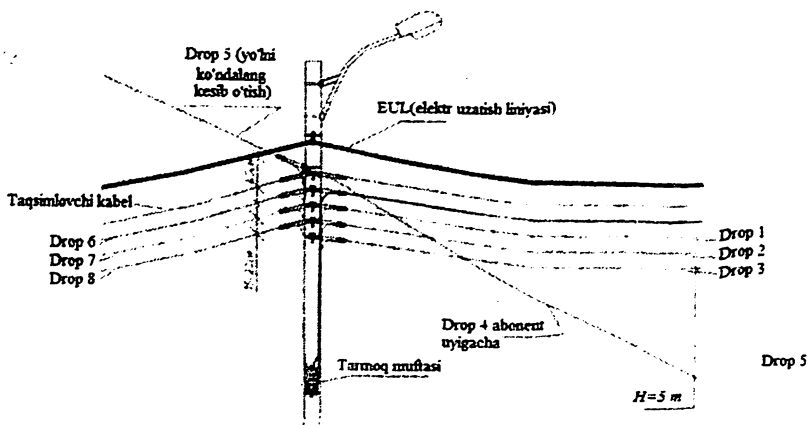
9.10-rasm FTTC havo aloqa liniyasini qurishda optik kabellarni tayanchlarga vertikal usulda osish texnologiyasi qo'llanilishi
