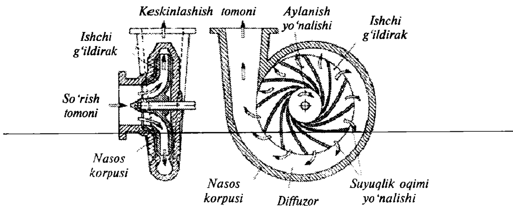
3.7-rasm. Nasos va uning kesimda koʻrinishi.
