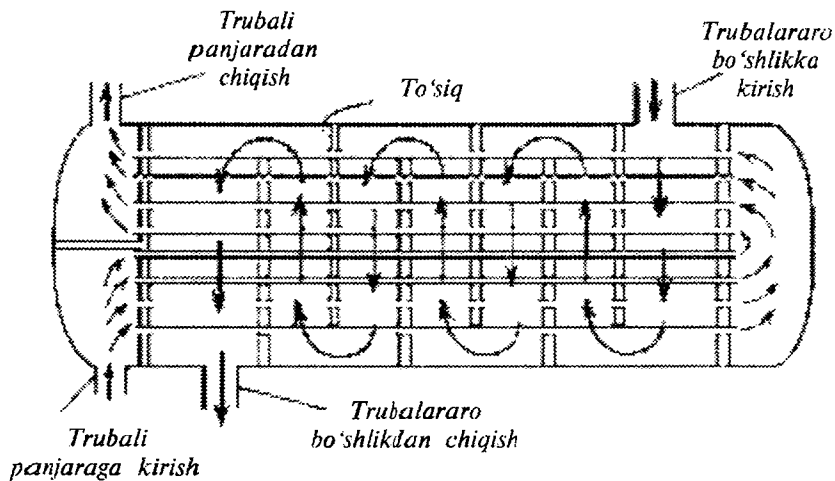
7.2-rasm. Sirtqi issiqlik almashinish qurilmasi (qobiq quvurli).
