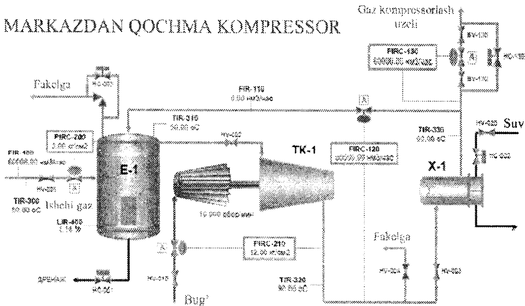
5.4-rasm. Kompressorlash tugunlari sxemasi
