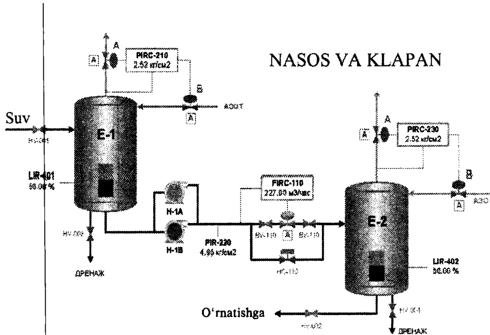
3.9-rasm. Ikkita sig'imdand iborat texnologik qurilma
