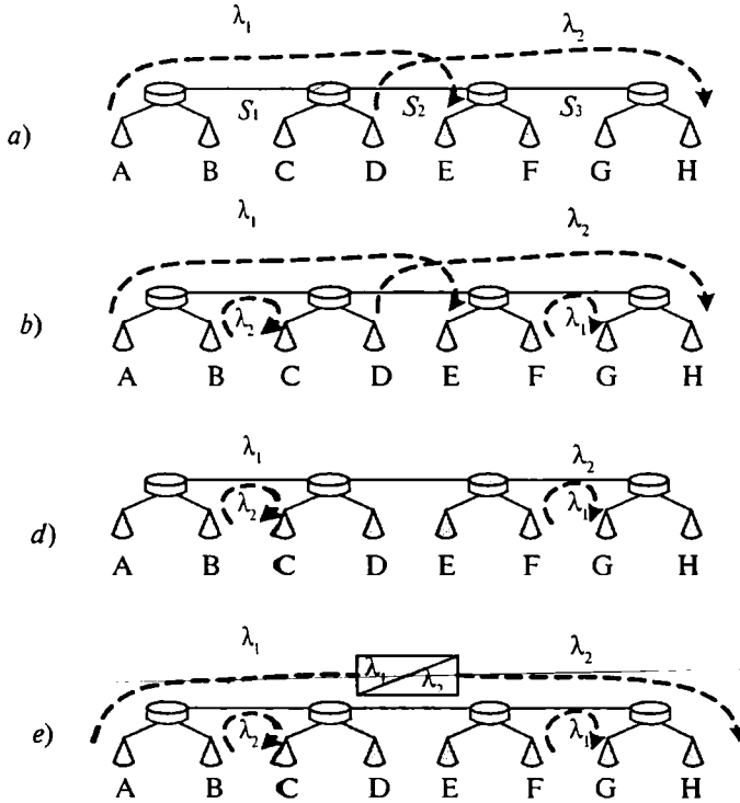
12.5-rasm. Dinamik to‘lqin marshrutlashtirishli optik tarmoq: a–d – tarmoqda to‘lqin konversiyasiz vujudga keladigan cheklanishlar; e – to‘lqin konversiyasi tarmoqni yanada o‘zgaruvchan qiladi
