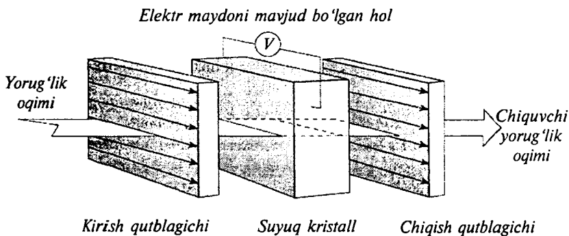
8.4-rasm. Suyuq kristallarda elektr maydoni ta'sirida qutblanish tekisligining o'zgarishiga asoslangan filtrning ish jarayoni
