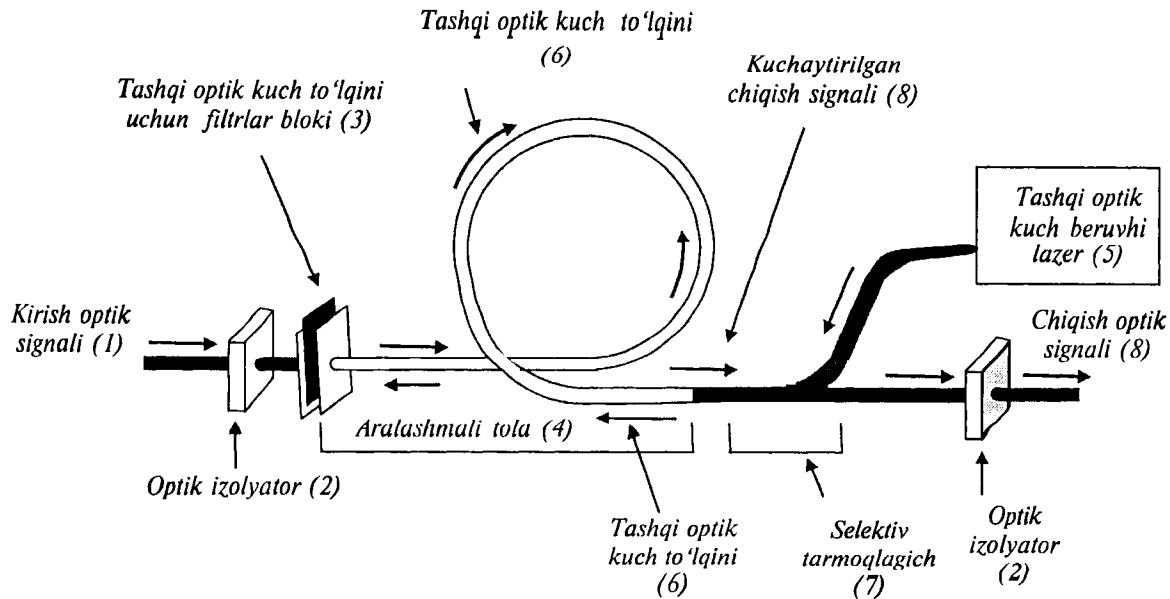
5.1-rasm. Aralashmali optik kuchaytirgichning tuzilishi
