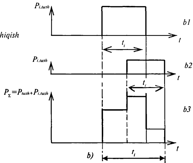
7.1-rasm. Yorug'likning takroriy aks etish natijasida nurlanish impulslari shaklining buzilishi:
