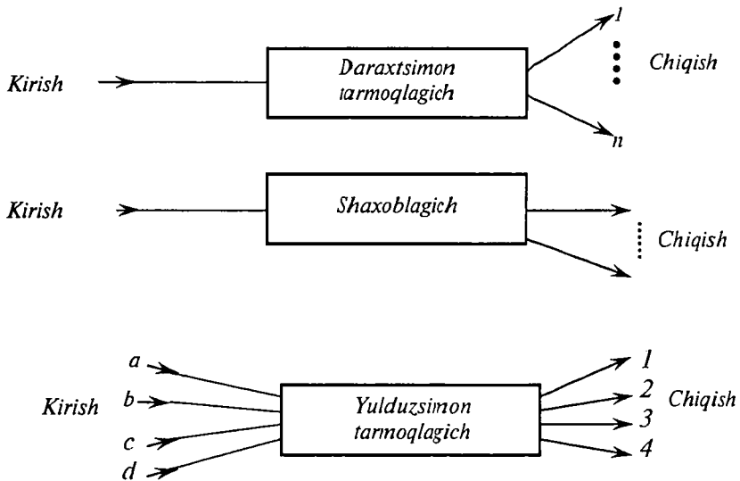
7.6- rasm. Optik tarmoqlagichning turlari: a – daraxtsimon tarmoqlagich; b – shahoblagich; d – yulduzsimon tarmoqlagich
