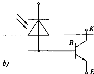
4.14-rasm. Fotodiod-tranzistorning tuzilishi (a) va elektr sxemasi (b)
