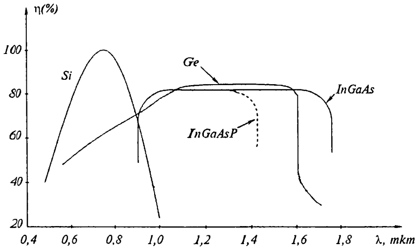
4.15-rasm. Yarimo'otkazgichlarning kvant samaradorligi va to'qin uzunligi orasidagi bog'lanish grafigi
