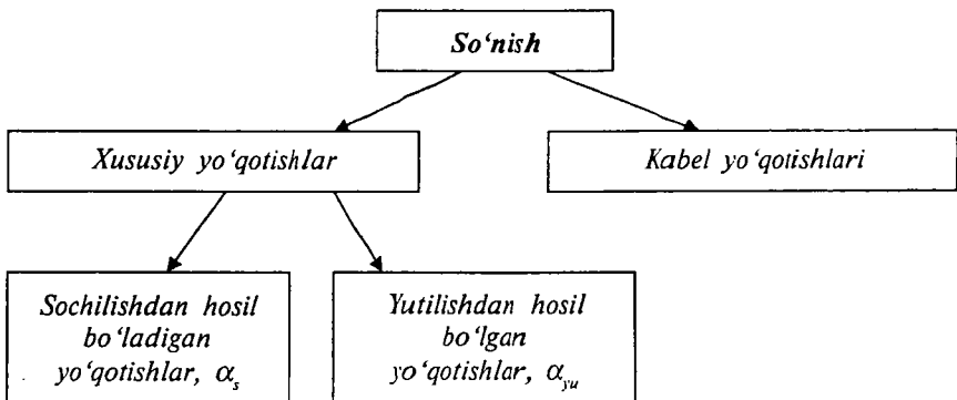
2.14-rasm. Toladagi yoʻqotishlarning asosiy turlari
