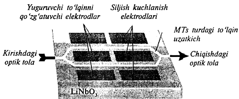
6.7-rasm. Max-Tsender interferometri turidagi elektrooptik modulyatorning tuzilish sxemasi.
