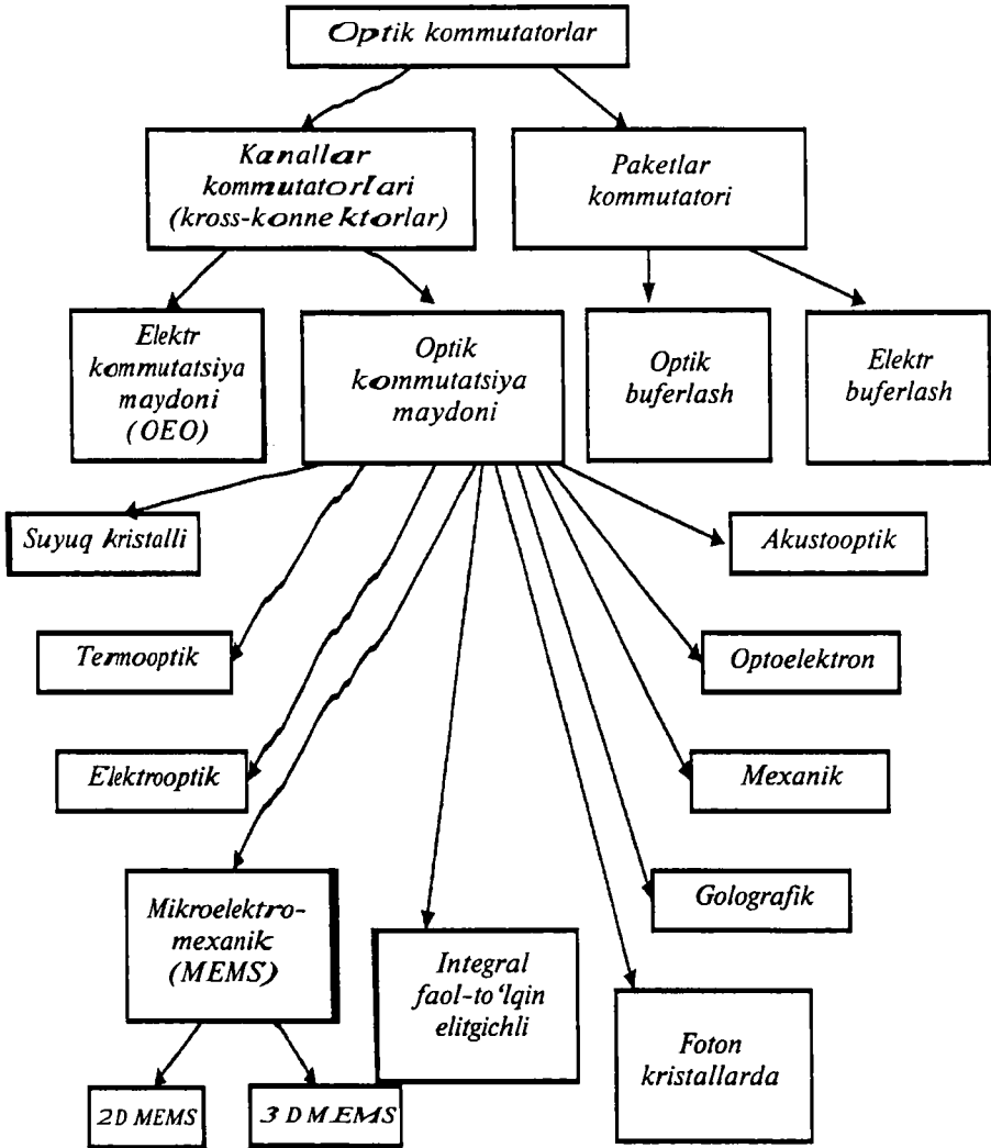
10. 2.-rasmi. Optik kommutatorlar tasnifi
