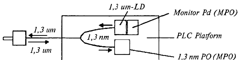
7.10-rasm. NEL firmasi tomonidan ishlab chiqilgan transiverning tuzilish sxemasi
