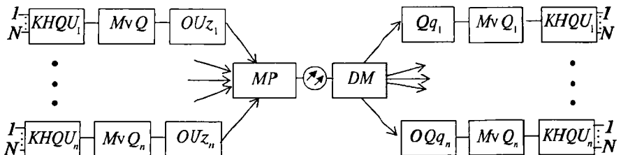
1.8-rasm. To‘lqin uzunligi bo‘yicha zichlashtirilgan TOATning tuzilish sxemasi
