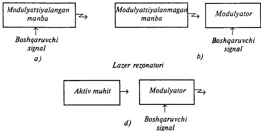
6.1-rasm. Yorug'lik nurlanishini to'g'ridan to'g'ri (a), tashqi (b) va ichki (d) modulyatsiyalash usullari
