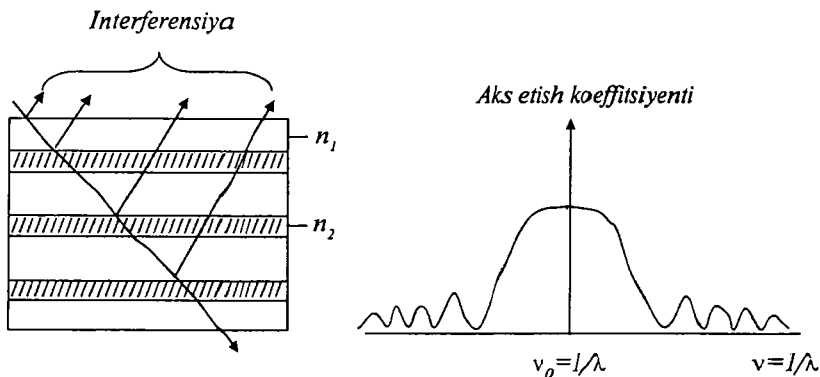
8.3-rasm. Ko‘p qatlamli dielektrik tuzilishli filtrning ish prinsipi:
