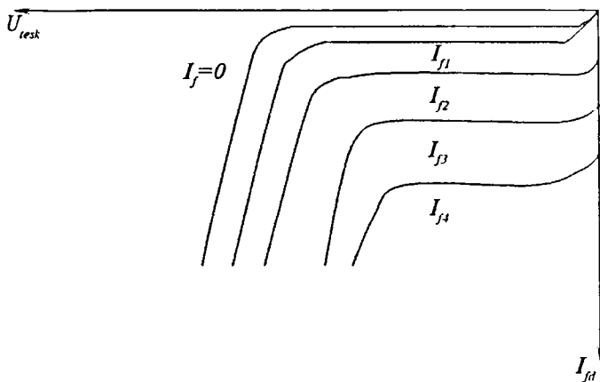
4.11-rasm. Ko'chkili fotodiodning volt-ampere xarakteristikalari oilasi
