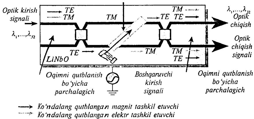
8.5-rasm. Akustooptik qayta sozlanuvchi filtrning tuzilishi
