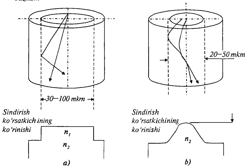
2.4-rasm. Pog'onali (a) va gradientli (b) ko'p modali optik tolalarning tuzilishi va sindirish ko'rsatkichining ko'rinishlari
