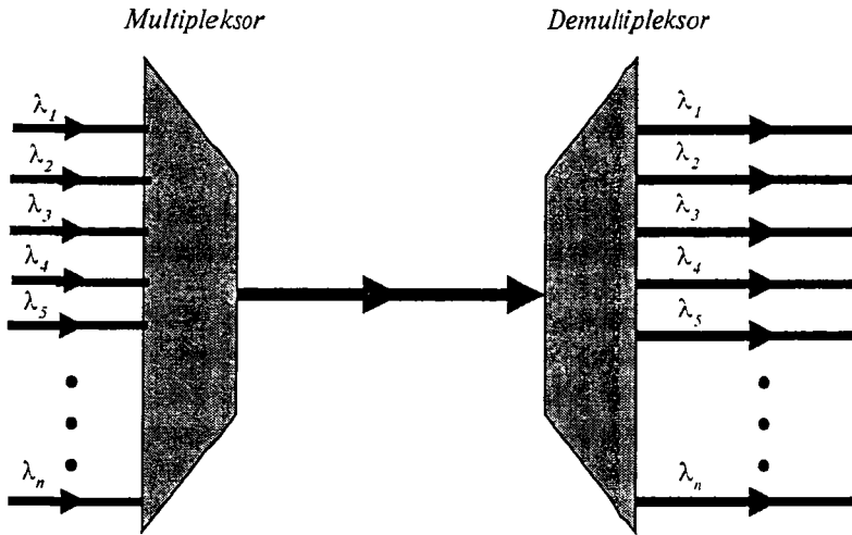
9.1-rasm. Spekttr bo'yicha zichlashtirilgan tolali optik aloqa tizimlarida multiplekslash va demultiplekslash jarayonlari
