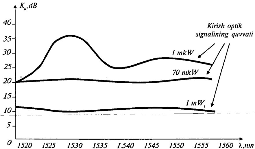
5.5-rasm. Erbiy aralashmali tolali optik kuchaytirgich kuchaytirish ko'effitsiyentining optik signal to'lqin uzunligiga bog'liqligi
