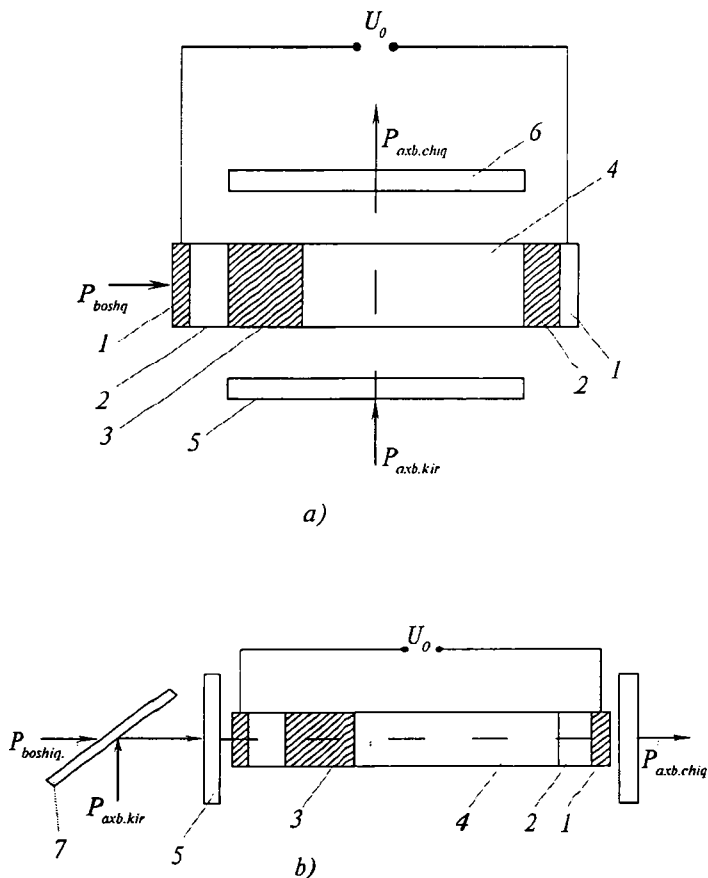
14.1-b rasm. Perpendikular turdagi (a) parallel turdagi (b) yorugʻlik bilan boshqariladigan qulfnig sxemasi
