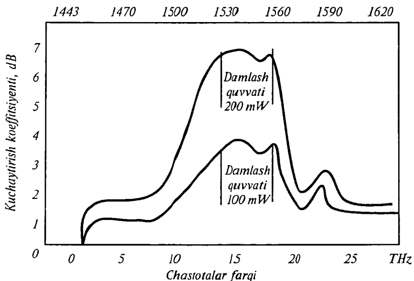
5.6-rasm. Raman kuchaytirgichning spektri
