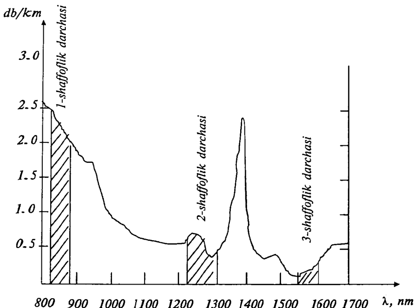
2.7-rasm. To‘lqin uzunligiga bog‘liq ravishda optik toladagi so‘nishning o‘zgarishi
