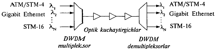
12.1-rasm. Oddiy ko'p to'liqli aloqa liniyasi
