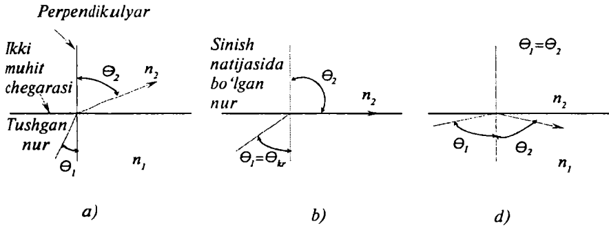
2.11-rasm. Bir necha tushish burchaklari uchun nurning tarqalish yo'li, n_1 > n_2 , bunda n_1 va n_2 ikki xilli muhitlarning sindirish ko'rsatkichlari
