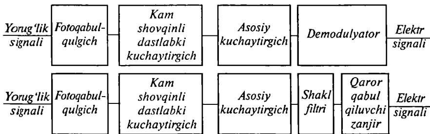
4.16-rasm. Analog (a) va raqamli (b) signallarni qabul qiluvchi optoelektron modulning tarkibiy funksional elementlari
