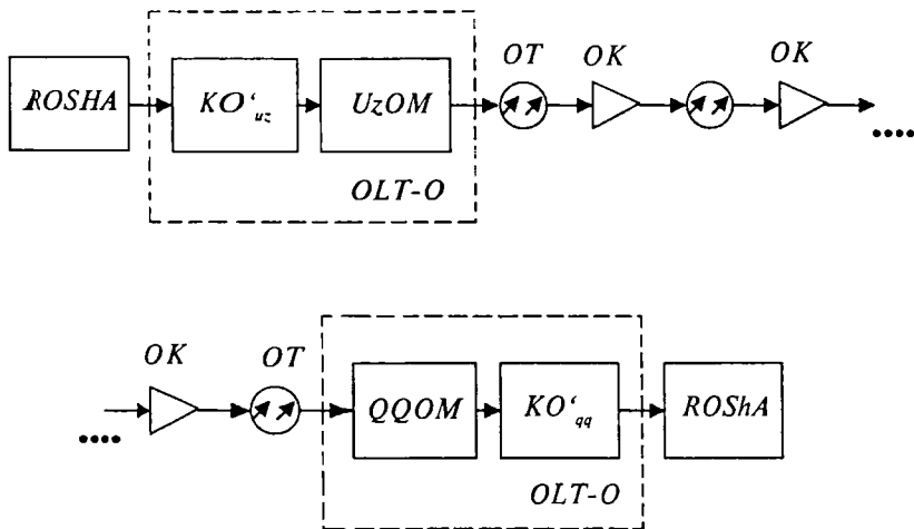
11.5-rasm. Raqamli TOATda optik kuchaytirgich (OK) qo'llanilgan optik liniya traktining umumlashgan tuzilish sxemasi
