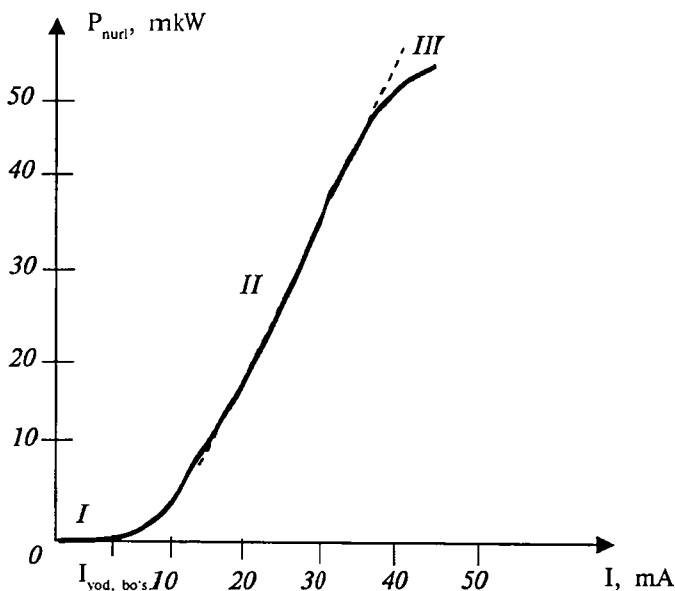
3.4-rasm. Yorug'lik diodining vatt-ampere xarakteristikasi
