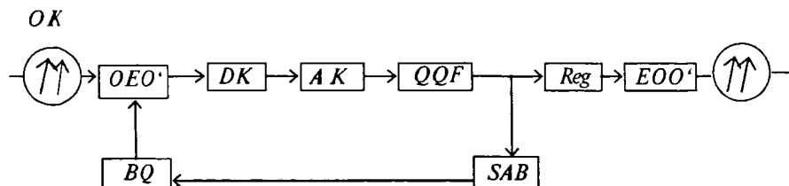
11.1-rasm. Raqamli retranslyator-regeneratorning umumlashgan tuzilish sxemasi
