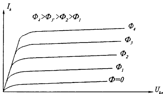
4.13-rasm. Bipolar fototranzistorning volt-amper xarakteristiklari oilasi
