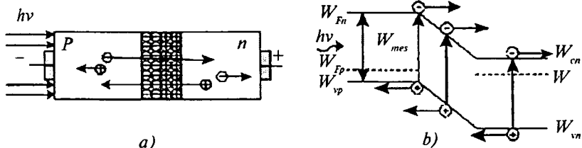
4.1-rasm. Fotodiodda tok hosil bo'lish jarayoni
