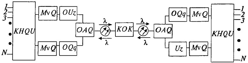
1.7-rasm. Bir tolali, bir polosali, bir kabelli TOAT sxemasi
