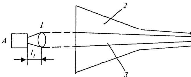
7.2-rasm. Nurlanish quvvatini optik tolaga kiritish qurilmasi: A – nurlanish manbai; 1 – sferik linza; 2 – konussimon tuzilishli bir modali optik tola; 3 – optik tolaning o‘zagi
