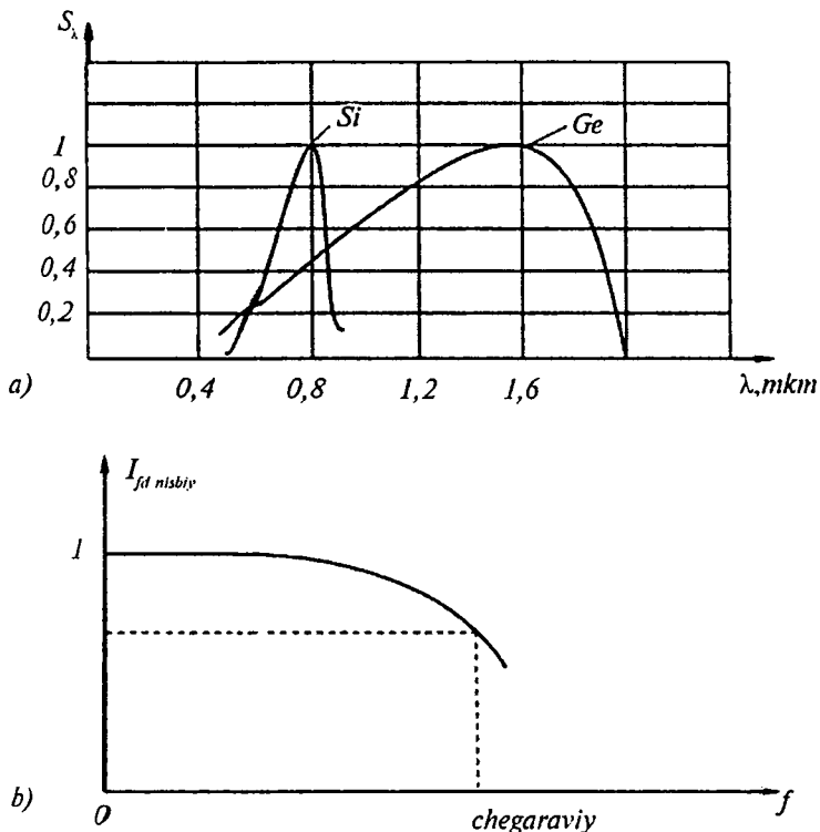
4.4-rasm. Fotodiodning spektral (a) va chastotaviy (b) xarakteristikalarini
