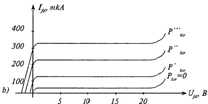
4.7-rasm. SP109 fotodiodining volt-farada (a) va volt-amper (b) xarakteristikalari
