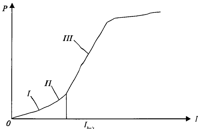
3.14-rasm. Yarimo'tkazgichli injeksion lazerning vatt-amper xarakteristikasi
