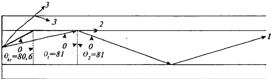
2.12-rasm. Optik tolada to'liq ichki qaytish jarayoni
