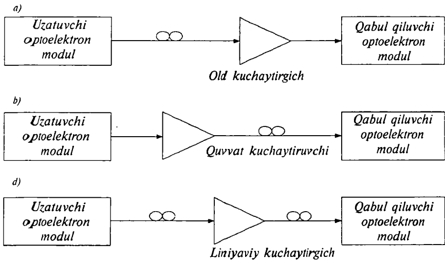
5.11-rasm. Optik kuchaytirgichlarning tolali uzatish tizimlarida qo'llanish usullari:
