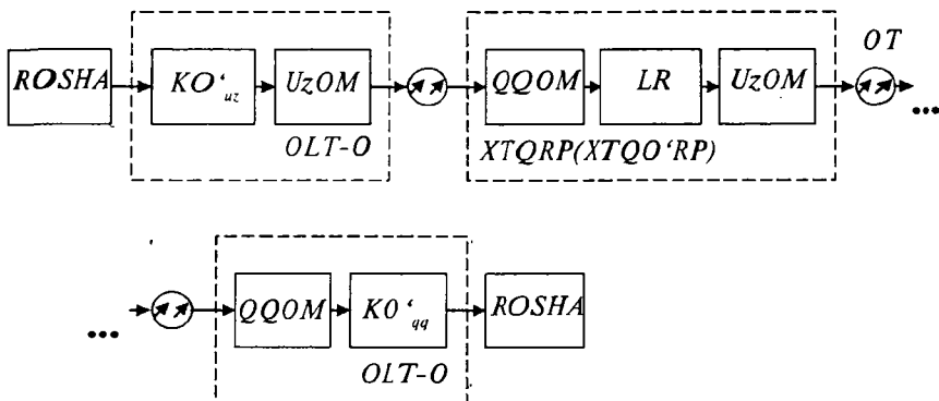
11.4-rasm. Raqamli TOATda regeneratord qo'llanilgan optik liniya traktining tuzilish sxemasi
