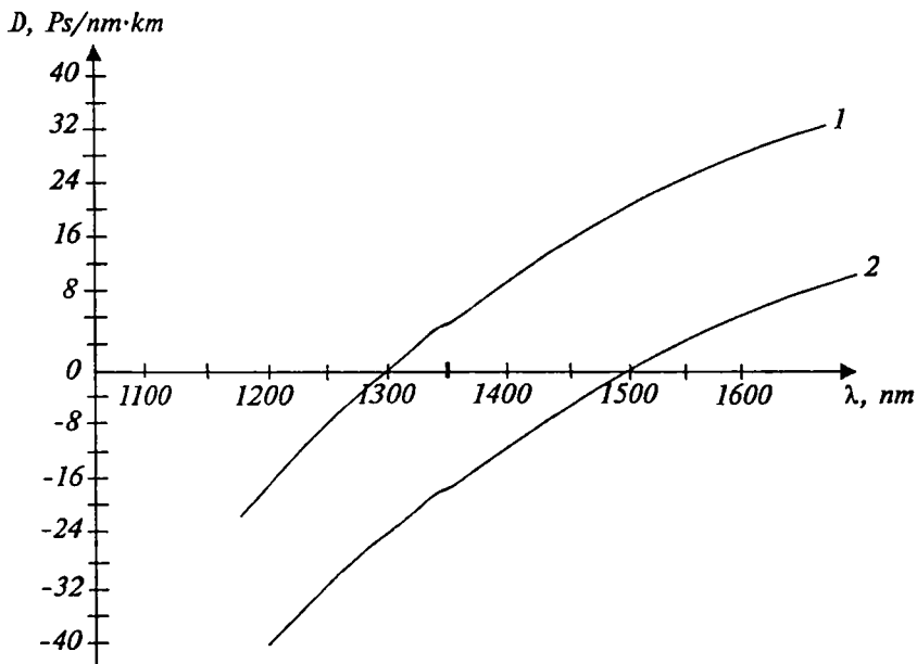
2.21- rasm. Xromatik dispersiyaning to‘lqin uzunligiga bog‘liqligi: 1 – toza kvarts shishasining xromatik dispersiya xarakteristikasi; 2 – siljigan dispersiyali tolaning xromatik dispersiya xarakteristikasi
