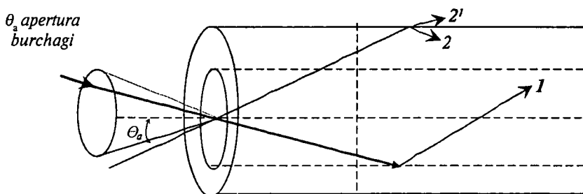
2.13-rasm. Optik tolaning apretura burchagi
