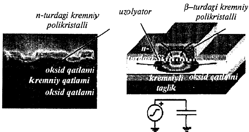
6.12-rasm. Kremniyli fazaviy optik modulya torning tuzilishi
