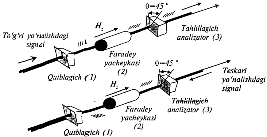
8.6-rasm. Optik izolatorning tuzilish sxemasi va ish prinsipi: a – toʻgʻri yoʻnalishdagi foydali optik signal undan toʻsiqlarsiz oʻtadi; b – teskari yoʻnalishdagi zararli signal qutblagich orqali oʻtmaydi
