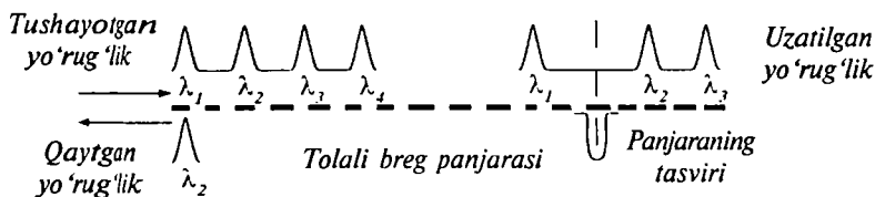
9.6-rasm. Totali bregg panjarasida guruhiy signaldan muayyan to'liqin uzunlikli kanalni ajratish jarayoni.
