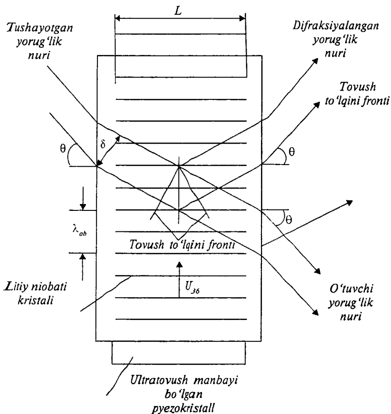
6.9-rasm. Yorug'lik nurining akustooptik modulyatordan o'tish sxemasi
