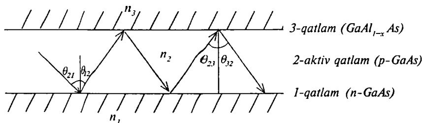
3.17-rasm. Geteroo'tishli tuzilmalarda to'liqin uzatish
