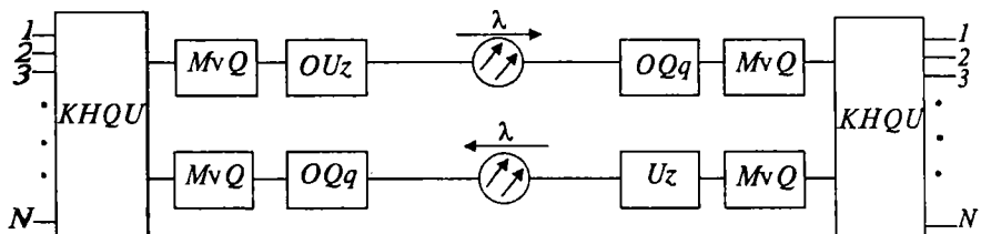
1.6-rasm. Ikki tolali bir polosali bir kabelli TOAT sxemasi
