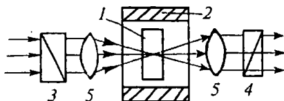
6.10- rasm. Magnitooptik modulyatorning tuzilish sxemasi:
