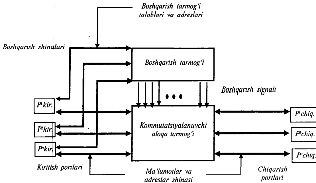
10.3-rasm. Köt li va markazlashgan boshqaruvli kommutatorning blok-sxemasi
