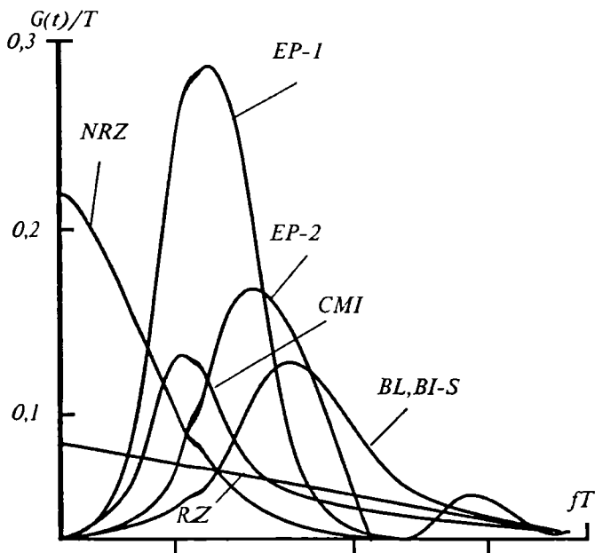
11.7-rasm. Raqamli TOAT energetik spektrining uzluksiz qismi
