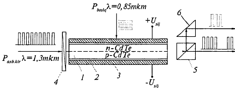
14.3-rasm. Yorug'lik bilan boshqariladigan fazoviy almashlab ulagichning tuzilish sxemasi
