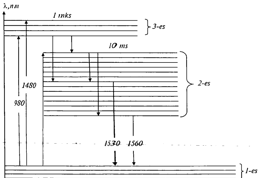
5.2-rasm. Kvars tolasi tarkibidagi erbiy ionlari ( Er^{+3} )ning energetik sathlari majmuasi
