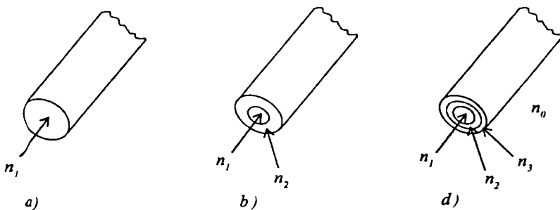
2.1-rasm. Yorug'lik uzatuvchi optik tolalar
