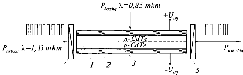
14.2-rasm. Qutblanuvchi kommutatordan foydalanishga asoslangan yorug‘lik bilan boshqariluvchi qulfnng sxematik tuzilishi [1]
