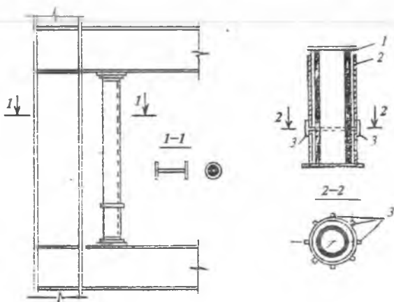
9.8-rasm. Oldindan zo'riqtirilgan tirkak bilan kuchaytirish.
