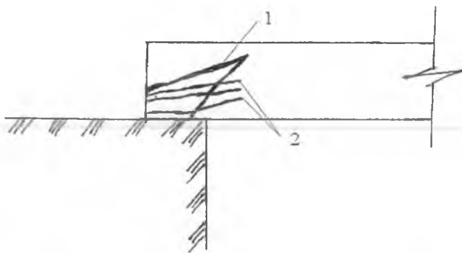
6.2-rasm. Oldindan zo'riqtirilgan elementning tayanch qismidagi darzlar. 1 – zo'riqtirilgan armaturadagi ankerovka buzilganda. 2 – siqilish kuchlanishi ta'sirida kesimdagi qiya armatura yetarli bo'lmagan holda.
