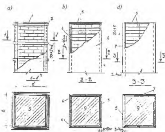
9.3-rasm. Tosh stolblarni kuchaytirish: po'lat (a), temir-beton (b), armaturalangan qorishmali halqa (d) bilan kuchaytirish.
