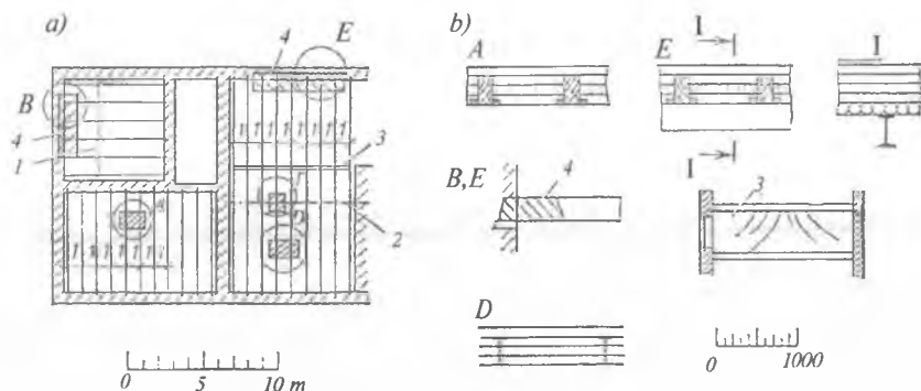
3.4-rasm. Orayopmalarni tekshirishga oid chizma sxemasi:
