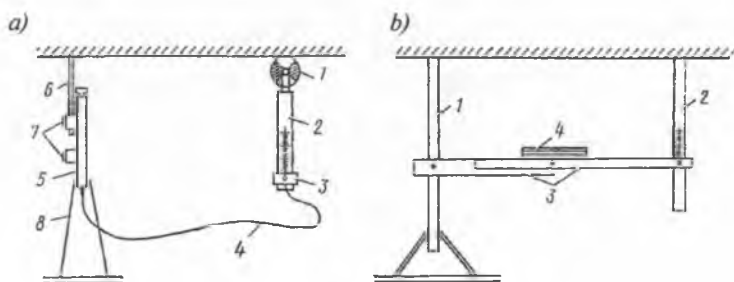
3.7-rasm. Solqilarni oʻlchash uchun asboblari:
