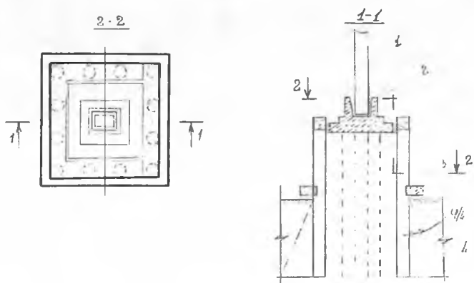
8.1-rasm. Zaminlarni to'siqli svaylar bilan kuchaytirish.
