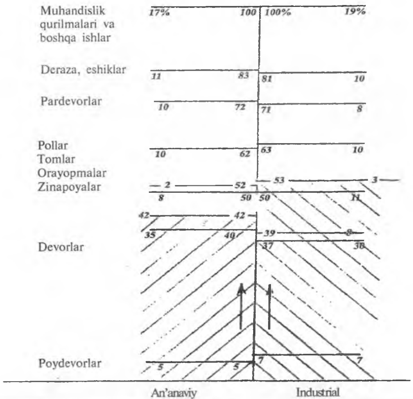
1.20-rasm. Binoning konstruktiv elementlarining solishtirma og'irligi. Almashtirilmaydigan konstruksiyalar sxrix bilan ko'rsatilgan.
