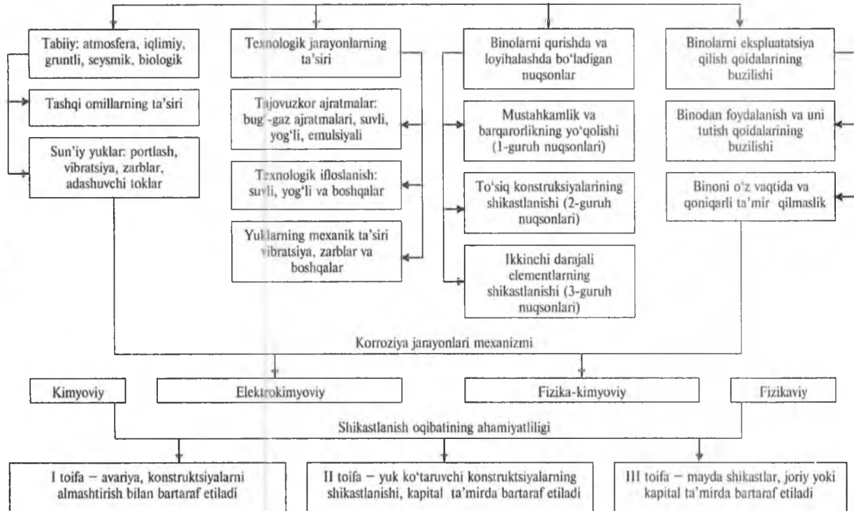
5.1-rasm. Shikastlanishni keltirib chiqaruvchi sabablar.
