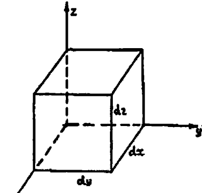
1-chizma. Uch o'lchamli Dekart koordinat sistemasi uchun dV = dx dy dz
