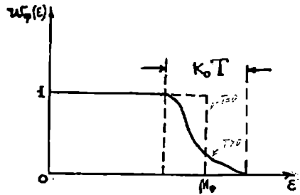
13 - chizma. Fermi-Dirak taqsimotining energiyaga bog'liqlik grafiqi
