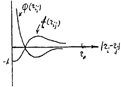
7-chizma. O'zaro ta'sir potentsial energiyasi f(r_{ij}) va f(r_{ij}) -funksiyalarining zarralar orasidagi masofaga bog'liqligi
