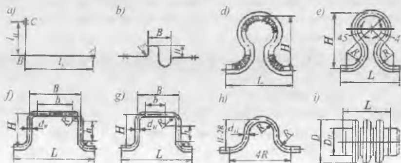
17-rasm. Kompensator qurilmalarning turlari:
