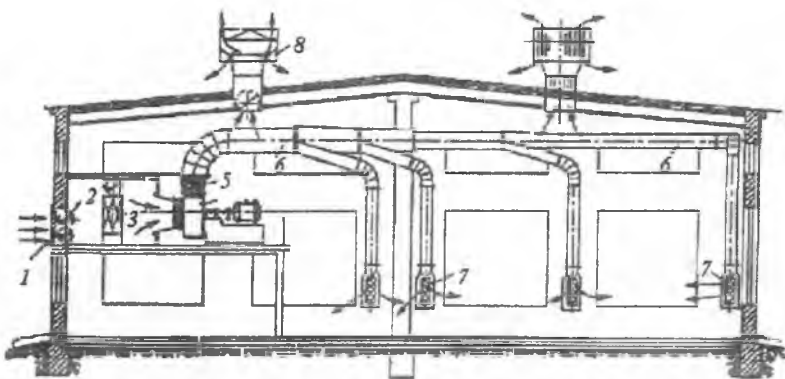
35-rasm. Sanoat binolarining oqib kelish va so'rib chiqarish umum almashtiruv ventilatsiyasi:
