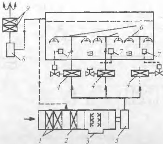
47-rasm. Ko'p zonali to'g'ri oqimli HKT: shartli belgilar 45-rasm bo'yicha.
