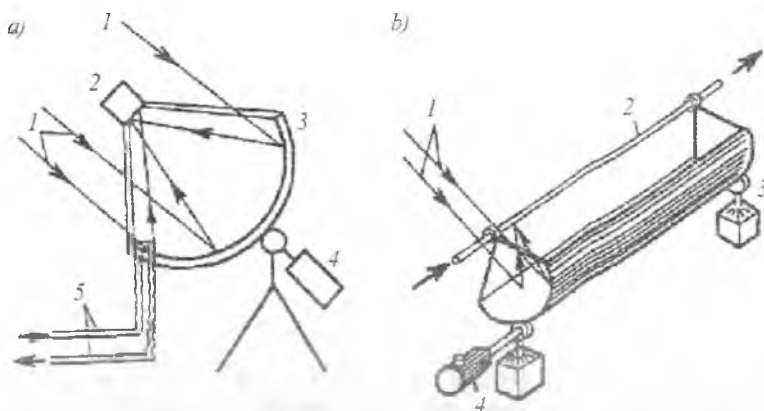
28-rasm. Konsentratsiyalaydigan quyosh kollektorlari:
