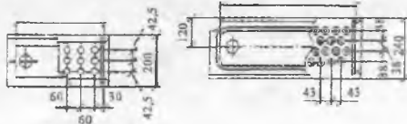
37-rasm. Bir yo'nalishli spiralsimon o'rnanagan kalorifer.
