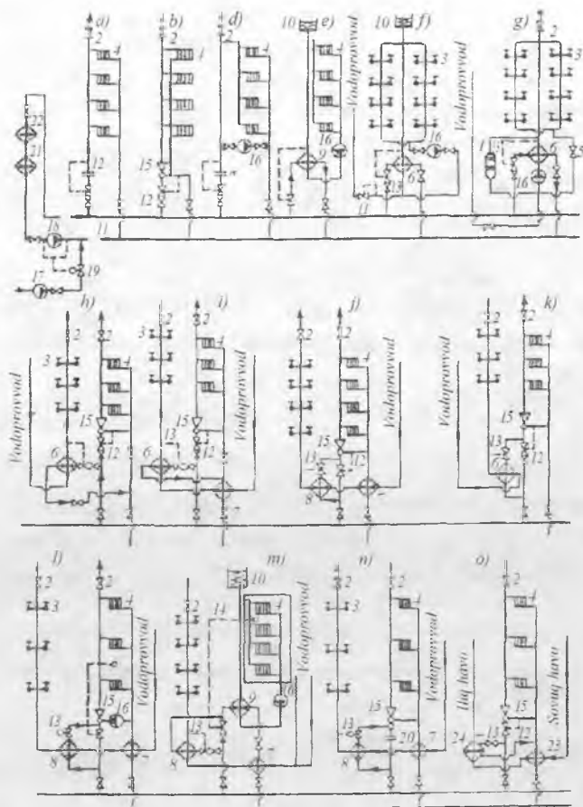
5-rasm. Issiqlik ta'minotining suvli ikki quvurli yopiq tizimi:
