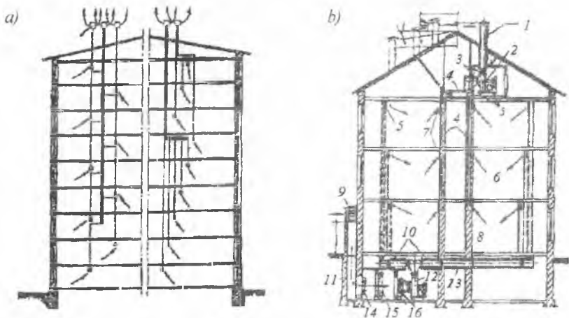
33-rasm. Ko'p qavatli turar joy va jamoat binolarini tabiiy (I) va sun'iy (II) ventilatsiya chizmalari:
