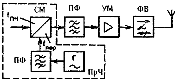
Рис. 1. Структурная схема передатчика БРТР
