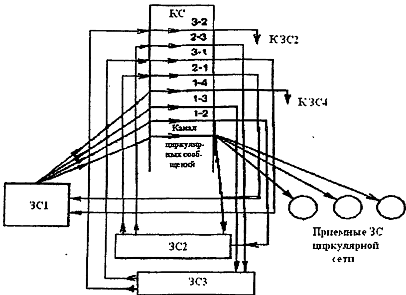
Рис. 1. Схема организации циркулярных и дуплексных каналов через ИСЗ
