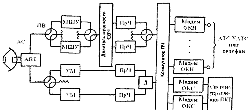
Рис. 6. Функциональная схема ЦУС/ЦЗС телефонной сети VSAT
