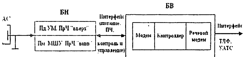
Рис.5. Функциональная схема станции VSAT-ТЛФ
