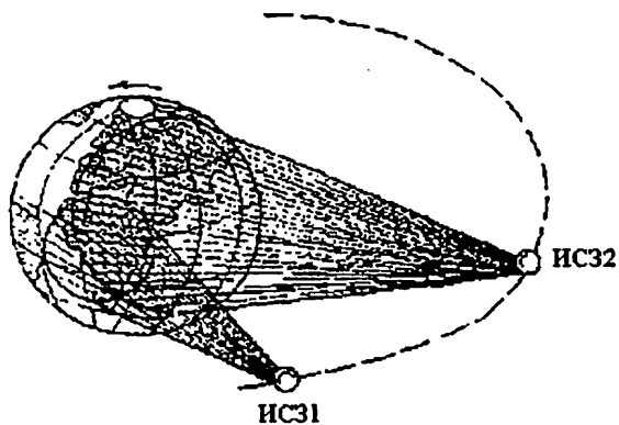
Рис. 2. К определению зоны обслуживания системы спутниковой связи с несколькими ИСЗ
