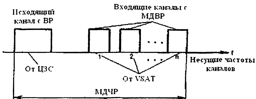
Рис. 4. Многостанционный доступ в сетях VSAT типа «звезда»
