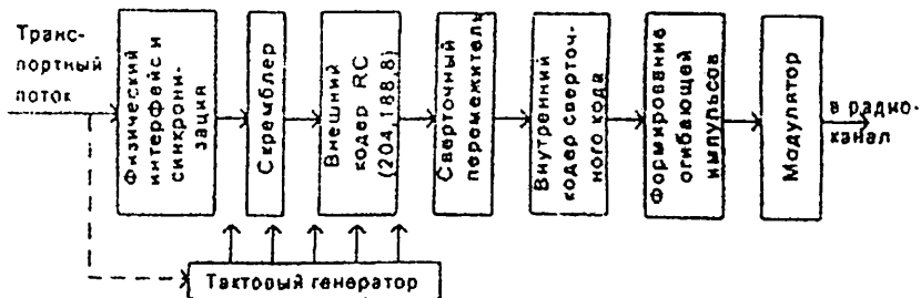
Рис. 1. Последовательность этапов обработки сигналов в спутниковом ТВ вещании
