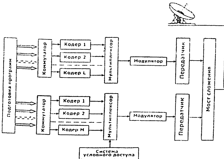
Рис. 2. Структурная схема передающей части системы цифрового вещания
