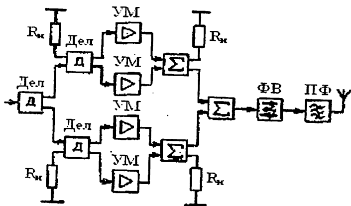
Рис. 2. Схема сложения мощностей четных усилителей
