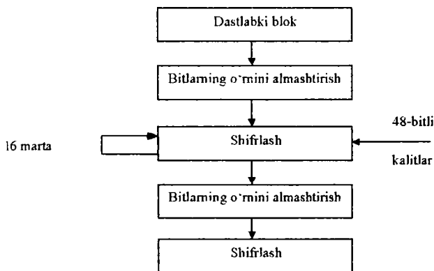
5.11- rasm. DES algoritmidagi shifrlash jarayonining blok-sxemasi.
