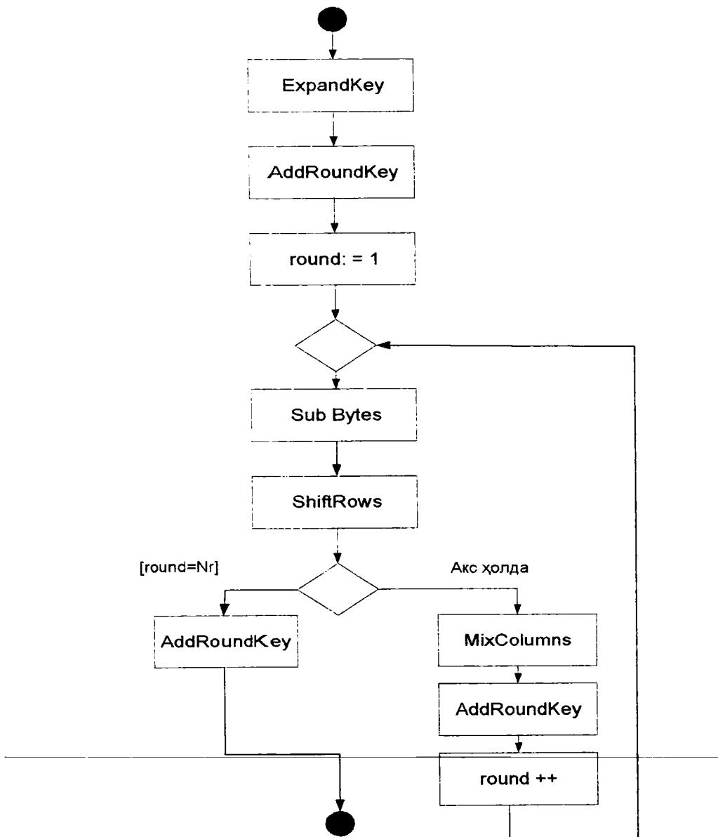
5.12–rasm. Shifrlash jarayoni.
