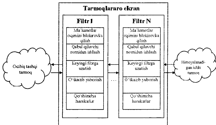
8.2-rasm. Tarmoqlararo ekran tuzilmasi.
