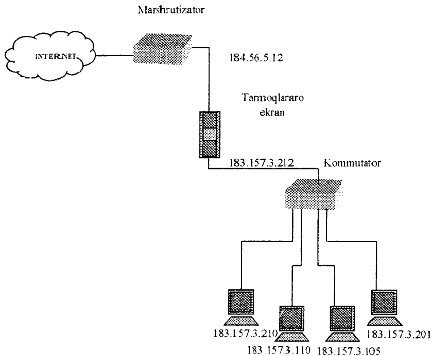
8.4-rasm. Tarmoq adreslarini translatsiyalash.
