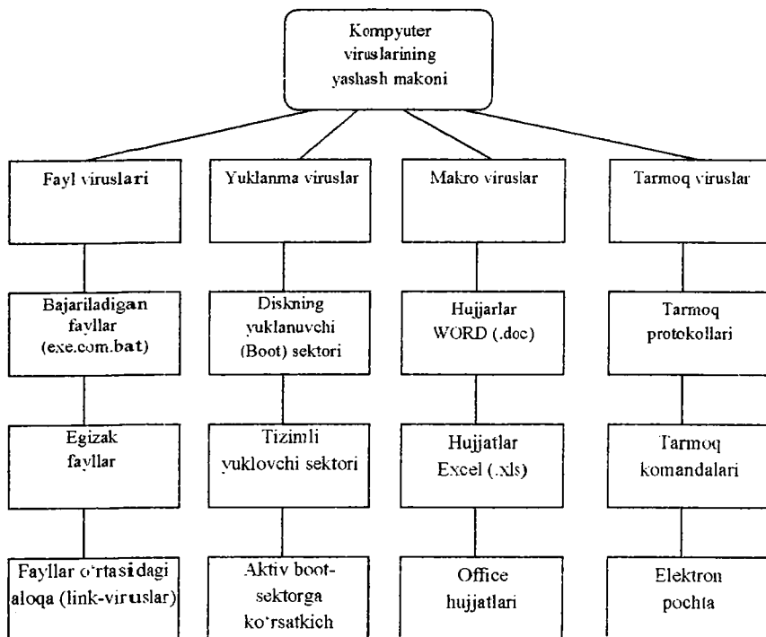
7.1-rasm. Yashash makoni bo'yicha kompyuter viruslarining turkumlanishi.
