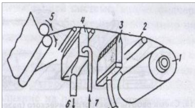
3.11-расм. Электростатик босма ускунанинг ишлаш чизмаси.
