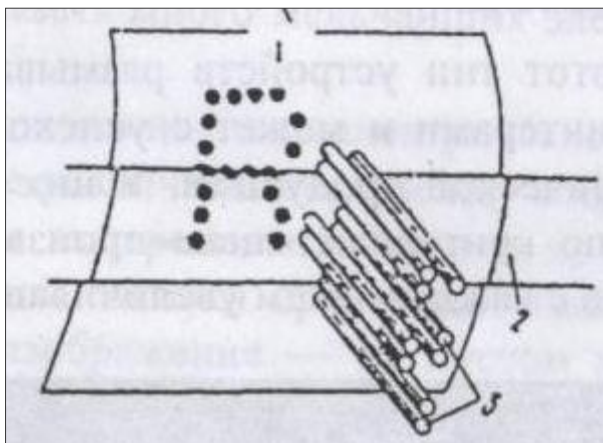
3.10-расм. Мозаикали (матрицали) принтернинг ишлаш принципи 1-қоғоз, 2-бўёқни узатувчи тасма, 3-игна
