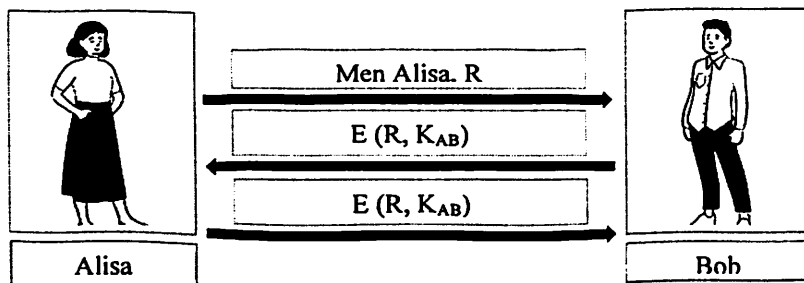
6.13-rasm. Ikki tomonlama autentifikatsiyami
