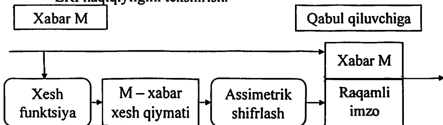
5.1- rasm. Elektron raqamli imzoni shakllantirish jarayoni
