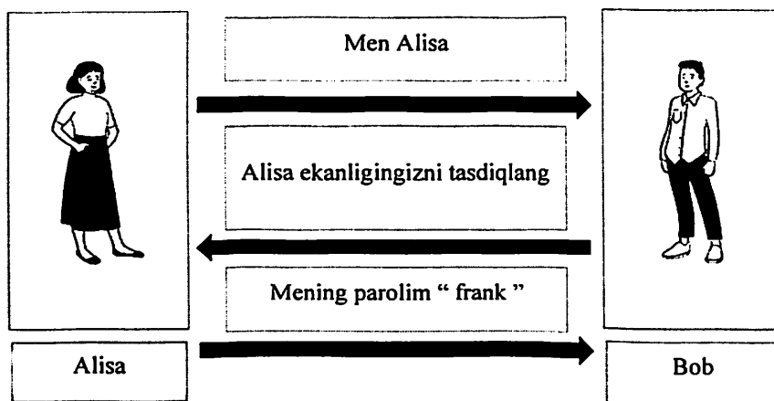
6.7-rasm. Sodda autentifikatsiya protokoli
