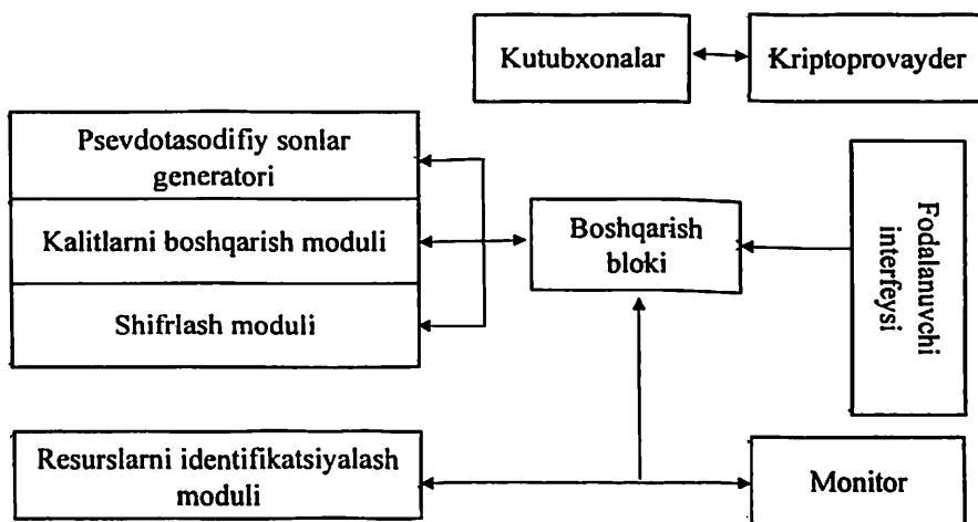
6.5-rasm. Kriptografik dasturiy vositalarning umumiy sxemasi
