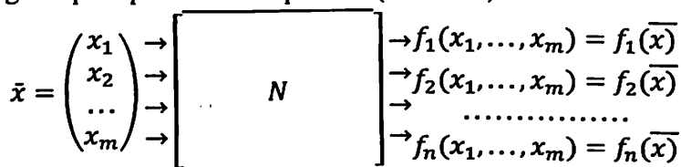
6.4-rasm. Nazariy kriptografiyada protokol sxemasi
