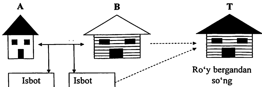
6.2-rasm. Arbitrli protokol
