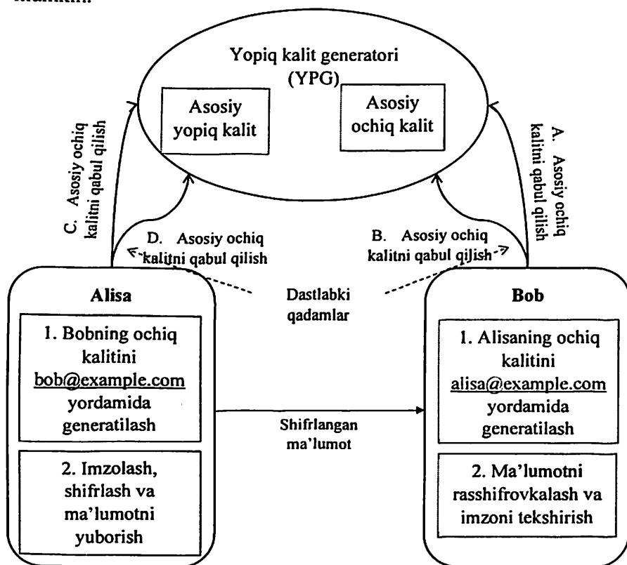
6.21-rasm. Identifikatorga asoslangan shifrlash algoritmining sxemasi
