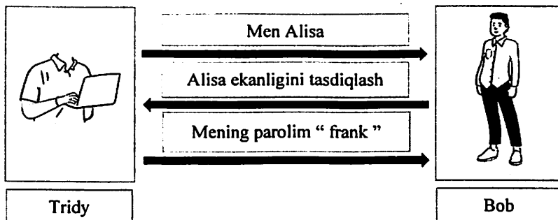
6.8-rasm. Takrorlash hujumi
