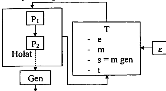
3.4-rasm. /dev/random ning umumiy strukturasi
