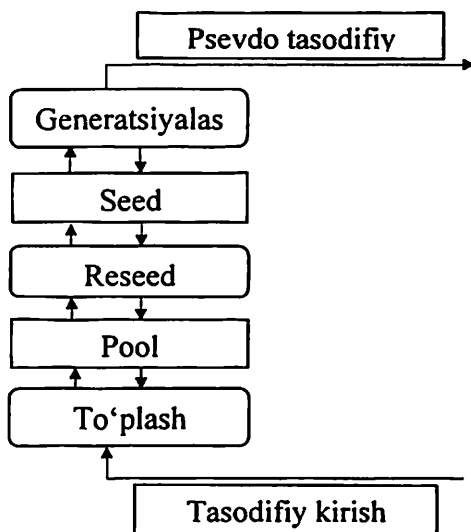
3.3-rasm. Umumiy KPTSG, doimiy ichki holatni yangilab borish jarayoni
