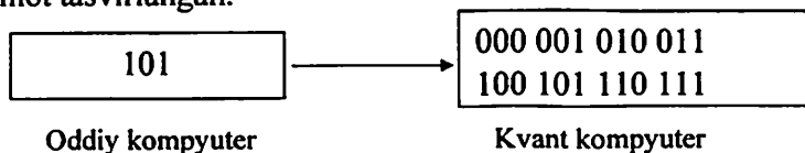
8.12-rasm. Oddiy va kvant kompyuterlarning registridagi maʼlumot
