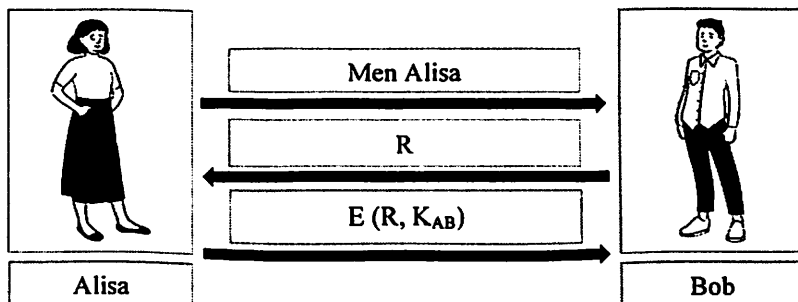
6.12-rasm. Simmetrik kalit asosida autentifikatsiya protokoli
