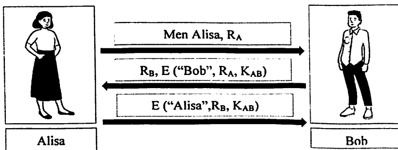
6.16-rasm. Bardoshli ikki tomonlama autentifikatsiyalash protokoli
