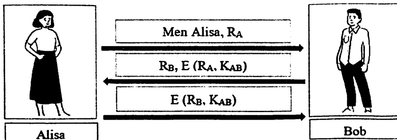
6.14-rasm. Xavfsiz ikki tomonlama autentifikatsiya
