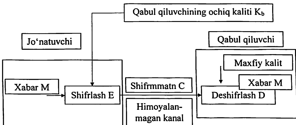
4.1 - rasm. Assimetrik shifrlash usullarining umumiy ko'rinishi
