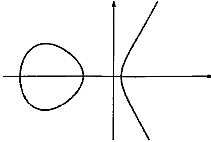
1.7-rasm. (1.5) tenglik grafigi
