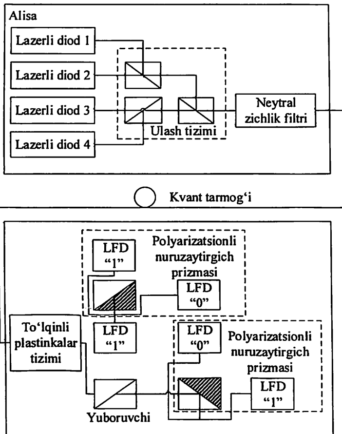
8.11-rasm. Polyarizatsiyalri kodlash tizim tuzilmasi
