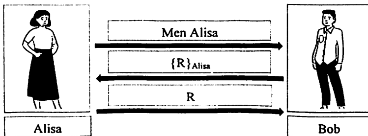
6.17-rasm. Ochiq kalit asosida autentifikatsiyalash
