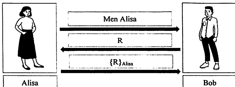
6.18-rasm. Raqamli imzo orqali autentifikatsiyalash
