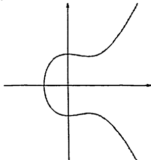
1.5-rasm. y^2 = x^3 + ax^2 + bx + c funksiya grafigi
