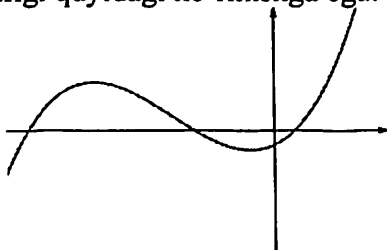
1.6-rasm. b holat uchun funksiya grafigi
