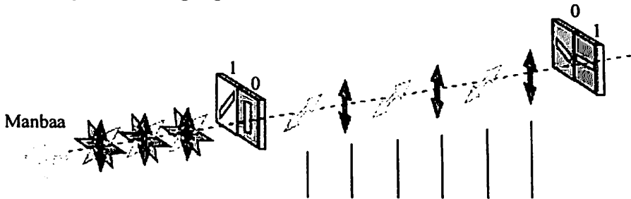
8.7-rasm. B92 protokolidagi polarizatsiya holatlari
