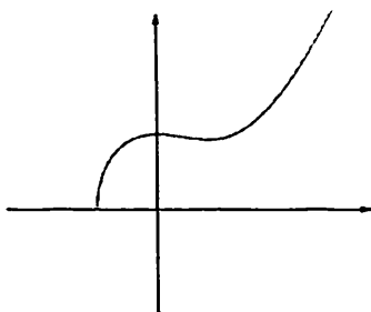
1.4-rasm. y = \sqrt{x^3 + ax^2 + bx + c} funksiya grafigi
