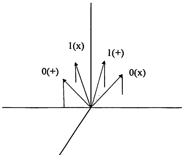
8.1-rasm. BB84 protokolidagi fotonlarning polyarizatsiya holati
