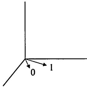
8.7-rasm. B92 protokolidagi polarizatsiya holatlari
