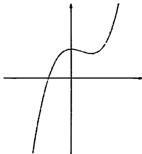
1.3-rasm. a holat uchun funksiya grafigi
