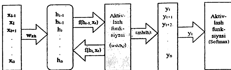
4.2.15-rasm. Recurrent neyron tarmoq arxitekturasi
