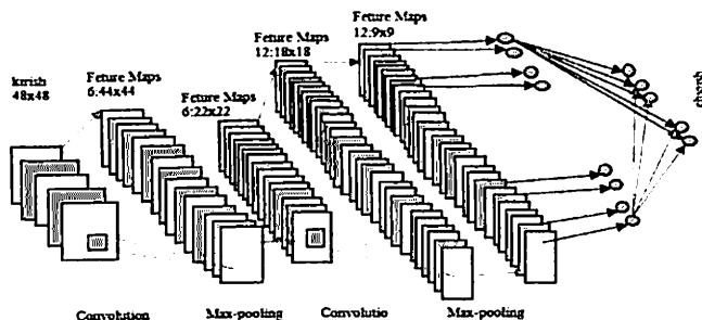
4.2.4- rasm. CNN arxitekturasi
