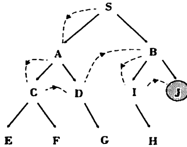
2.2.14-rasm. Chuqurlik bilan cheklangan qidiruv
