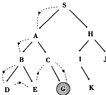
2.2.13-rasm. Chuqurlikdagi birinchi qidiruv
