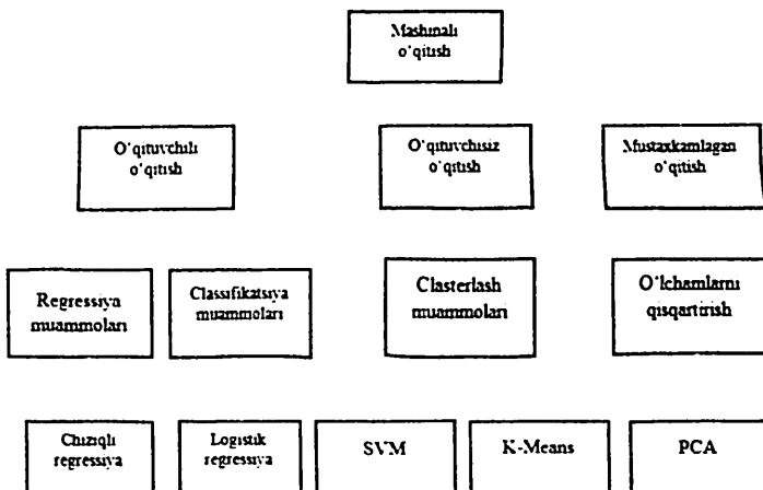
3.1.1- rasm. Mashinali o'qitish usullari
