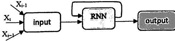
4.2.16- rasm. Recurrent neyronning yadro qatlami arxitekturası
