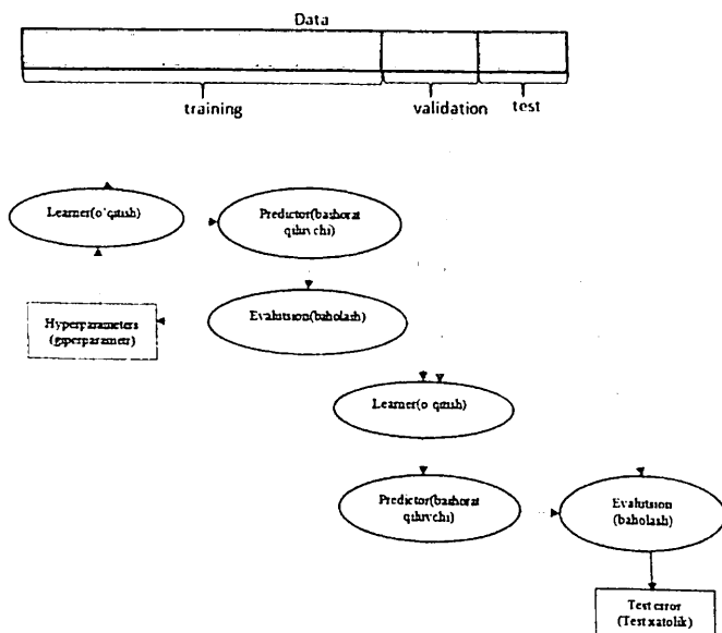
3.1.3-rasm. Modelni o'qitish va testlash jarayoni
