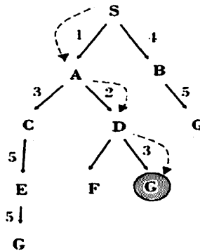
2.2.16-rasm. Yagona xatolikni qidirish strukturasi
