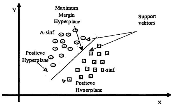
3.2.13-rasm. SVM qaror chegarasi va geparplan
