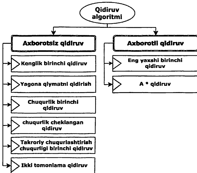
2.2.11-rasm. Axborotsiz va axborotli qidiruv algoritmlari strukturasi
