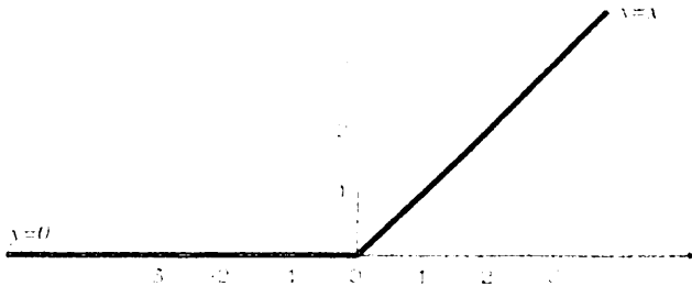
4.2.2-rasm. ReLU aktivlash funksiyasining grafik ko'rinishi
