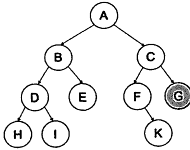
2.2.15-rasm. Chuqurlik bo'yicha qidiruv
