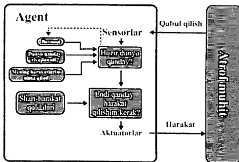
2.1.4-rasm. Modelga asoslangan refleks agent strukturasi
