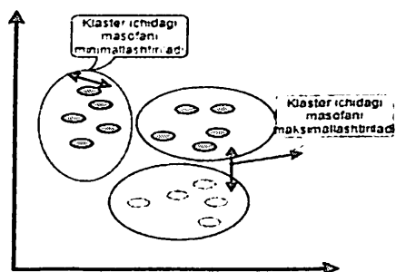
2.2.6-rasm. Klasterlash
