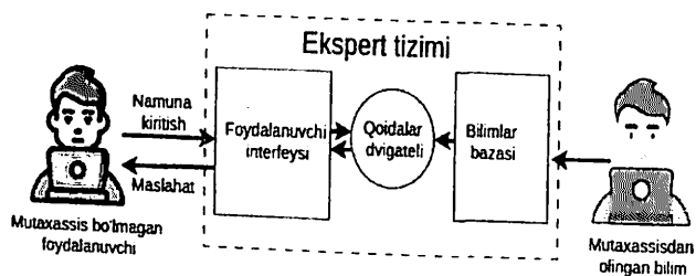
3.4.1-rasm. Expert tizimlari strukturasi
