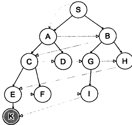
2.2.12-rasm. Kenglik-birinchi qidiruv strukturasi
