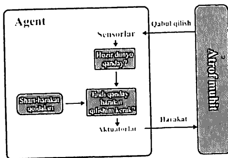
2.1.3-rasm. Oddiy refleks agent strukturasi
