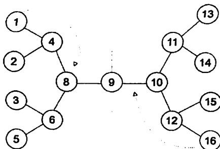
2.2.17-rasm. Ikki yo'nalishli qidiruv algoritmalmas
