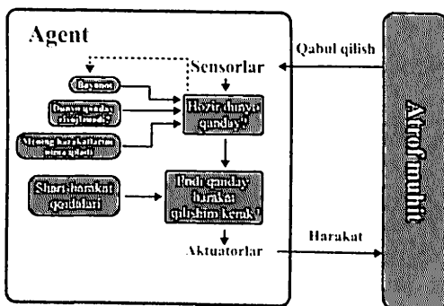
2.1.5-rasm. Maqsadga asoslangan refleks agent strukturasi
