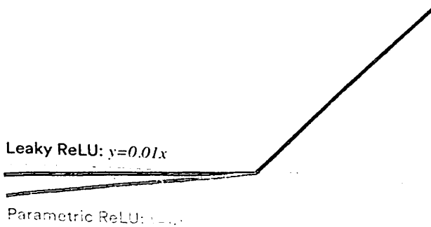
4.2.3-rasm. Leaky ReLU va Parametrik ReLU (PReLU) aktivlash funksiyasining grafik ko'rinishi
