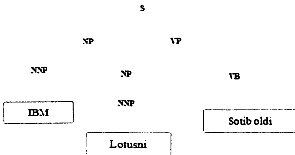
4.3.4-rasm. Sintaktik analizator gaplarni nodeterministik tahlil qilish yuqoridan pastga algoritmi
