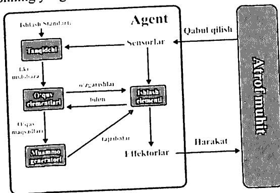
2.1.7-rasm. O'quv agentlariga asoslangan refleks agent strukturasi
