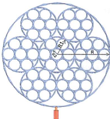
3.16-rasm. A2 eksklyuziv antenaning modeli
