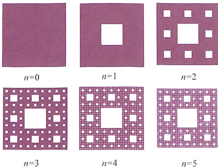
3.10-rasm. Kvadratik Serpin gilamini qurish
