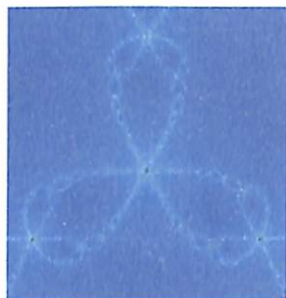
Nyuton fraktali
