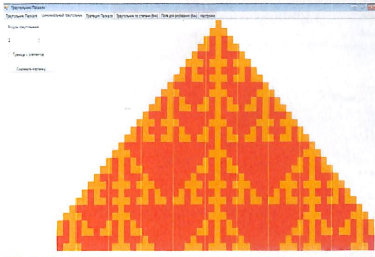
5.28-rasm. Trinomial uchburchak yorligʻi
