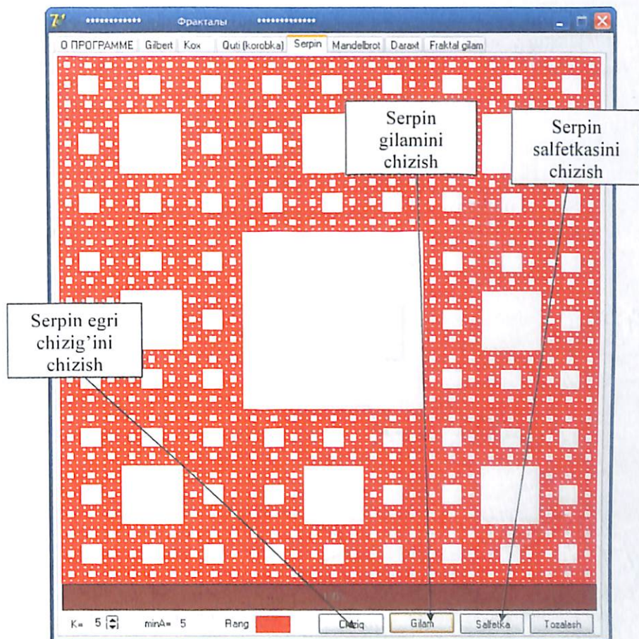
5.17-rasm. Serpin kvadrat gilami
