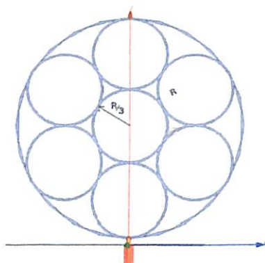
3.15-rasm. A1 eksklyuziv antenaning modeli
