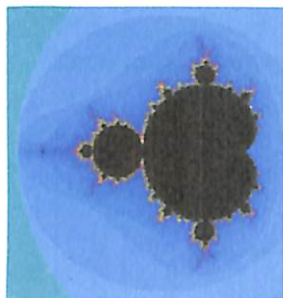
Mandelbrot fraktali
