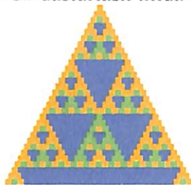
5.32-rasm. Paskal uchburchagi 3 moduli bo'yicha binomial koeffitsiyentlarning tarqalishi
