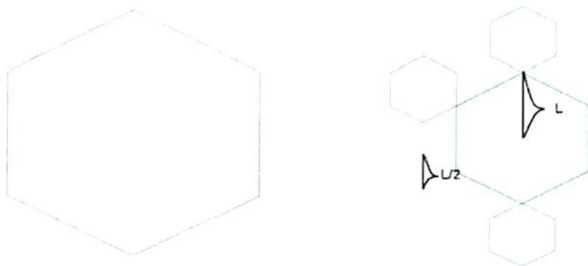
4.9-rasm. Oltiburchakli fraktallar, 1-qadam va 2-qadamda
