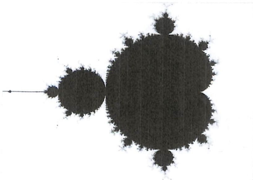
2.6-rasm. Mandelbrot to'plamining 200 marta kattalashtirilgan ko'rinishi
