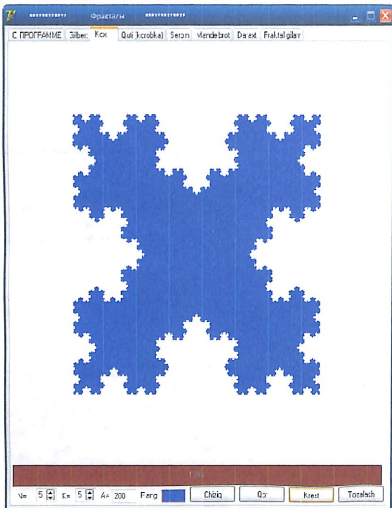
5.16-rasm. Kox krestik fraktali
