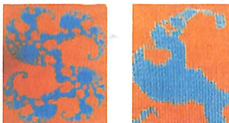
2.16-rasm. Juliya fraktali naqshining obyektidagi tasviri
