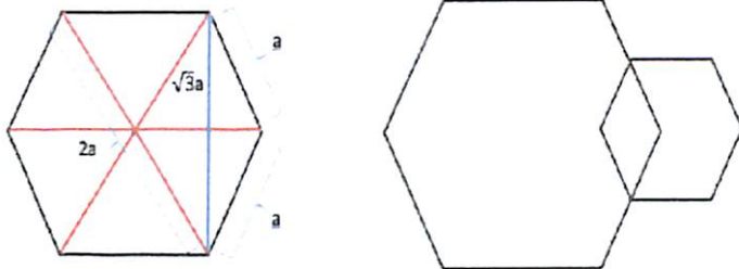
4.8-rasm. Oltiburchakli fraktallar, 1-qadam va 2-qadamda
