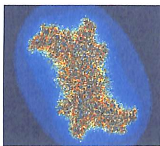
1.4-rasm. Stoxastik fraktallar
