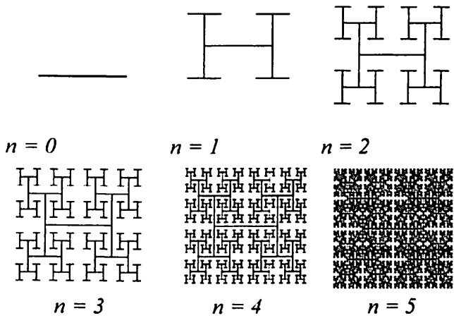
3.14-rasm. “Keyli daraxti”ga asoslangan fraktal
