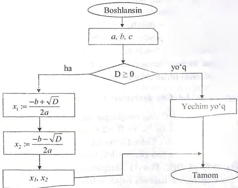
1-rasm. Kvadrat tenglama uchun blok-sxema.
