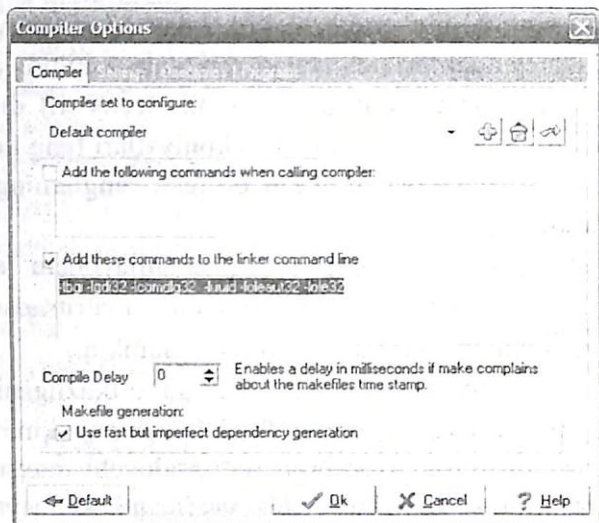
15-rasm. Muhitni grafik rejimga sozlash oynasi.
