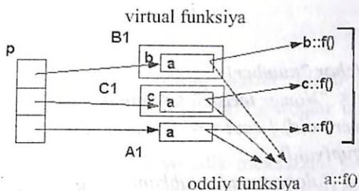
22-rasm. Virtual funksiya.
