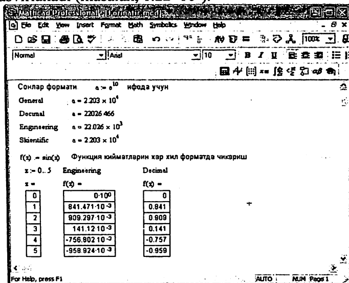
3.4-rasm. Sonlarni formatlash va qiymatlarni har xil formada tasvirlash.
