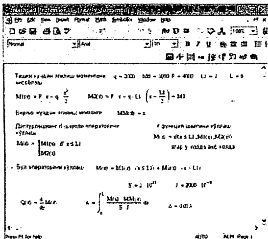
3.5.-rasm. Uzlukli funksiyalarni hisoblashda shartlarni ishlatish.
