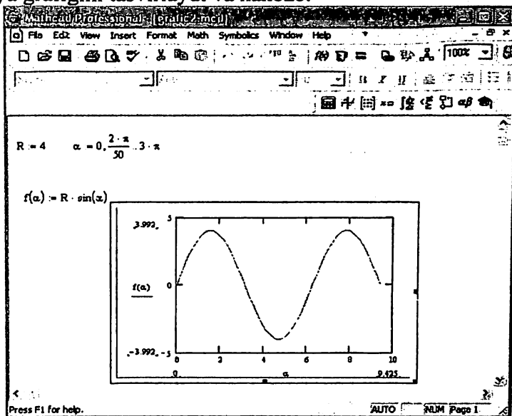
3.24.-rasm. Funksiya grafigini qurish.
