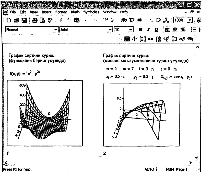
3.25.-rasm. Ikki o'zgaruvchili funktsiya grafiginini qurish.
