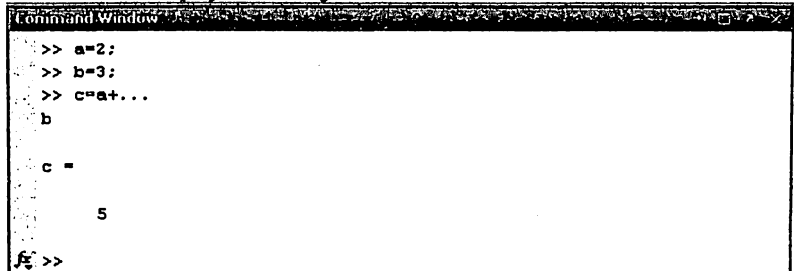
2.10 -rasm. Matematik ifoda.
