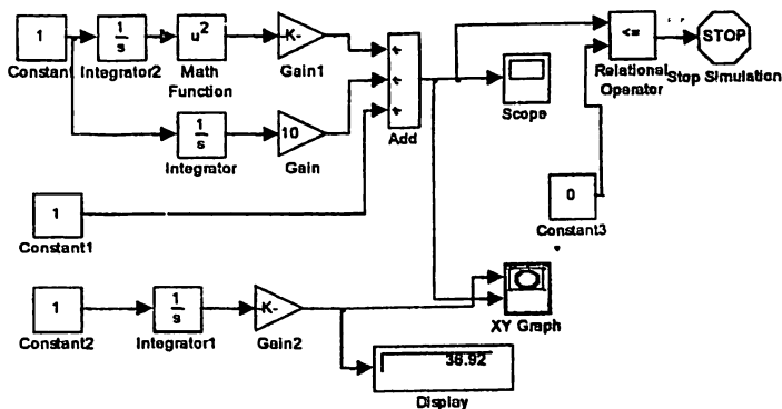
4.8 -rasm. Tosh trayektoriyasi modelining sxematik tuzilishi
