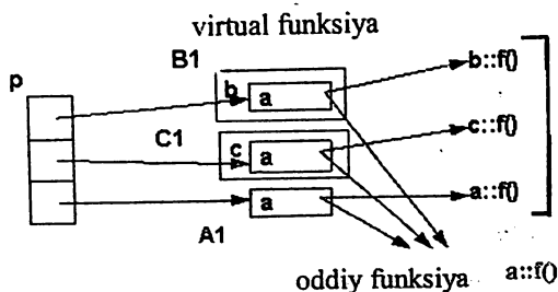
22-rasim. Virtual funksiya.
