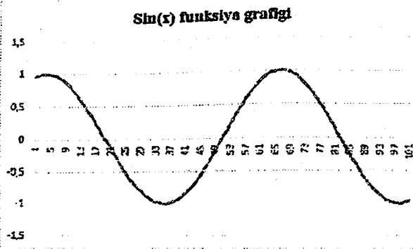
4.111-rasm. Sin(x) funksiya grafigi
