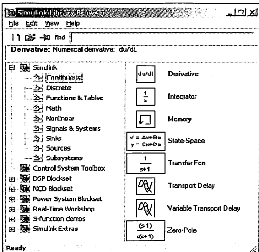
7.32-rasm. Kutubxona bo‘limlarining bloklerini terish oynasi
