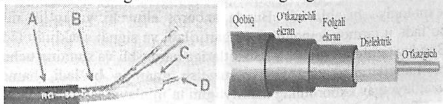
8.1-rasm. Koaksial kabel
