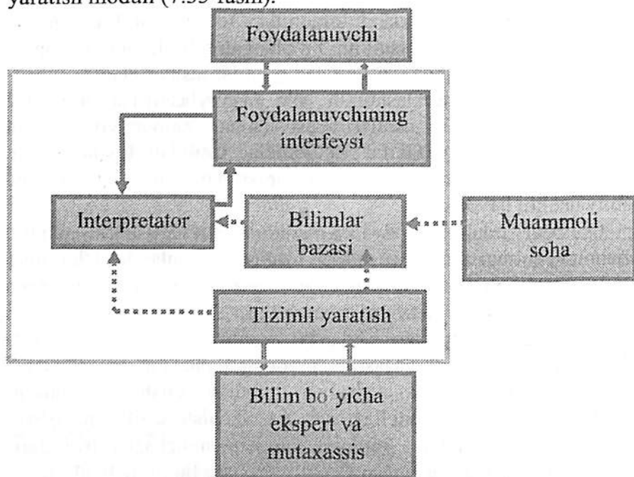
7.37 – rasm. Ekspert tizimining tarkibiy qismi
