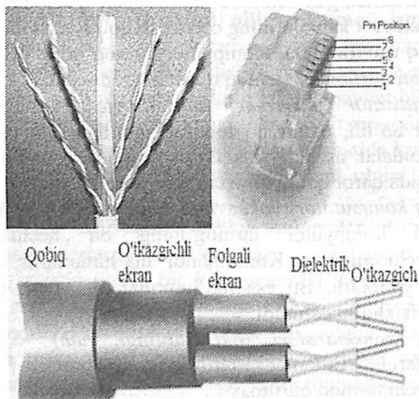
8.2-rasm. O'rama juft kabel
