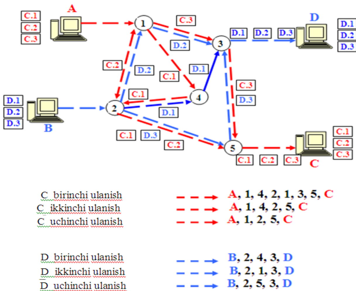
2.3 – rasm. Paketlarni tarmoqda har xil yo‘llar orqali uzatilishi
