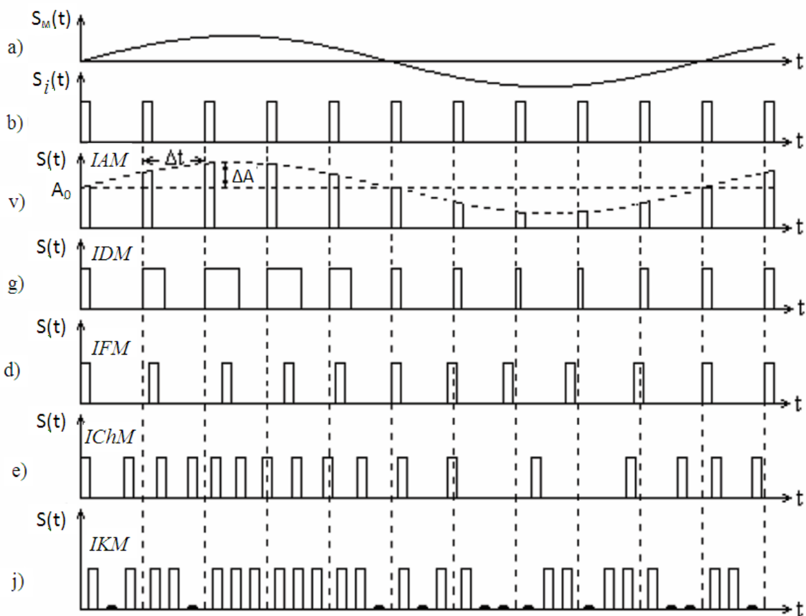
5.12-rasm. Turli parametrlari modulyatsiyalangan impulsar ketma-ketliklari vaqt diagrammalari
