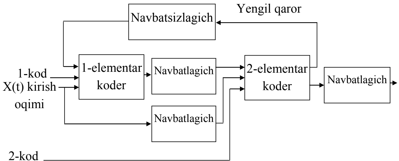
4.7-rasm. Ikkita elementar koderlardan tashkil topgan turbo dekoder sxemasi
