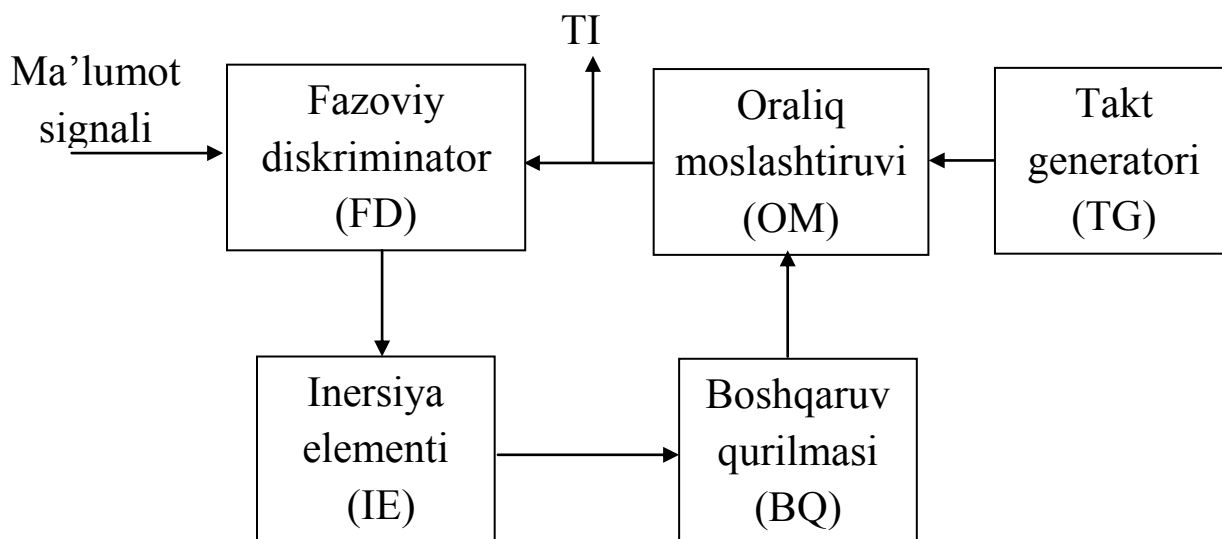
4.22-rasm. TG ga bevosita ta'sir ko'rsatuvchi qurilma
