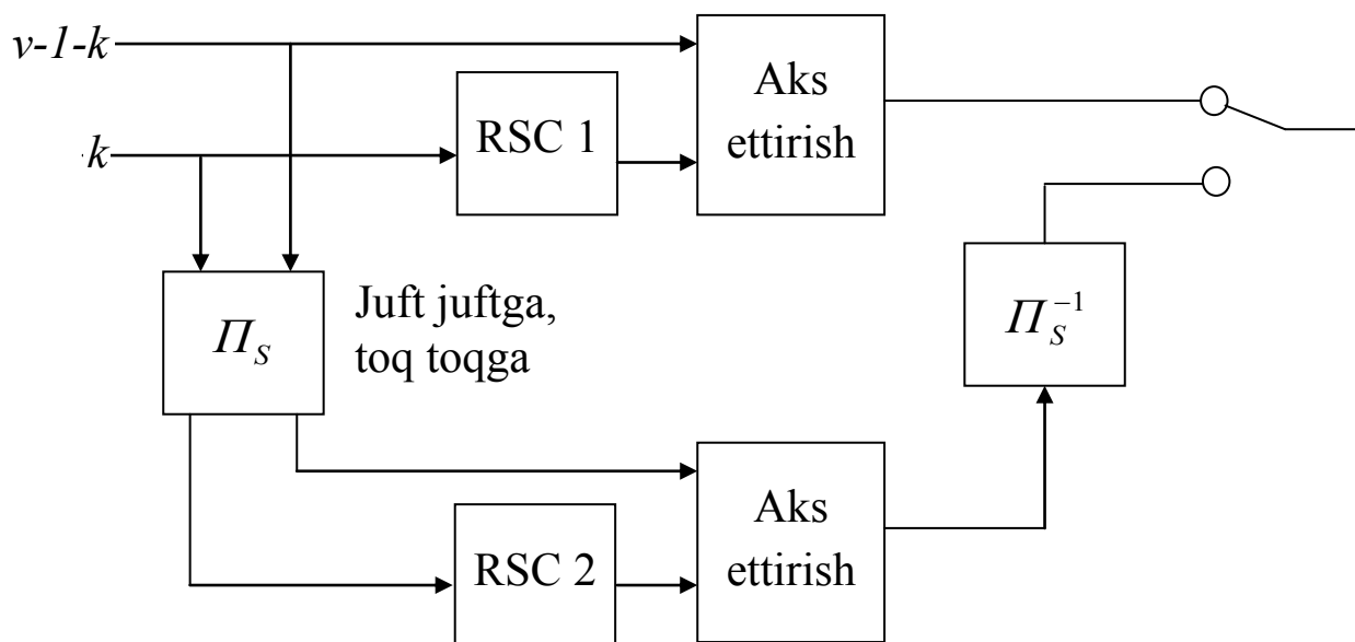
5.8-rasm. Simvulli aralashtirishda panjarada turbo kodli modulyatsiya koderining tuzilishi
