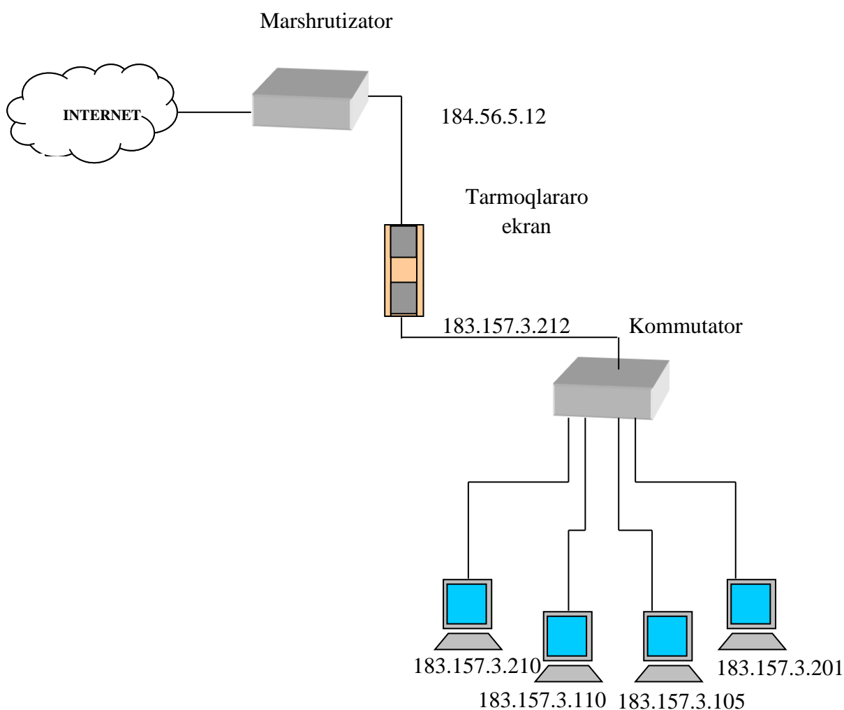
8.4–rasm. Tarmoq adreslarini translatsiyalash
