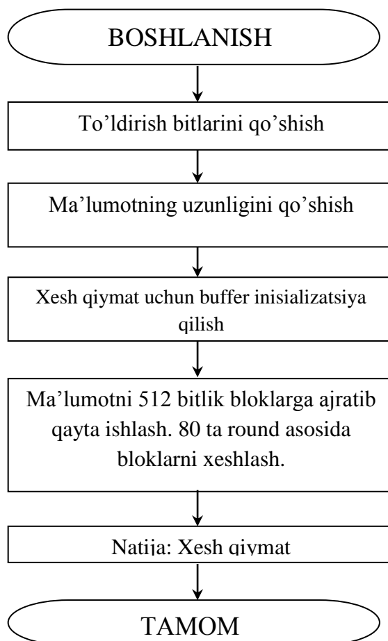
5.18-rasm. SHA1 algoritmi ishlash blok sxemasi
