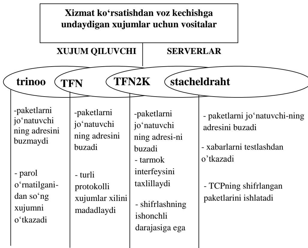
2.1-rasm. Xizmat qilishdan voz kechishga undaydigan xujum vositalarining xarakteristikalarini
