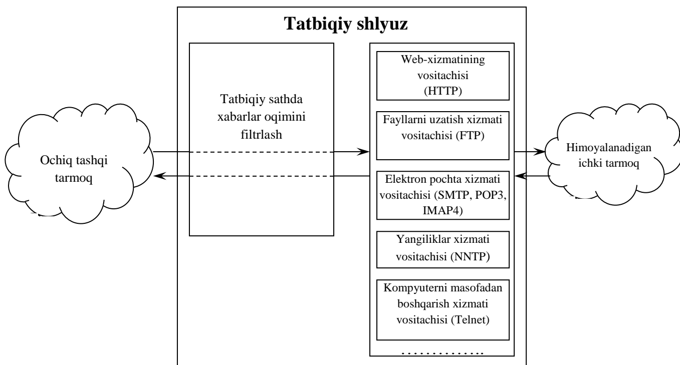
8.9-rasm. Tatbiqiy shlyuzning ishlash sxemasi.
