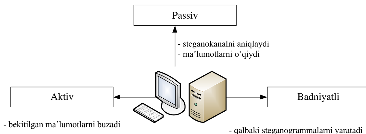
5.25-rasm. Steganografik tizimlarni buzuvchilar turi
