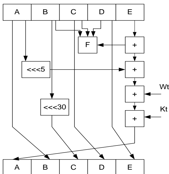
5.17-rasm. SHA-1 algoritmidagi bir iteratsiyasining sxemasi.
