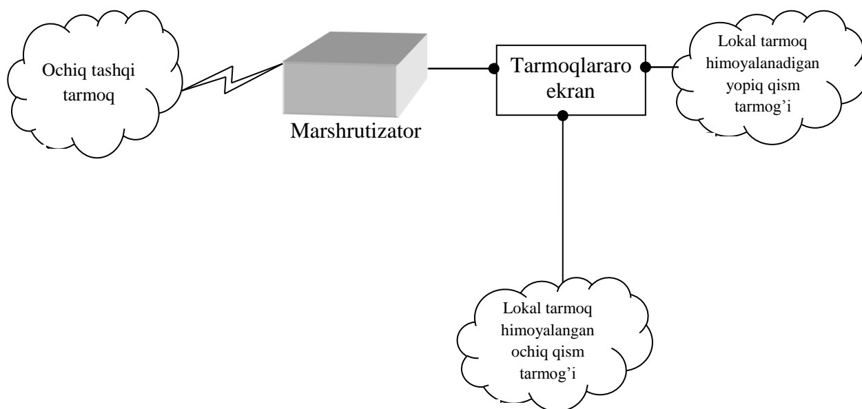
8.14 -rasm. Uchta tarmoq interfeysli bir brandmauer asosida yopiq va ochiq qismstarmoqlarni alohida himoyalash sxemasi
