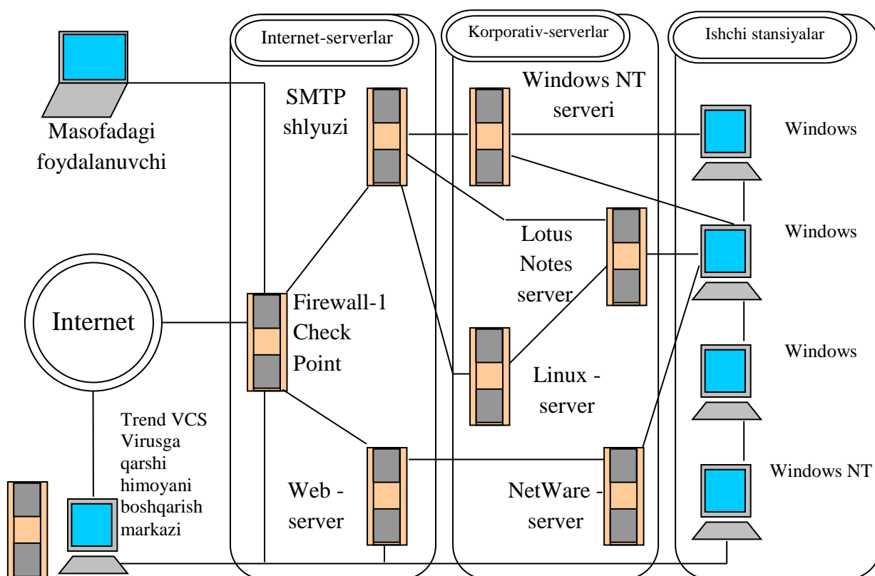
7.2–rasm. Korporativ tarmoqning namunaviy arxitekturasi
