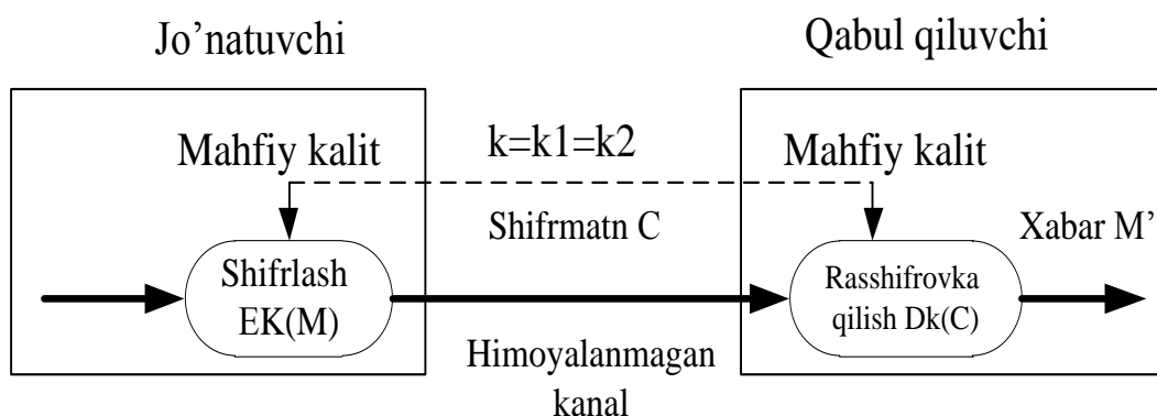
5.9-rasm. Simmetrik shifrlash kriptotizimining sxemasi.
