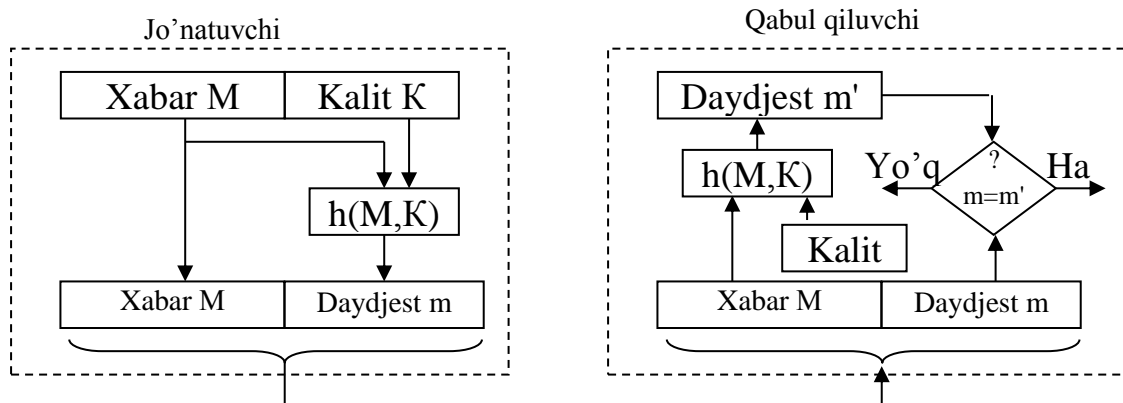
6.5–rasm. Ma'lumotlar yaxlitligini tekshirishda bir tomonlama xesh-funksiyaning ishlatilishi (II-variant).
