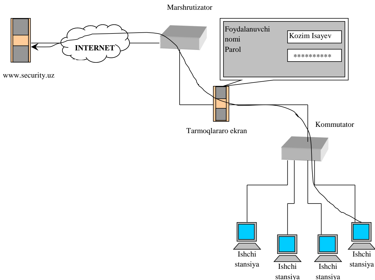
8.3–rasm. Parol bo'yicha foydalanuvchini autentifikatsiyalash sxemasi
