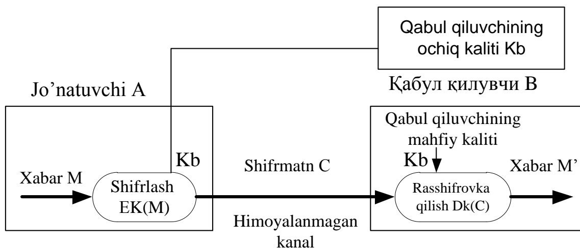
5.15-rasm. Asimmetrik shifrlashning umumlashtirilgan sxemasi.
