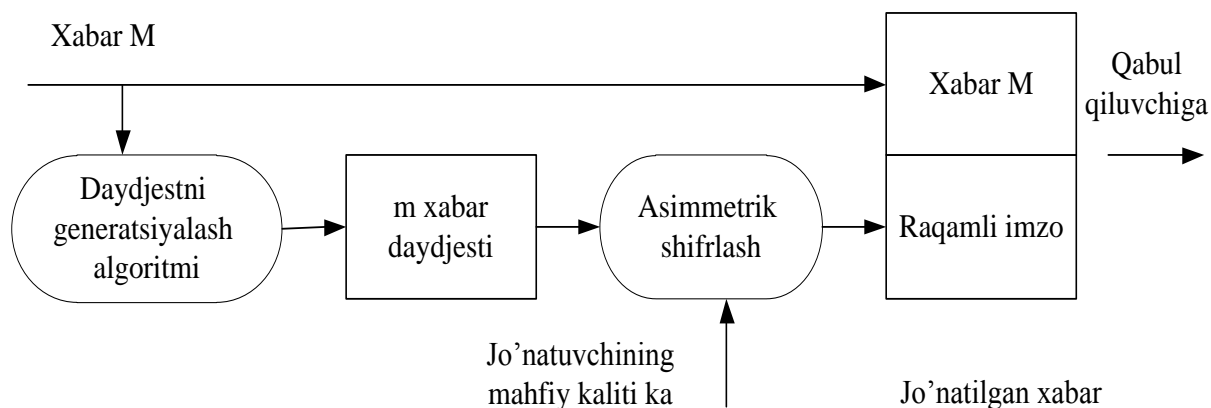
5.20-rasm. Elektron raqamli imzoni shakllantirish sxemasi.
