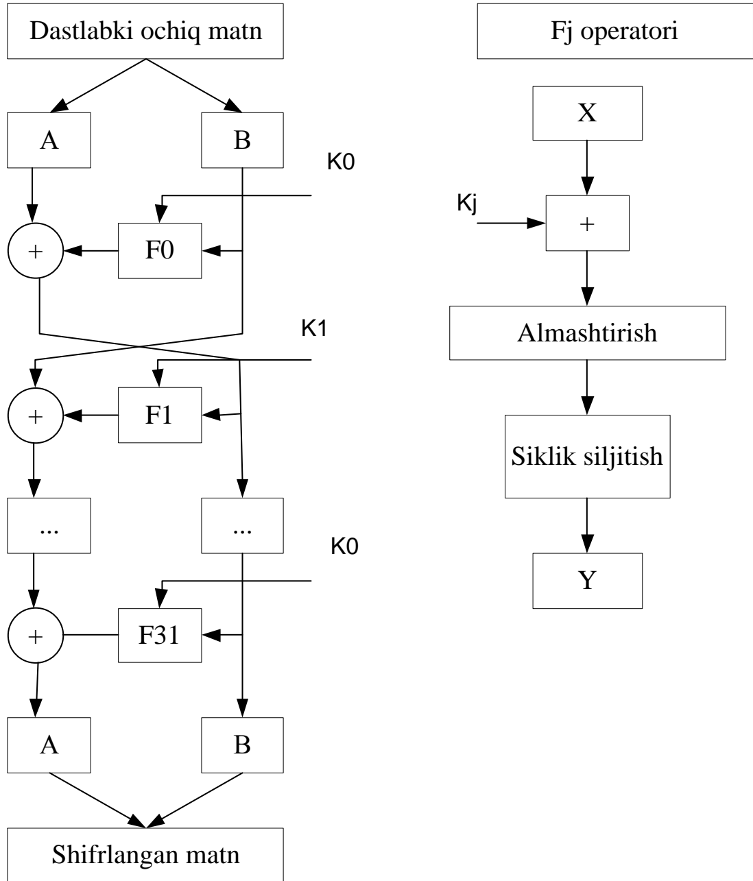
5.14-rasm. Oddiy almashtirish algoritmidagi shifrlash jarayonining blok-sxemasi.
