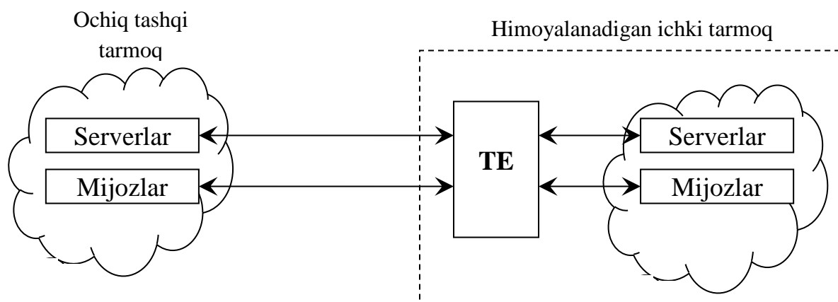
8.1-rasm. Tarmoqlararo ekranni ulash sxemasi
