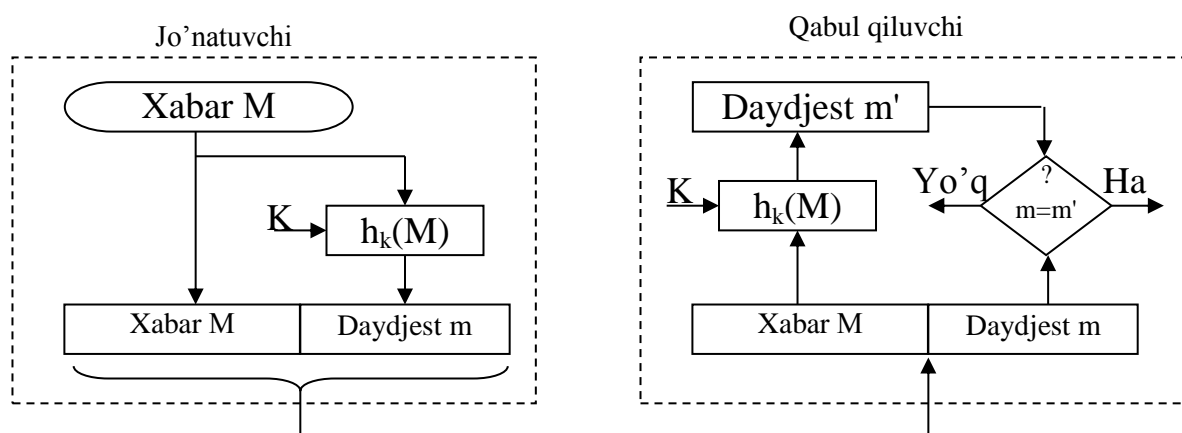
6.4–rasm. Ma'lumotlar yaxlitligini tekshirishda bir tomonlama xesh-funksiyaning ishlatilishi (I-variant).
