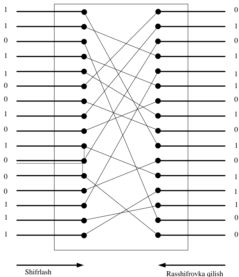
5.7-rasm. O'rin almashtirish sxemasi.
