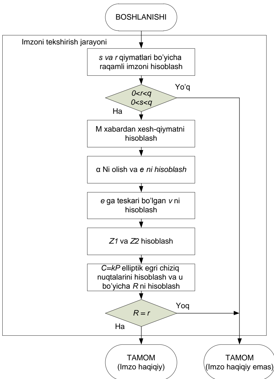
5.24-rasm. Elektron raqamli imzoni tekshirish jarayoni
