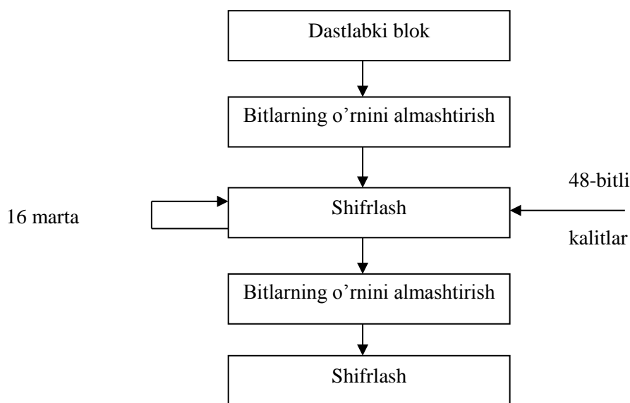
5.11- rasm. DES algoritmidagi shifrlash jarayonining blok-sxemasi
