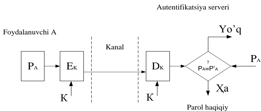
6.1-rasm. Paroldan foydalangan holda oddiy autentifikatsiyalash.
