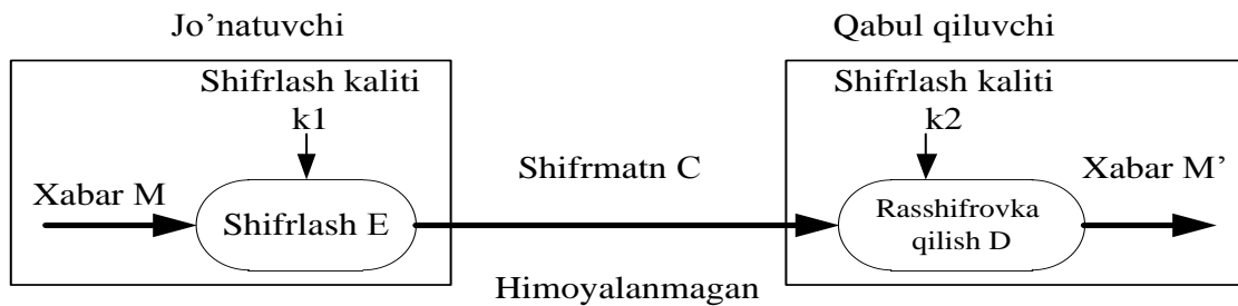
5.8-rasm. Shifrlash kriptotizimining umumlashtirilgan sxemasi.
