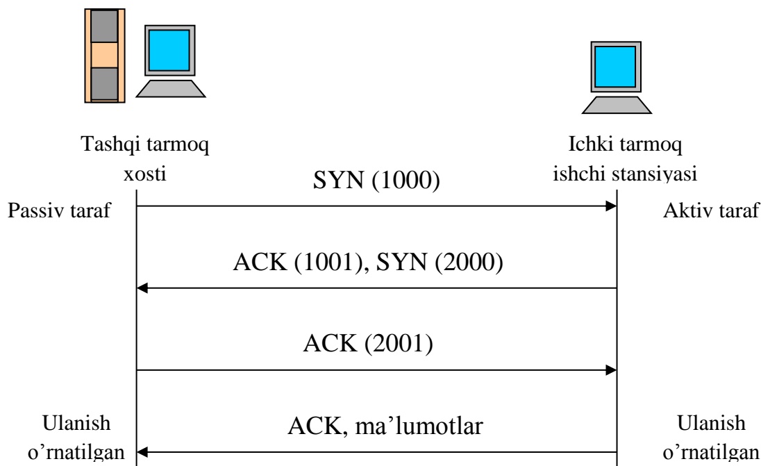
8.7-rasm. TCP protokoli bo'yicha aloqani kvitirlash sxemasi.
