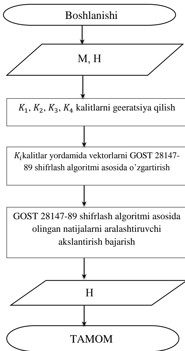
5.19-rasm. Xesh qiymatni hisoblash algoritmining blok-sxemasi
