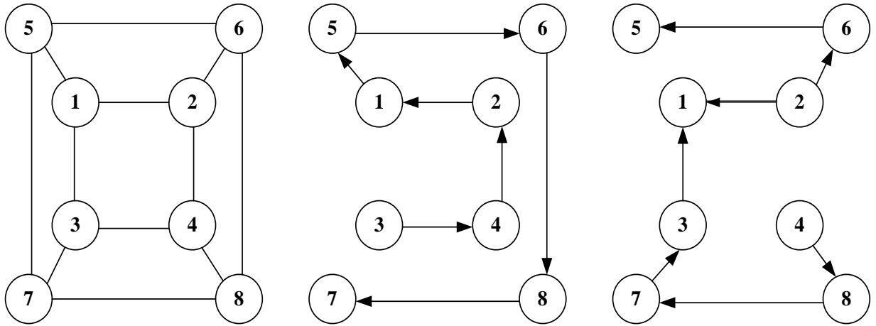
5.5-rasm. 8-elementli jadval va Gamilton marshrutlari variantlari.
