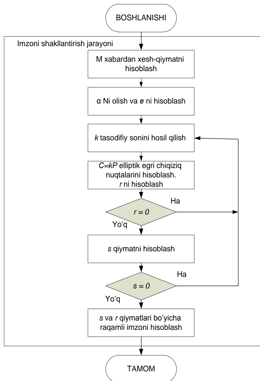
5.23-rasm. Elektron raqamli imzoni shakllantirish jarayoni.
