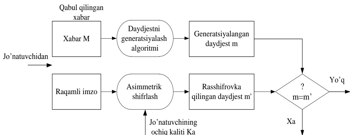
5.21-rasm. Elektron raqamli imzoni tekshirish sxemasi
