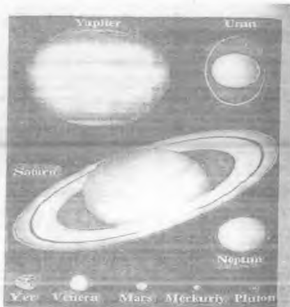
1-rasm. Quyosh tizimida planetalarning joylashishi.
