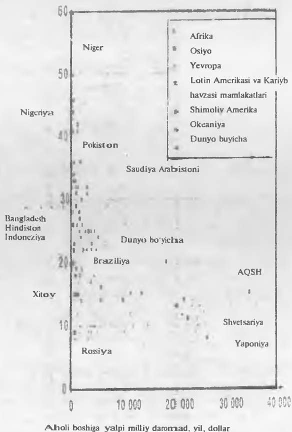
13-rasm. Tug'ilish va yalpi milliy daromad aholi boshiga (2001 yilda).
