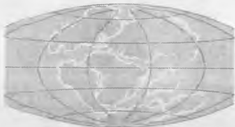
4-rasm Yura davrida Yer shari qit'alarining ko'rinishi.
