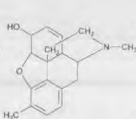
Кодеин
