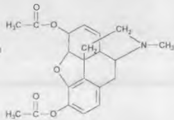
Героин
