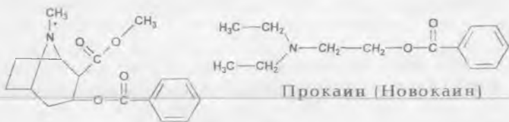
Кокаин
