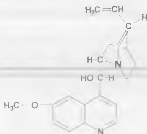
Хинин
