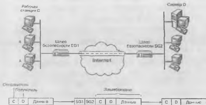
Рис. 3. Схема виртуального защищенного туннеля
