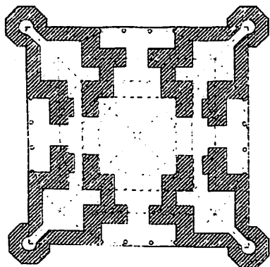
75-rasm. Bog'i Maydondagi «Chilstun» nomli ikki qavatli hashamatli saroy binosini qayta tiklash loyihasi (T.Mamatmusayev bo'yicha).
