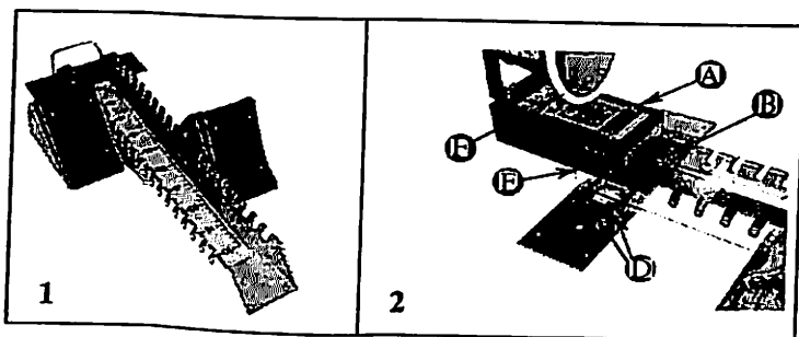
3-rasm. Start tirkaklari (1) va Falstartni qayd etuvchi moslama – Reactime (2). A – Sensor qutisi, B – Vint, D – Qotirgichlar, E – Montaj platasi, F – Ovoz kuchaytirgich.
