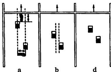
2-rasm. Start tirgaklarining joylashtirilishi: a – oddiy start uchun; b – uzoqlashtirilgan start uchun; d – yaqinlashtirilgan start uchun.
