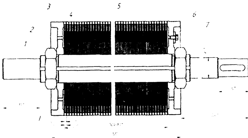
4-расм. Комбинацияланган арра-металл чўткали цилиндрнинг схемаси. 1 – вал; 2 – чап ёндаги сиқувчи гайка; 3 – чап диск; 4 – арралар орасига ўрнатиладиган металл чўткали дискдан тайёрланган қистирма; 5 – арра; 6 – ўнг диск; 7 – ўнг ёндаги сиқувчи гайка.
