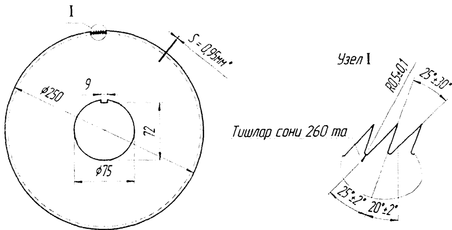
3-расм. Аррали дискнинг тиш профилининг ўлчамлари.
