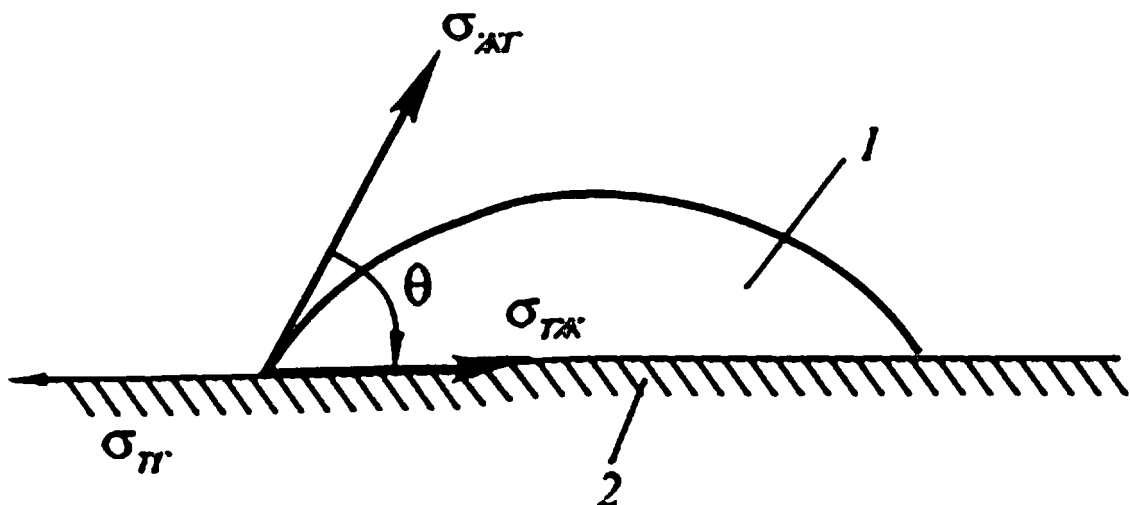
1-расм. Суюқлик томчисининг қаттиқ жисм сиртида ёйилиши: 1 – томчи; 2 – қаттиқ жисм.
