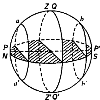
7-расм. Ер экваторидагилар учун юлдузлар ҳаракати расми
