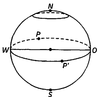
4-расм. Ер экватори ва қутб доираси
