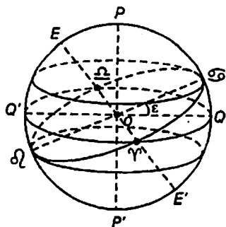
3-расм. Экваториал координатлар расми
