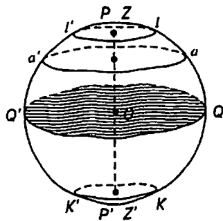
9-расм. Шимолий қутбдагилар учун юлдузлар ҳаракати расми
