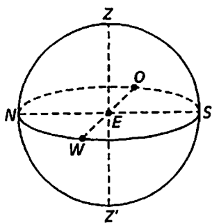
5-расм. Уфқ ва зенитга оид расм
