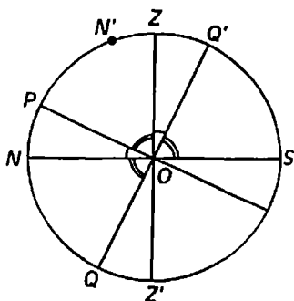
10-расм. Осмон доирасининг меридианига текислик проекцияси
