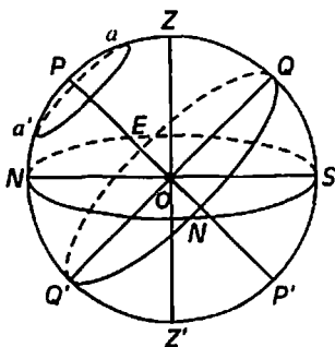
6-расм. Экваториал ва горизонтал координатлар расми
