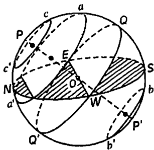
8-расм. Шимолий кенгликдагилар учун Ер ҳаракати расми
