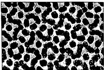
9.1-rasm. Avtotip ko'p rangli bosma (nusxa mikrofotoqrafiyalari), rastr nuqtalari orasidagi masofa qariyb 167 mkm:
