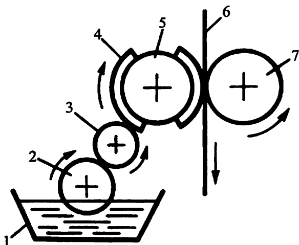
3.14-rasm. Fleksografik uskunasi bosma apparatining prinsipial tizmasi:
