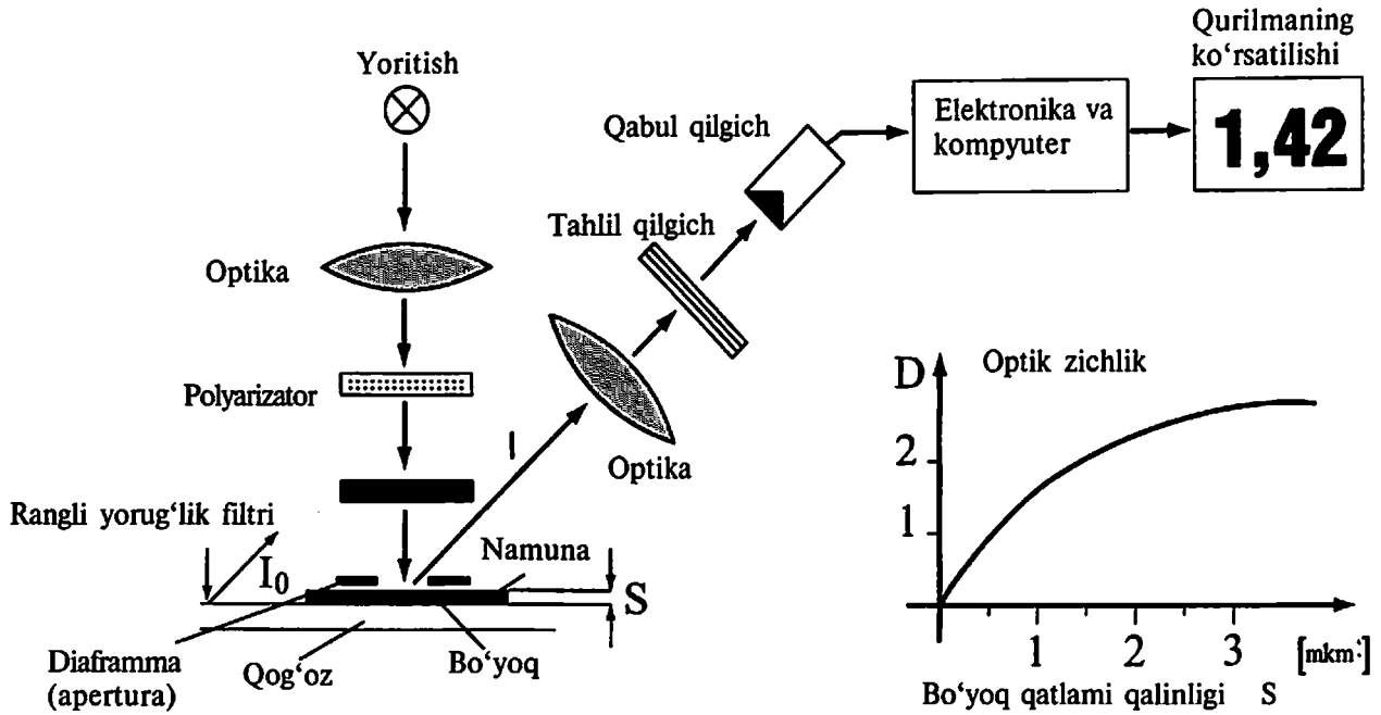
12.3-rasm. Optik zichlikni o'lchash uchun densitometrning tuzilish prinsipi
