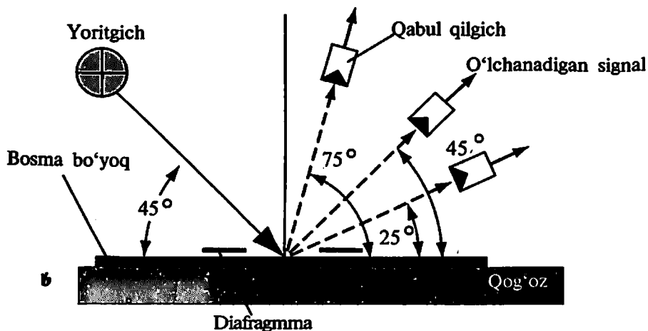
12.17-rasm. Yaltiroqlikni o'lchash prinsipi:
