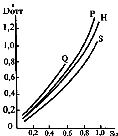
18.2-rasm. Turli bo'yoqlarda bosilgan shkalali ofset nusxalarning gradatsion xususiyatlari:
