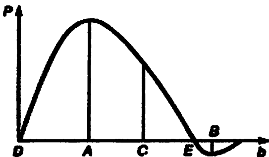
3.5-rasm. Bo‘yoq apparati tekislovchi guruhning silindri va valigi kontakti maydonida bosimning taqsimlanish shakli
