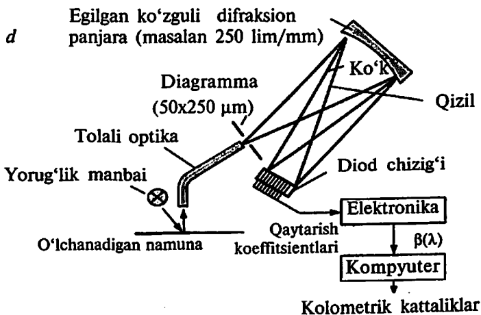
12.10-rasm. Spektral yorug'lik qaytarishni o'lchashning spektrofotometrik prinsiplari:
