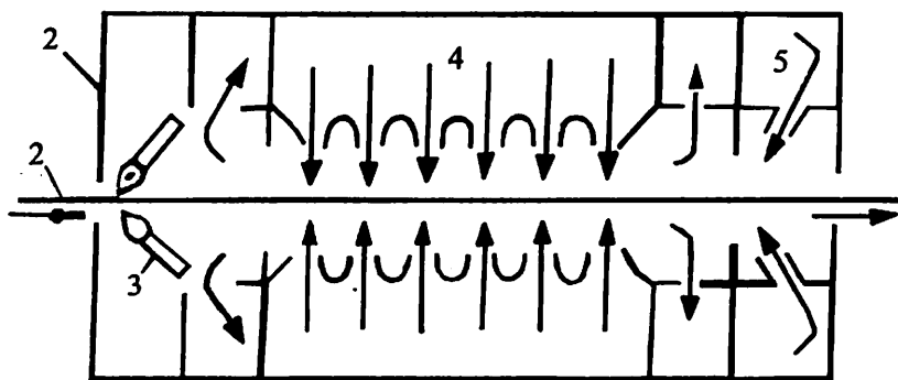
6.3-rasm. Otepka turidagi kombinirlangan uskuna
