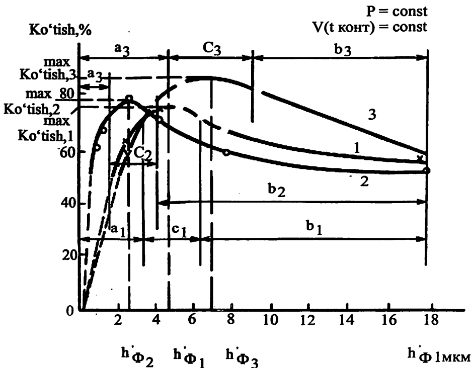
5.1-rasm. Bosma kontakti vaqtida qolip va bosiluvchi material orasidagi bo'yoqning ajralishi
