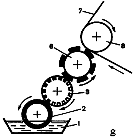
3.15-rasm. Fleksografik bosma uskunalari bo'yoq apparatining namunaviy tizmalari:
