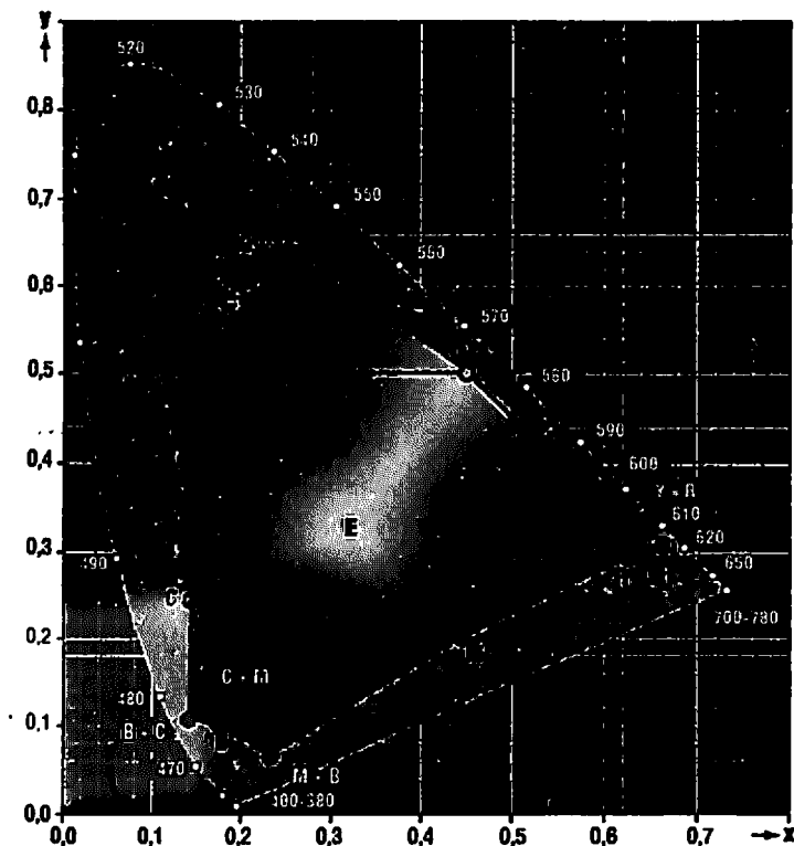
9.9-rasm. CIE ranglilik diagrammasida HiFi-bosmaning rang qamrovi ( x, y, z ) (tizim: havorang, qirmizi, sariq + qizil, yashil va ko'k bo'yoqlar odatdagi ko'p rangli bosmadagi qamrov bilan qiyoslaganda).
