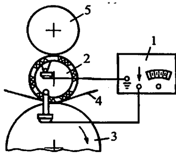
17.1-rasm. Chuqur bosma uskunasiidagi EP 20 qurilmasining joylashish tizmasi
