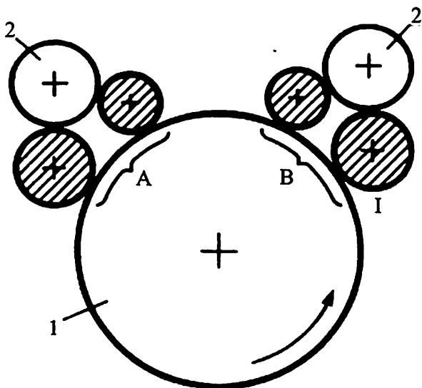
3.11-rasm. Rotatsion uskunasi bo‘yoq apparatining to‘rt valikdan tashkil topgan surtish guruhi
