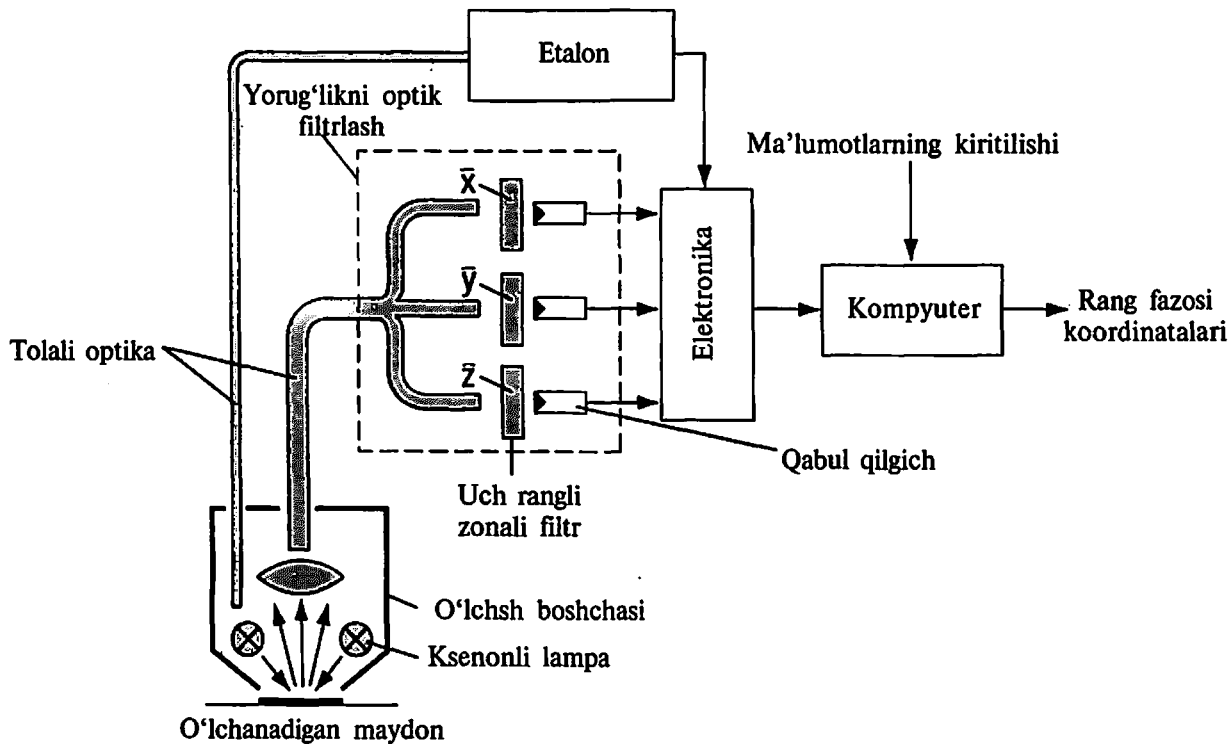
12.9-rasm. Fotoelektrik kolorimetr; filtrlar yordamida rangni uchta zonali tarkibiy qismlarga optik ajratish
