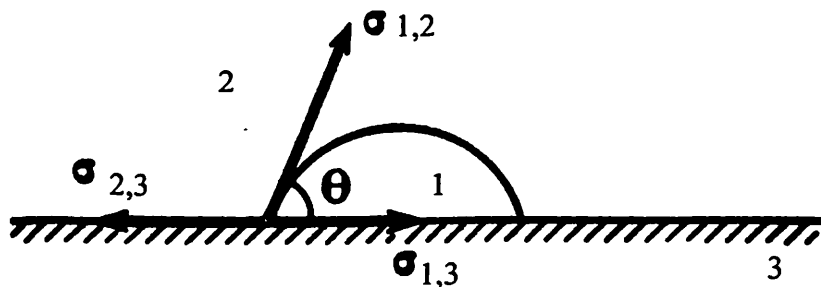
2.1-rasm. Namlash burchagi va yuza tortilishi o'rtasidagi bog'liqlik
