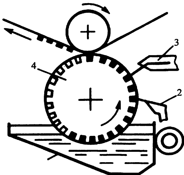
3.13-rasm. Qiya rakelni o'rnatish tizmasi:
