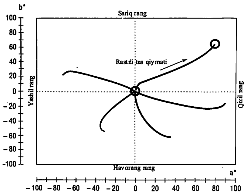
9.6-rasm. CIE Lab tizimida bo'yoqlar ustma-ust tushirilgan vaqtda, CMY asosiy ranglari uchun va ulardan olinadigan qo'shimcha RGB ranglari uchun rastr nuqtasining nisbiy o'lchami (0 dan 100% gacha) o'zgargandagi gradatsion egri chiziq (Thermotransfer Proof System «Rainbow», Imation rang namunasini termoo'tkazish tizimi)
