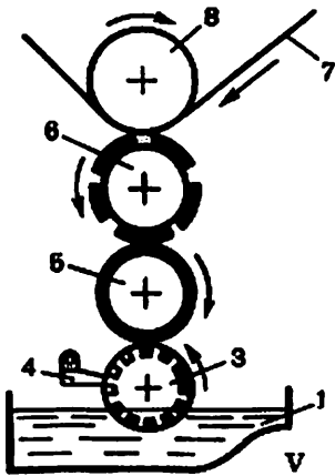
3.15-rasm. Fleksografik bosma uskunalari bo'yoq apparatining namunaviy tizmalari:
