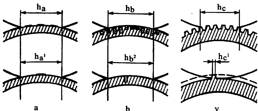
4.2-rasm. Bosishning turli usullarida qoliplarning turli koeffitsiyentda to'ldirilgandagi yuz kontaktining kengligi
