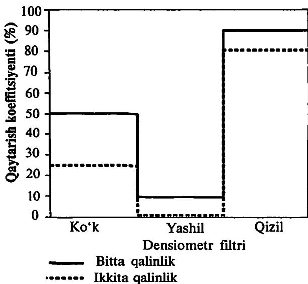
14.9-rasm. Bo'yoq qatlami qalinligining o'zgarishi ko'k, yashil va qizil yorug'likning tegishli qaytarish koeffitsiyentlariga noproporsional ta'sir ko'rsatadi
