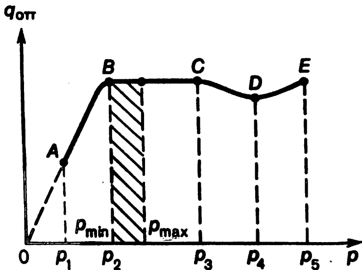
4.3-rasm. Qolipdan qog'ozga o'tayotgan bo'yoq miqdorining bosimga bog'liqligi
