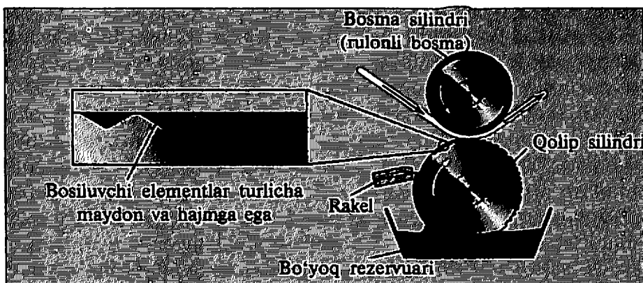
13.6-rasm. Chuqur bosma (tamoyili)
