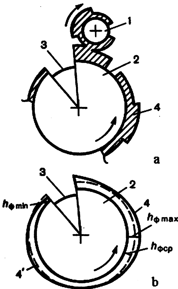
3.10-rasm. Bir valik bilan qolipga bo'yoq surtishda qolip silindrida bosilmaydigan maydonlarning mavjudligi munosabati bilan surtuvchi valik va qolip silindrida bo'yoq qatlamining taqsimlanishi
