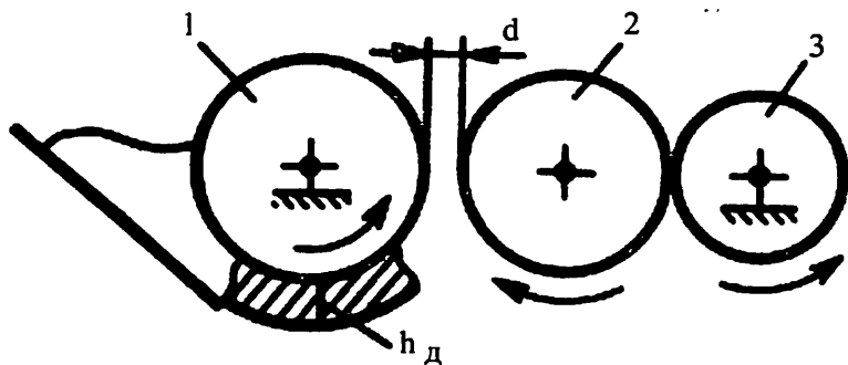
3.1-rasm. Plyonkali (tirqishli) bo‘yoq apparatining bo‘yoq uzatish tizmasi
