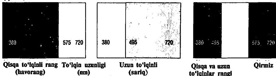
9.3-rasm. «Ideal» bo'yoqlar uchun spektral taqsimlanishlar (nisbiy yorug'lik qaytishi)
