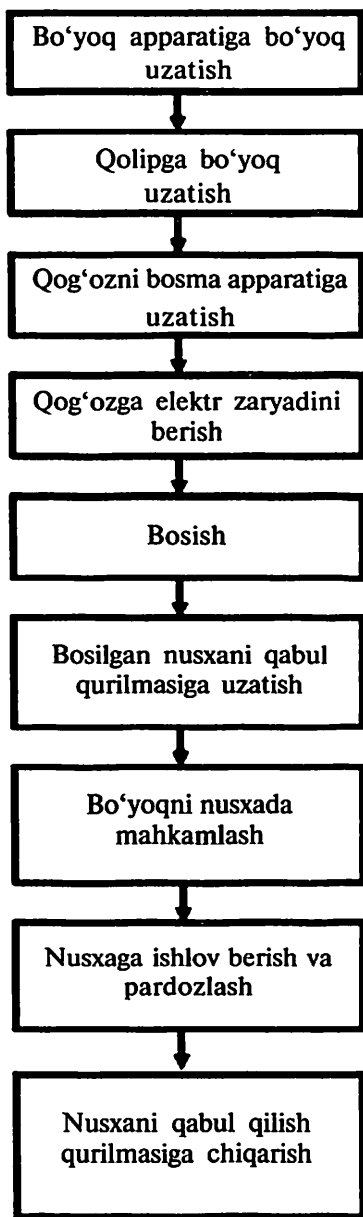
7.3-rasm. Yuqori bosma jarayoni texnologiyasi
