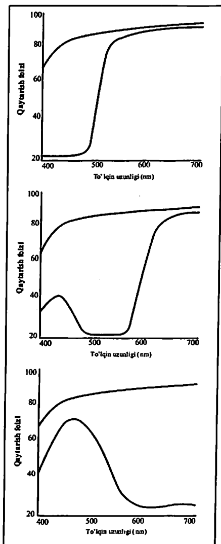
14.6-rasm. Real triada bo'yoqlarining spektrofotometrik egri chiziqlari, ular real materialda bosilganda qanday ko'rinishda bo'lishi ko'rsatilgan: sariq (tepada), qirmizi (o'rtada) va havorang (pastda)
