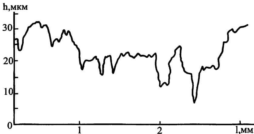
4.1-rasm. Yuqori bosma uchun mo'ljallangan №1 qog'oz yuzasining ko'ndalang kesimi (profilogrammasi)
