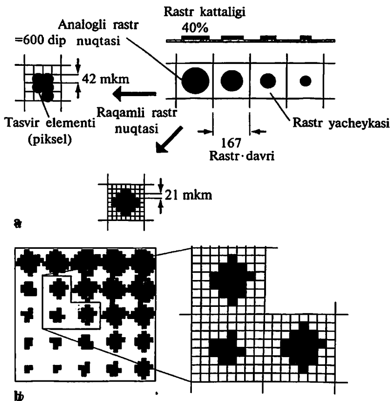
10.12-rasm. «Raqamli» rastr nuqtalari strukturasi:
