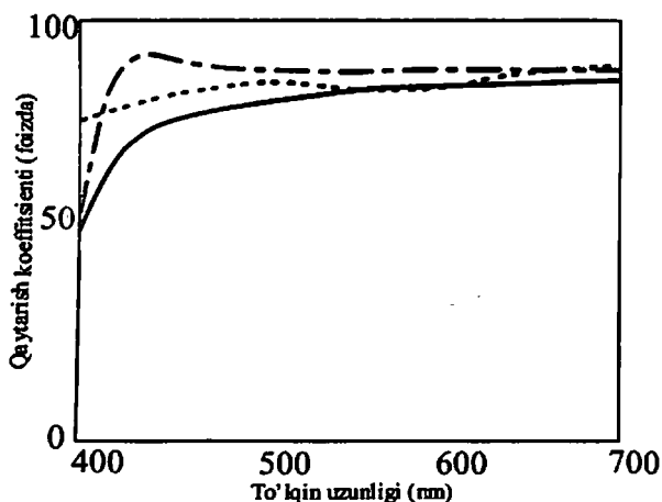
14.1-rasm. GATF tadqiqotlari doirasida tanlangan qog‘oz namunalarining spektrofotometrik egri chiziqlari
