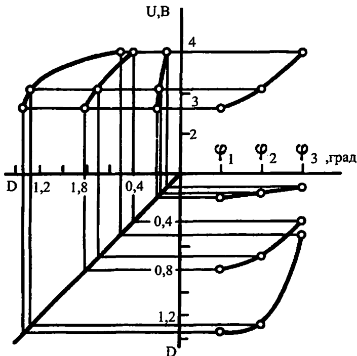
16.3-rasm. Nusxadalar optik zichligi D ning namlovchi eritmaning miqdoriga bog‘liqligi S_f^{nis} = 100\% ). \varphi — duktor vali aylanish burchagining o‘zgarishi, U, B — registrlovchi asbob ko‘rsatkichi
