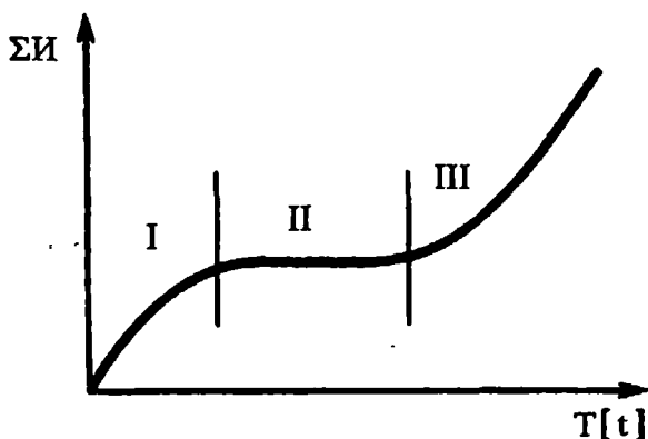
8.2-rasm. Bosma qoliqlarning bosish jarayonida yemirilishga chidamlilik ko'rsatkichlarining o'zgarish kinetikasi
