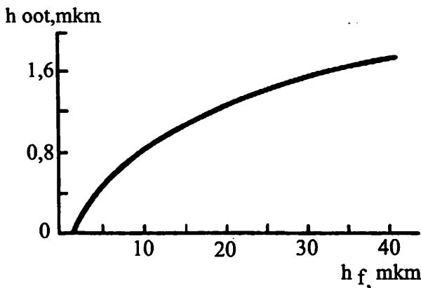
5.3-rasm. Varaqli chuqur bosmada bo'yoq o'tishining egri chizig'i
