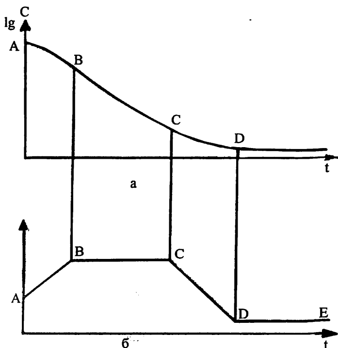
6.1-rasm. Bo‘yoqni mustahkamlashda asosiy fizik bosqichlar:
