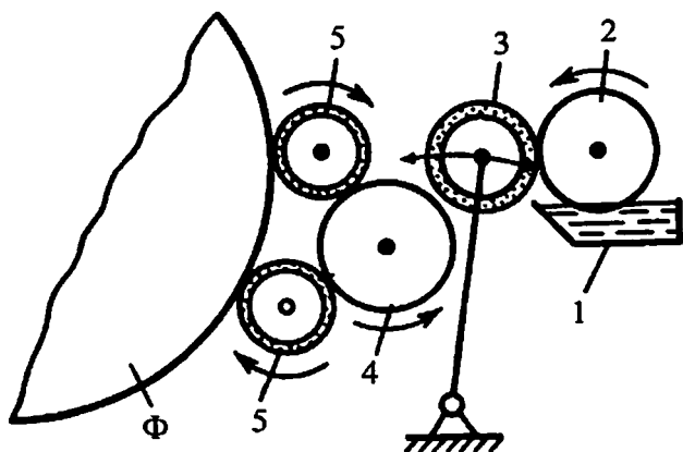
16.4-rasm. Varaqli ofset uskunasi namlash apparati
