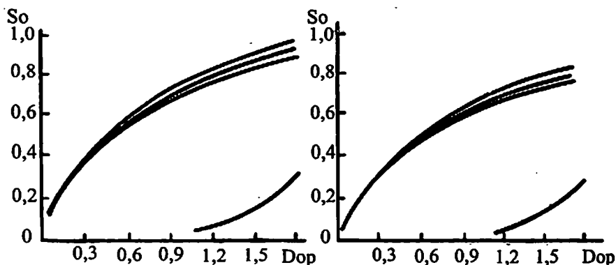
18.1-rasm. Turli bo'yoqlar uchun ranglarga ajratilgan qoliplarning gradatsion xususiyati:
