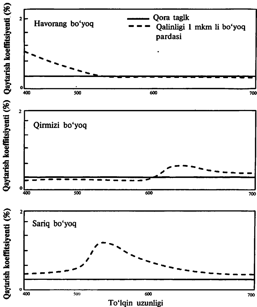
14.8-rasm. Bo'yoqlarning shaffoligini o'lash sohasidagi tadqiqotlar doirasida Leneta 105C qora tagligida bosilgan sariq, qirmizi va havorang SWOP bo'yoqlari namunalari uchun spektrofotometrik egri chiziqlar
