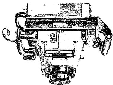
2.7.2.-rasm. WILD C2 firmasi tomonidan ishlab chiqarilgan aerofotokamera (1927-yil)
