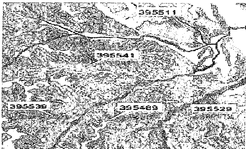
6.3.2-rasm. Hidrografik tarmoqlarning tuproq xaritasiga tushirilishi
