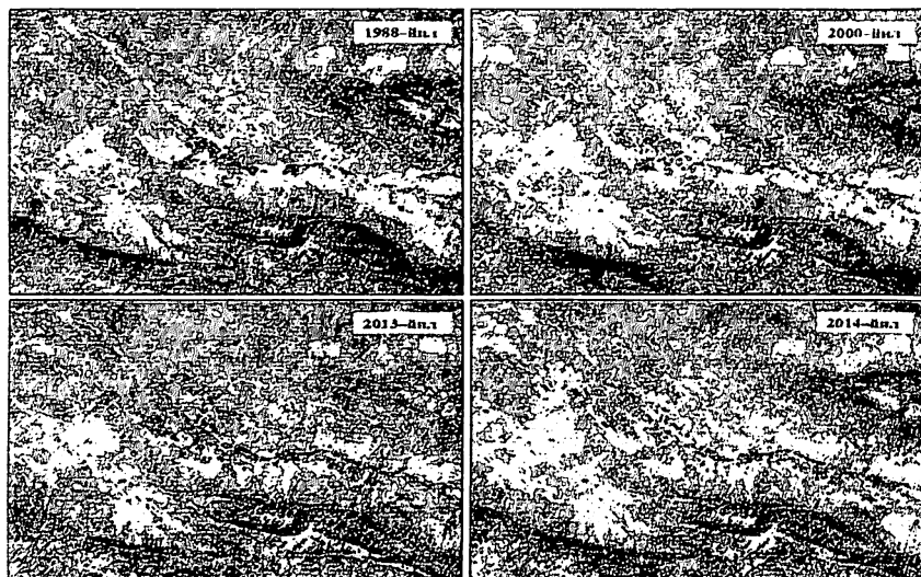
11.5.3-rasm. Nurota tumani xududida yillar bo'yicha sho'rlangan tuproqlarning tarqalishi
