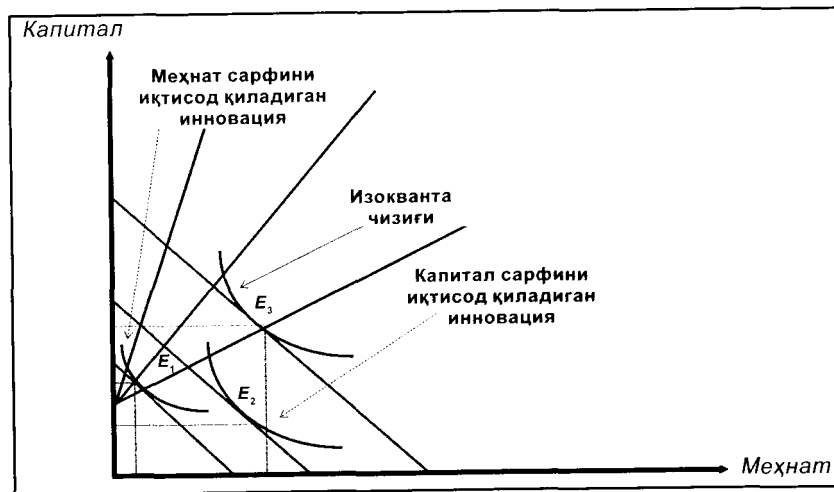
2.2.1-расм. Омиллар сарфини иқтисод қилувчи инновацион жараёнлар.
