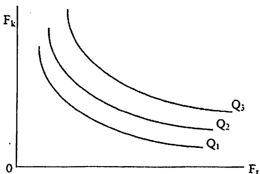
Изокванталар харитаси
