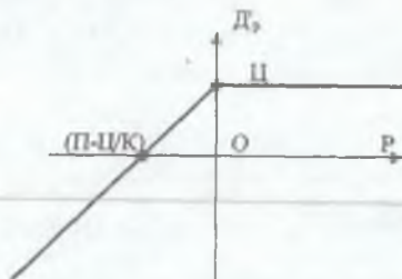
4.7.4-rasm. Put opsiyon sotuvchisi daromadi funksiyasi
