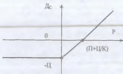
4.7.1-rasm. Koll opsiyon haridorining daromad funksiyasi
