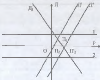
4.7.5-rasm. F'yucherslar operatsiyasidagi daromadlar funktsiyasi
