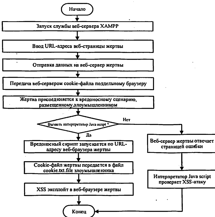
Рисунок 3. Блок-схема алгоритма обнаружения XSS-атаки на сервере LocalHost
