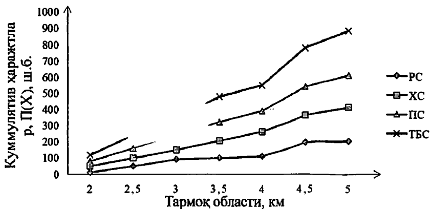
3-расм. Куммулятив харажатларнинг тармоқ области ўлчамига боғлиқлиги
