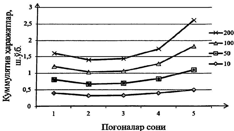
4-расм. Куммулятив ҳаражатларнинг поғоналар сони билан боғлиқлиги.
