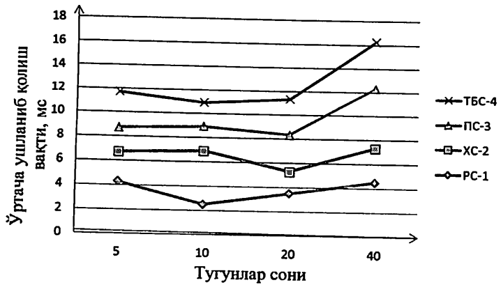
5-расм. Тармоқ тугунлари сонининг маълумотларнинг ўртача ушланиб қолиш вақтига боғлиқлик графиги.
