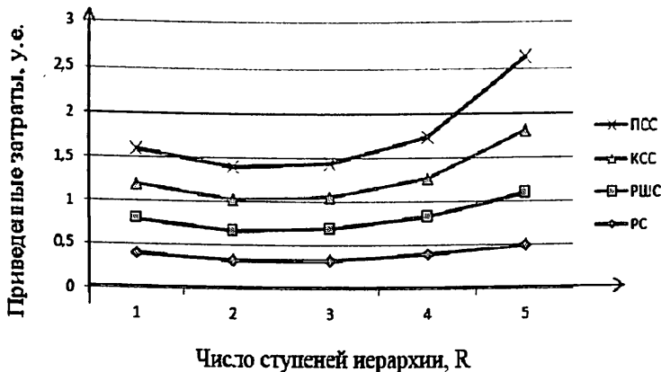
Рис.8. График зависимости общесетевых кумулятивных затрат от числа ступеней.
