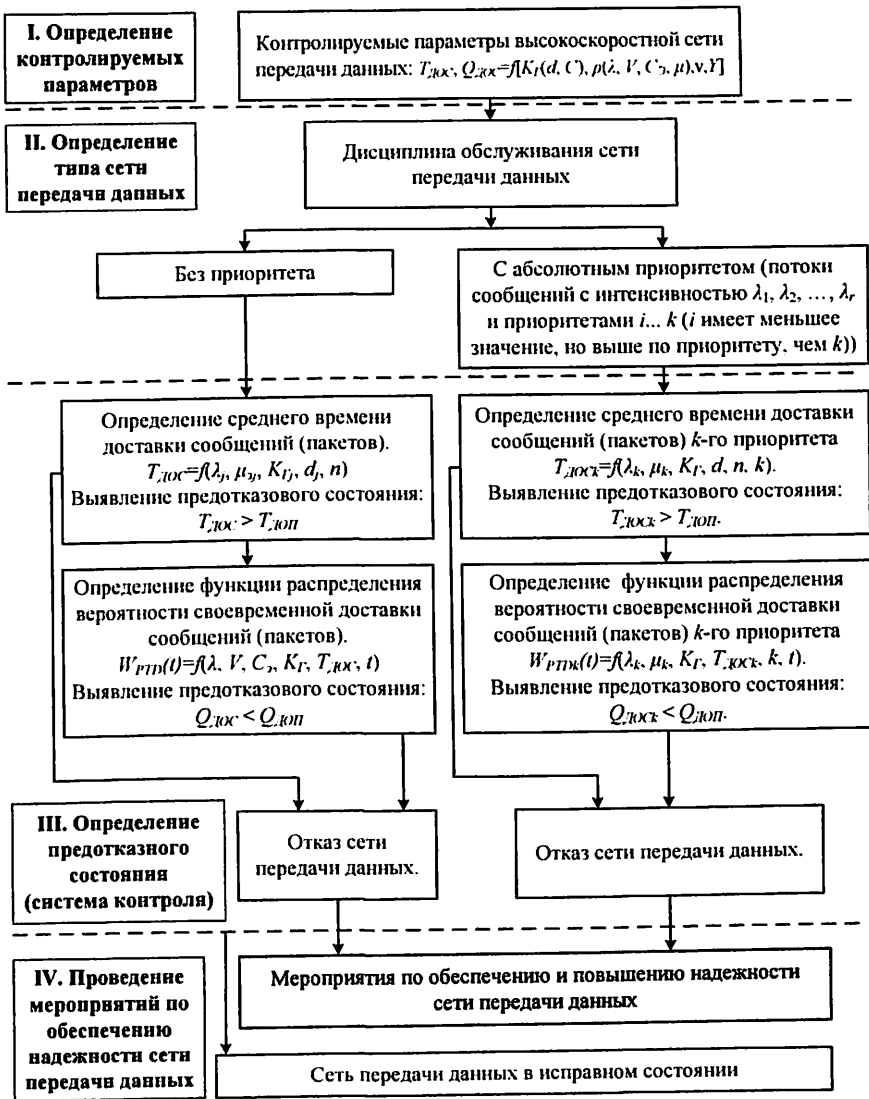
Рис. 1. Блок-схема реализации метода определения предотказного состояния высокоскоростной сети передачи данных
