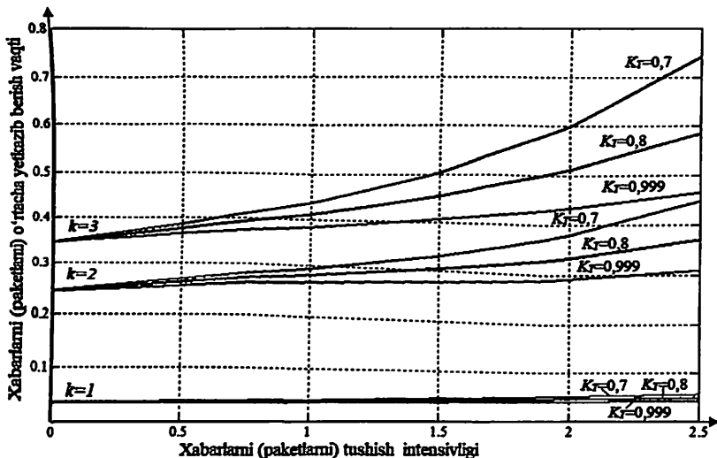
5-rasm. Turli ( K_T=0,7; 0,8; 0,999 ) tayyorik koeffitsiyentlarida xabarlarini (paketlarni) tushish intensivligiga bog'liq ravishda k -chi ( k=1; 2; 3 ) prioritetli xabarlarini (paketlarni) o'rtacha yetkazib berish vaqtining tadqiqi
