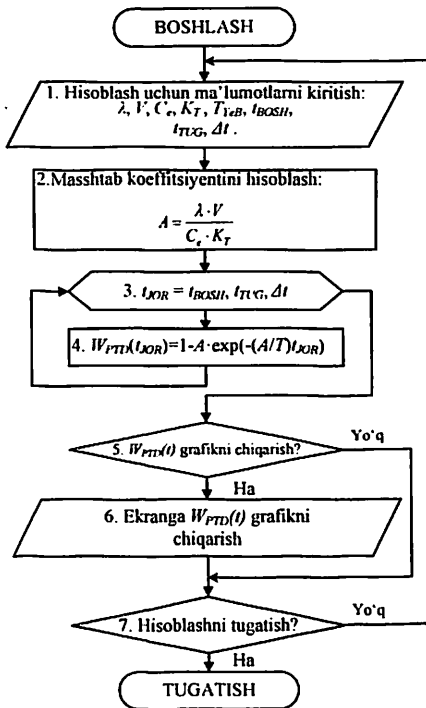
2-rasm. Xabarlarini (paketslarni) o'z vaqtida yetkazib berish ehtimoli taqsimoti funksiyasini hisoblash algoritmi
