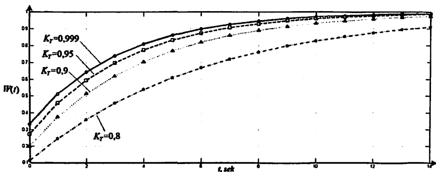
6-rasm. Turli ( K_T=0,8; 0,9; 0,95; 0,999 ) tayyorik koeffitsiyentlari qiymatlarida k=1 prioritetli xabarlarini (paketlarni) o'z vaqtida yetkazib berish ehtimoli taqsimoti funksiyasining tadqiqi
