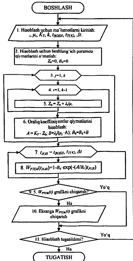
4-rasm. k -chi prioritetli xabarlarni (paketlarni) o'z vaqtida yetkazib berish ehtimoli taqsimoti funksiyasini hisoblash algoritmi
