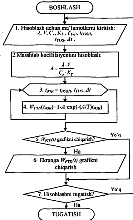
2-rasm. Xabarlarni (pakatlarni) o'z vaqtida yetkazib berish ehtimoli taqsimoti funksiyasini hisoblash algoritmi
