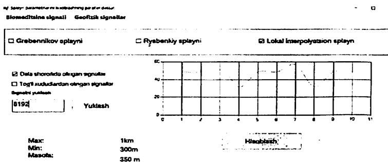
Рис. 6. Окно программы цифровой обработки аэромагнитного сигнала
