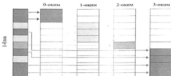
5-расм. Локал интерполяцион кубик сплайнлар параметрларини параллел ҳисоблаш жараёнларини қўриниши
