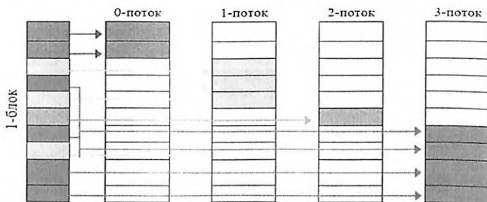
Рис. 5. Процессы параллельного вычисления параметров локальных интерполяционных кубических сплайнов
