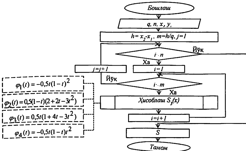
2-расм. Локал интерполяцион кубик сплайн модели асосида СРИБ алгоритми
