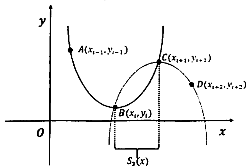
Рис. 1. Вид интервала построения локального кубического сплайна S_3(x)
