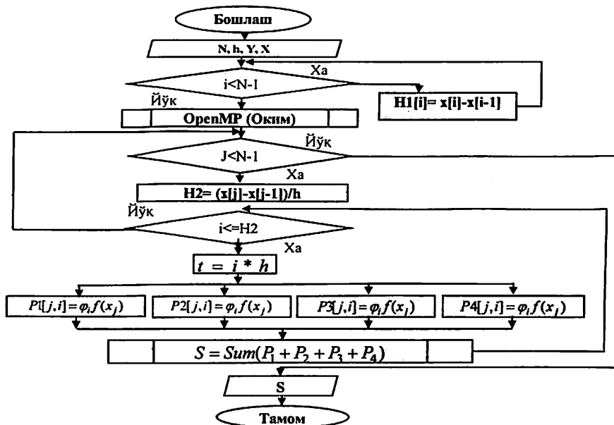
3- расм. Тенгмас ораликларда олинган сигналларни рақамли ишлаш жараёнларини кубик сплайнлар ёрдамида параллел ҳисоблаш алгоритми
