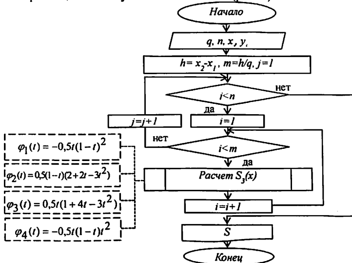
Рис. 2. Алгоритм СРИБ на основе модели локального интерполяционного кубического сплайна
