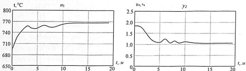
Рис. 2. Реализации управляющего воздействия и выходной переменной рассматриваемого процесса по каналу u_1 \rightarrow y_1
