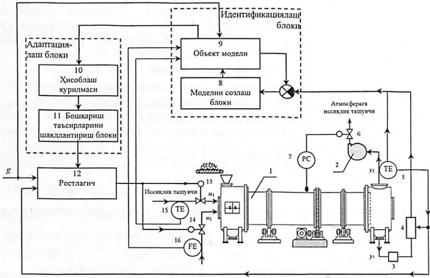
3-расм. Чиқиш ўзгарувчилари бўйича калий хлоридни қуритиш жараёнини адаптив бошқариш системасининг структураси.
