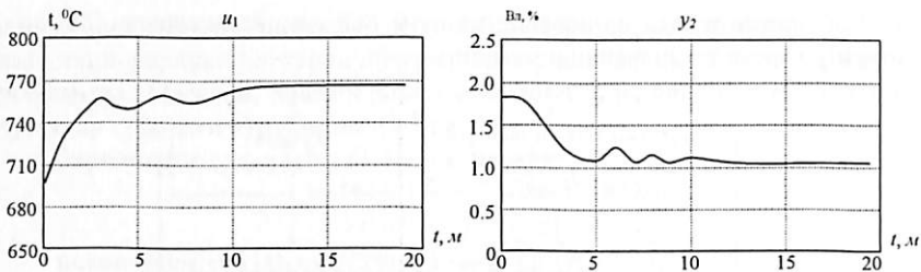
2-расм. u_1 \rightarrow y_1 канал бўйича кўриб чиқилаётган жараённинг бошқариш таъсирлари ва чиқиш ўзгарувчиларини амалга оширилиши.
