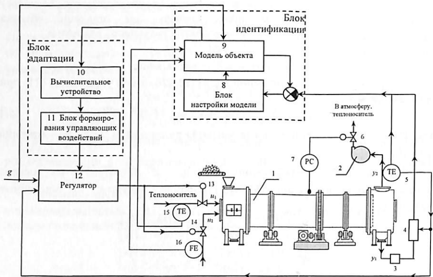
Рис.3. Структура адаптивной системы управления процессом сушки калия хлорида по выходным переменным
