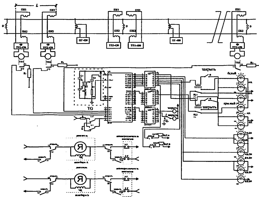
Рис 12. Микропроцессорная переездная сигнализация с автошлагбаумами.
