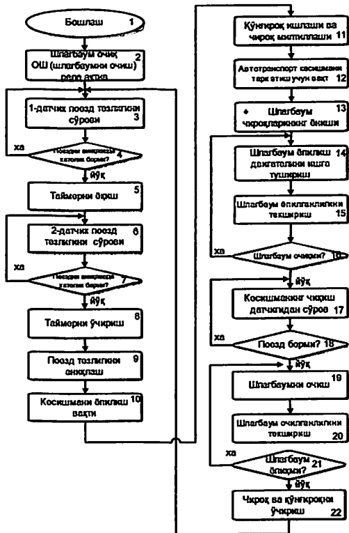
13-расм. Кесишма сигнализацияси қурилмалари ва автошлагбаумларни бошқариш ва назорат қилиш алгоритмининг блок-схемаси.
