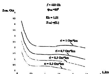
10-расм. f = 480 Гц ва \phi_{\text{вхн}} = 80^\circ сигналли частоталарида занжир узунлигининг рельс изининг синиш сезгирлигини таъминлаш шarti билан назорат датчиги кириш қаршилигининг боғлиқлик графикалари.
