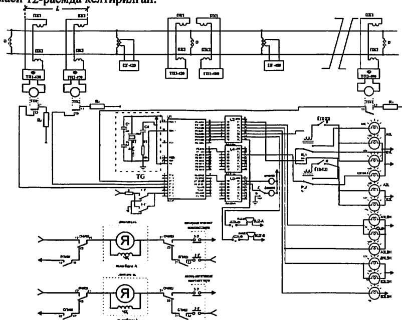
12-расм. Автошлагбаум билан микропроцессорли кесишма сигнализацияси.
