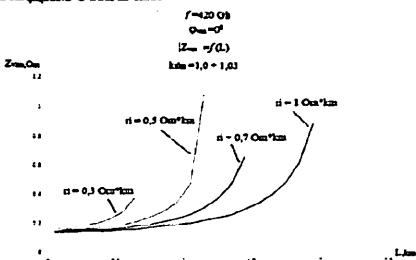
9-расм. \phi_{\text{вхн}} = 0^\circ ва f = 420 Гц сигнал частотасида занжир узунлигига шунг сезгирлигини таъминлаш шarti билан бошқарув датчиги кириш қаршилиги боғлиқлик графикалари
