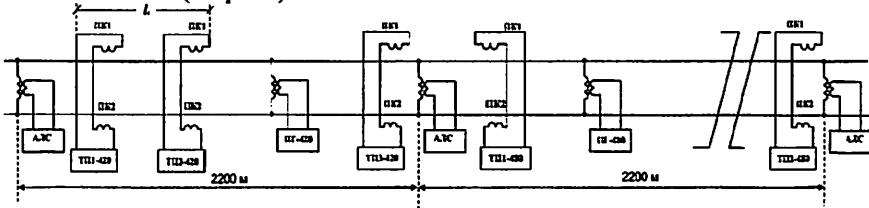
11-расм. Токли қабул қилгич билан назорат датчигининг схемаси
