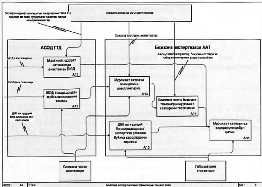
4-расм. БЭ ААТнинг фаолият кўрсатиш алгоритми
