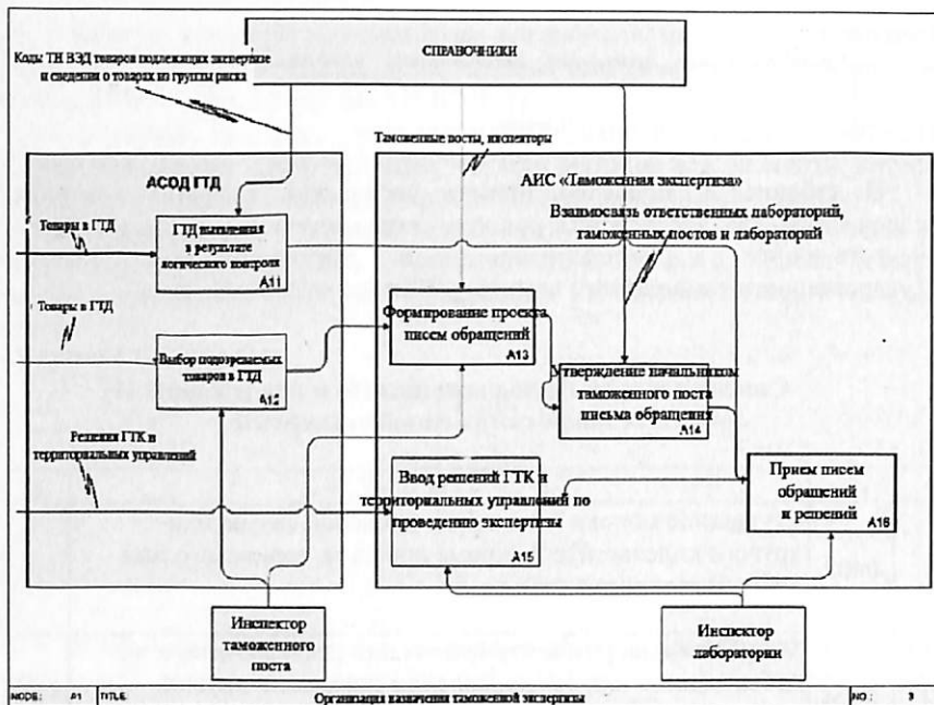
Рис.4. Алгоритм функционирования АИС ТЭ.
