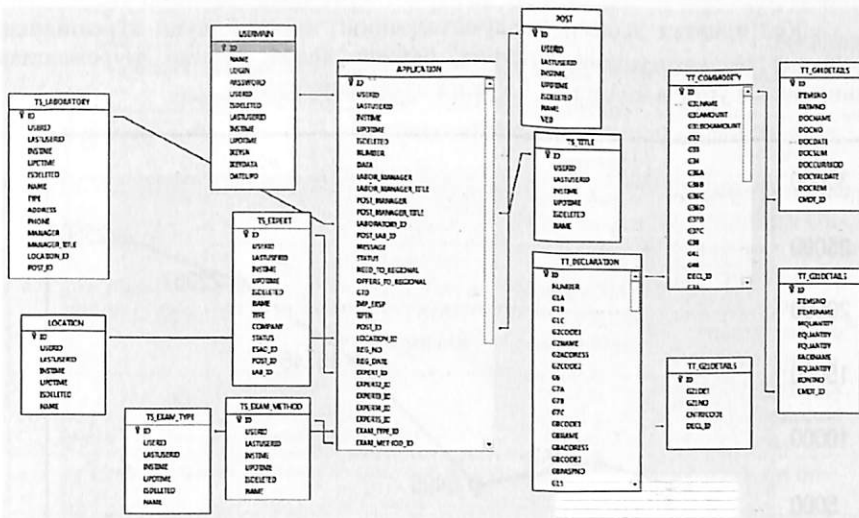
5-расм. БЭ ААТ нинг маълумотлар базаси таркиби
