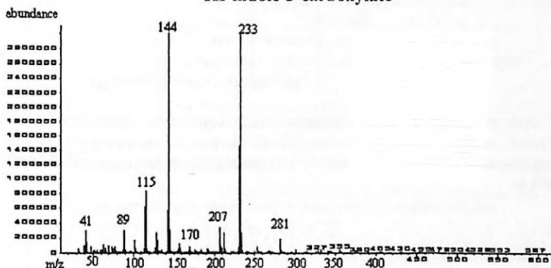
Рис. 2.4.4. Масс спектры NM-2201 Naphthalen-1-yl-1-(5-fluoropentyl)-1H-indole-3-carboxylate
