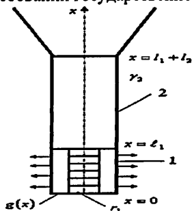
Рисунок 6. Физическая модель термометра сопротивления относительно температуры контролируемой среды
