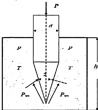
3-расм. Бирламчи ўлчаш ўзгарткичи ва материал ўртасидаги кучлар схемаси
