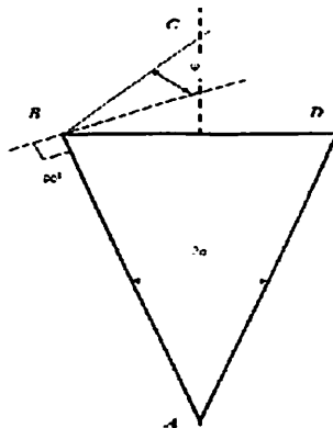
φ - ишқаланиш бурчаги; А, В, D – конус учлари; α – конус учи бурчаги.
