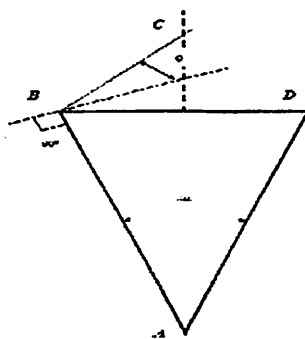
Рисунок 4. Геометрические размеры конусной части преобразователя \phi - угол трения; A, B, D - кончики конуса; \alpha - угол между образующими конуса
