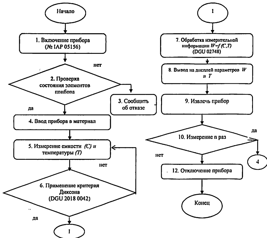
Рисунок 8. Алгоритм определения контролируемой влажности хлопко-сырца
