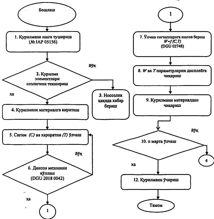
8-расм. Пахта назорат қилинаётган намлигини аниқлаш алгоритми
