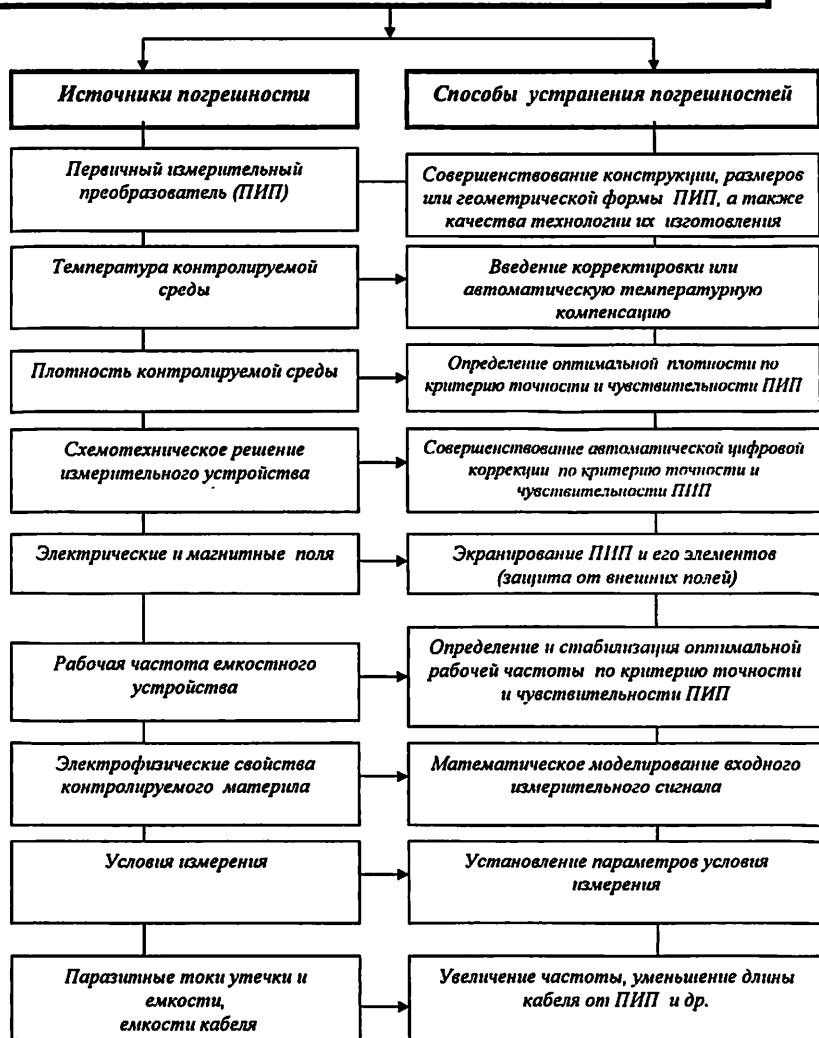
Рисунок 5. Классификация источников погрешностей и способы их устранения при контроле влажности материалов емкостным методом
