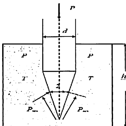
Рисунок 3. Схема сил между первичным измерительным преобразователем и материалом
