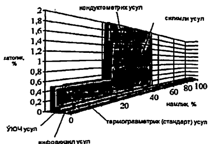
2-расм. Намликни назорат қилиш усуллари хатоликларининг солиштирма қийматлари
