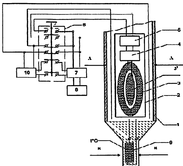
7-расм. Пахта намлиги ва ҳароратини назорат қилиш қурилмаси
