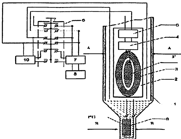
Рисунок 7. Устройство для контроля влажности и температуры хлопка-сырца
