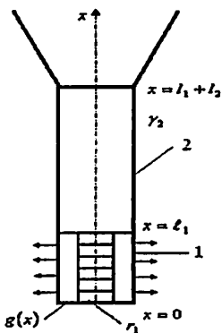
6-расм. Қаршилик термометрининг назорат қилинаётган муҳитнинг ҳарорат нисбатан физик модели:
