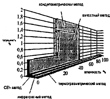
Рисунок 2. Сравнительные значения погрешностей методов контроля влажности
