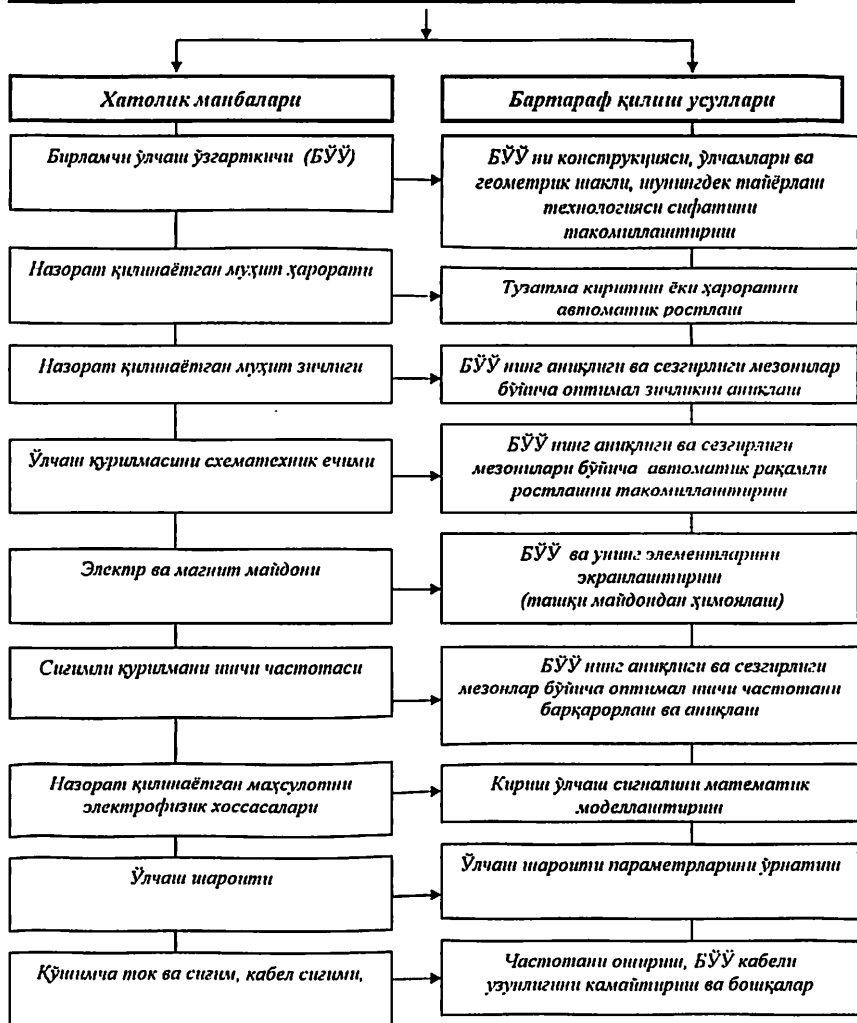
5-расм. Сигимли усулда материаллар намлигини назорат қилишда хатолик манбалари таснифи ва уларни бартараф қилиш усуллари
