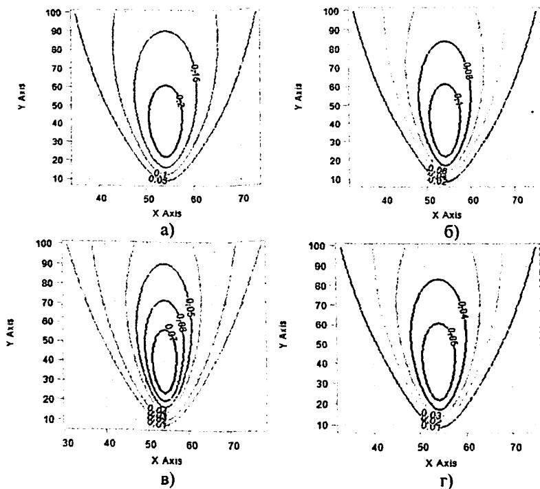
Рис. 3. Визуализация процесса переноса и диффузии оксида серы (IV) при разных скоростях ветра (ПДК=0,05 мг/м³).
