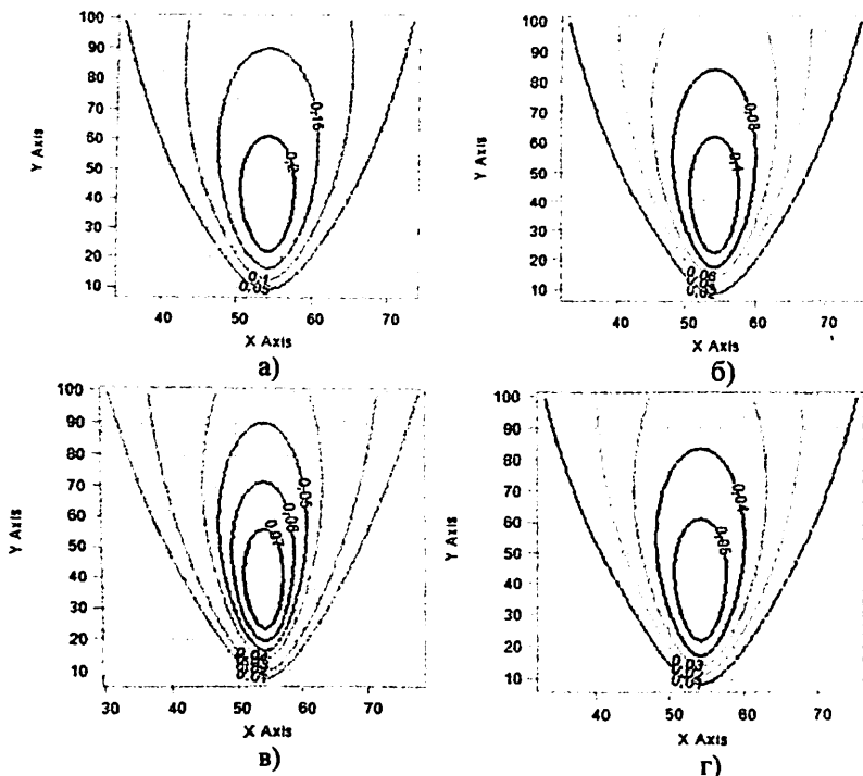
3 – расм. Олтингурт оксиди (IV) зарарли моддасининг атмосферада қўчиши ва диффузияси жараёнини шамолнинг турли тезликларида визуализация қилиш ( PЭМҚ=0,05\text{ мг/м}^3 ).
