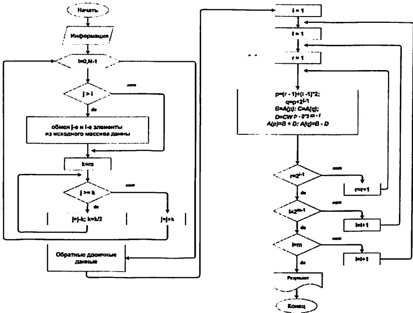
Рис. 4. Блок-схема алгоритма параллельной обработки массивов данных
