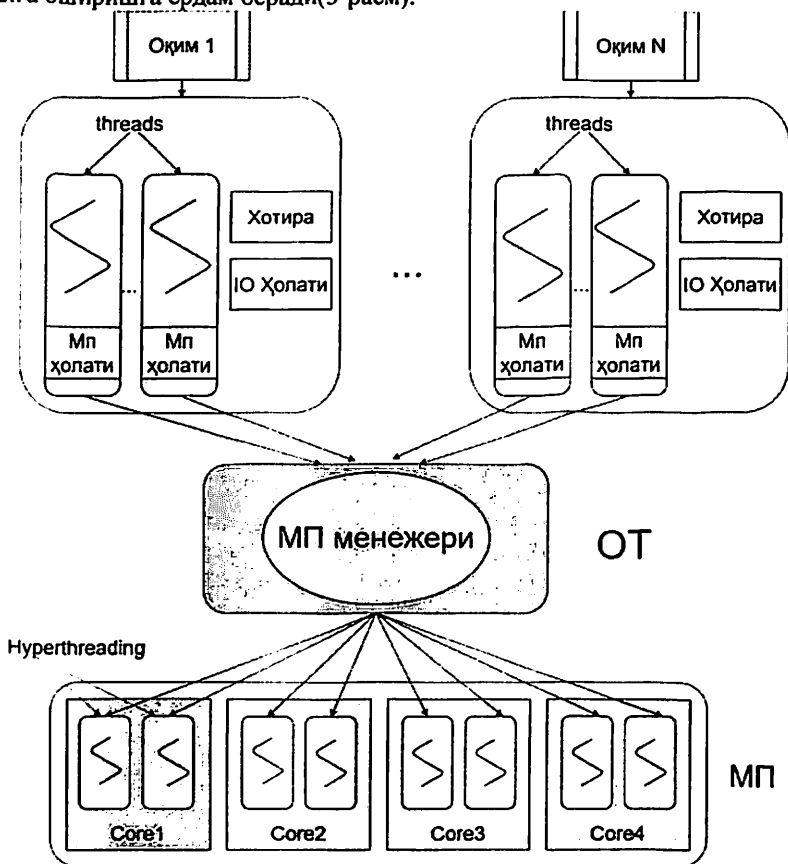
3-расм. Hyper-Threading технологиясидан фойдаланиб процессордаги оқимларини тавсифлаш.
