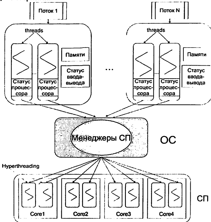
Рис. 3. Характеристика потоков в процессоре с использованием технологии Hyper-Threading.
